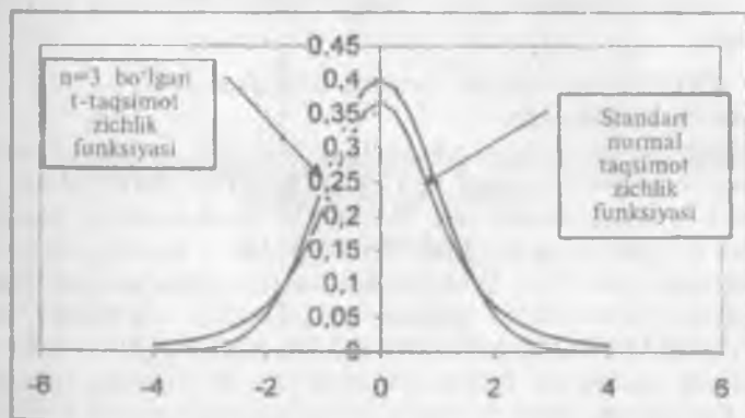
6-rasm. t - yoki Styudent taqsimoti.
