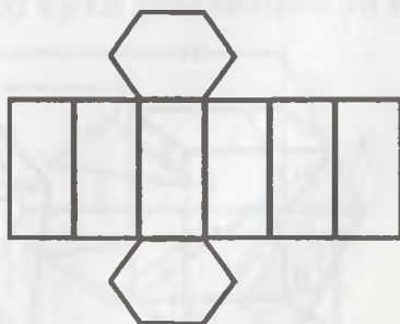
prizma yoyilmasi
