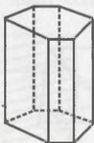
to'g'ri prizma
