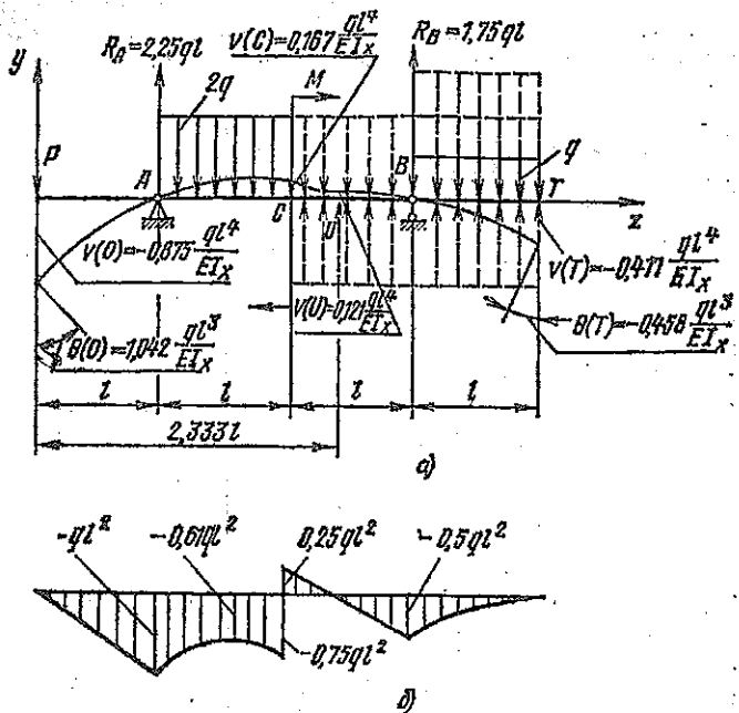
Рис. 9. Упругая линия статически определимой балки
