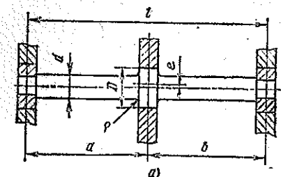
Рис. 21. Расчетная схема вращающегося вала с эксцентрично посаженным диском
