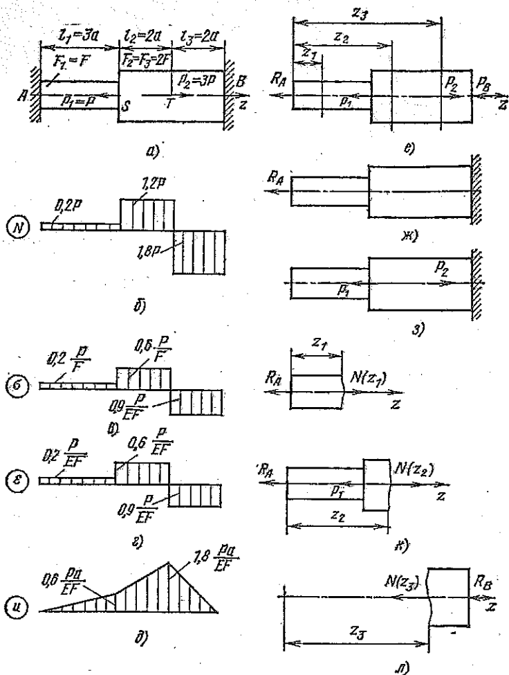
Рис. 4. Расчетная схема статически неопределимого ступенчатого стержня при растяжении-сжатии
