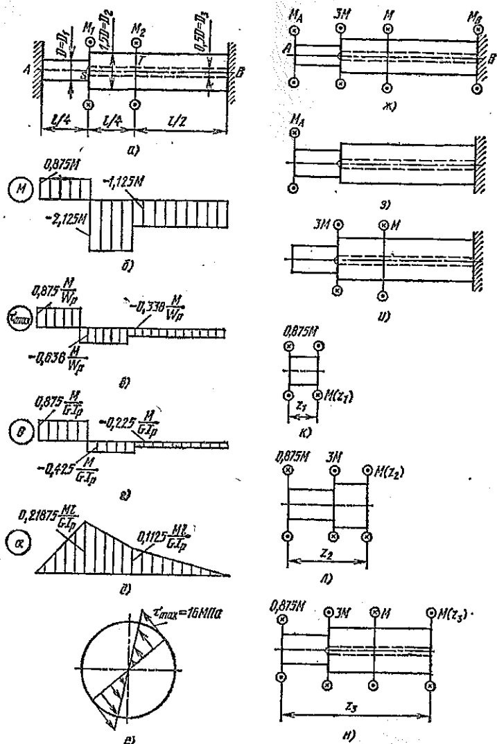
Рис. 6. Расчетная схема статически неопределимого круглого ступенчатого стержня при кручении
