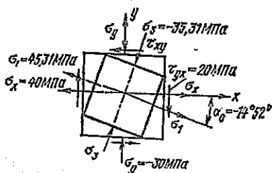
Рис. 19. Расчетная схема элемента, находящегося в условиях плоского напряженного состояния
