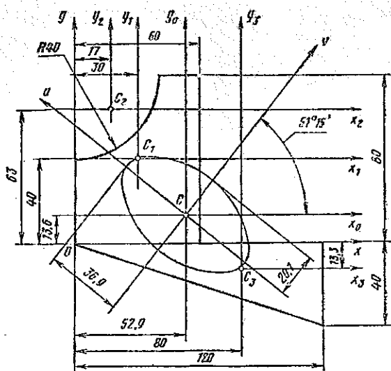
Рис. 25. Составное сечение
