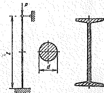
Рис. 23. Расчетная схема сжатого стержня, исследуемого на устойчивость
