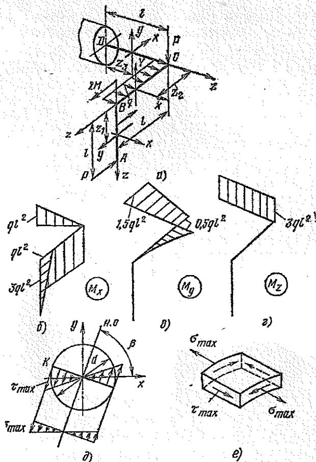
Рис. 18. Расчетная схема, эпюры внутренних моментов в напряжений в брусе круглого сечения с ломаной осью при произвольной нагрузке
