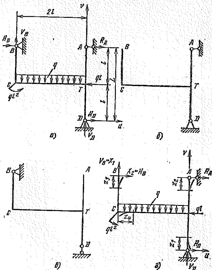
Рис. 11. Основная и эквивалентная системы плоской дважды статически неопределимой рамы
