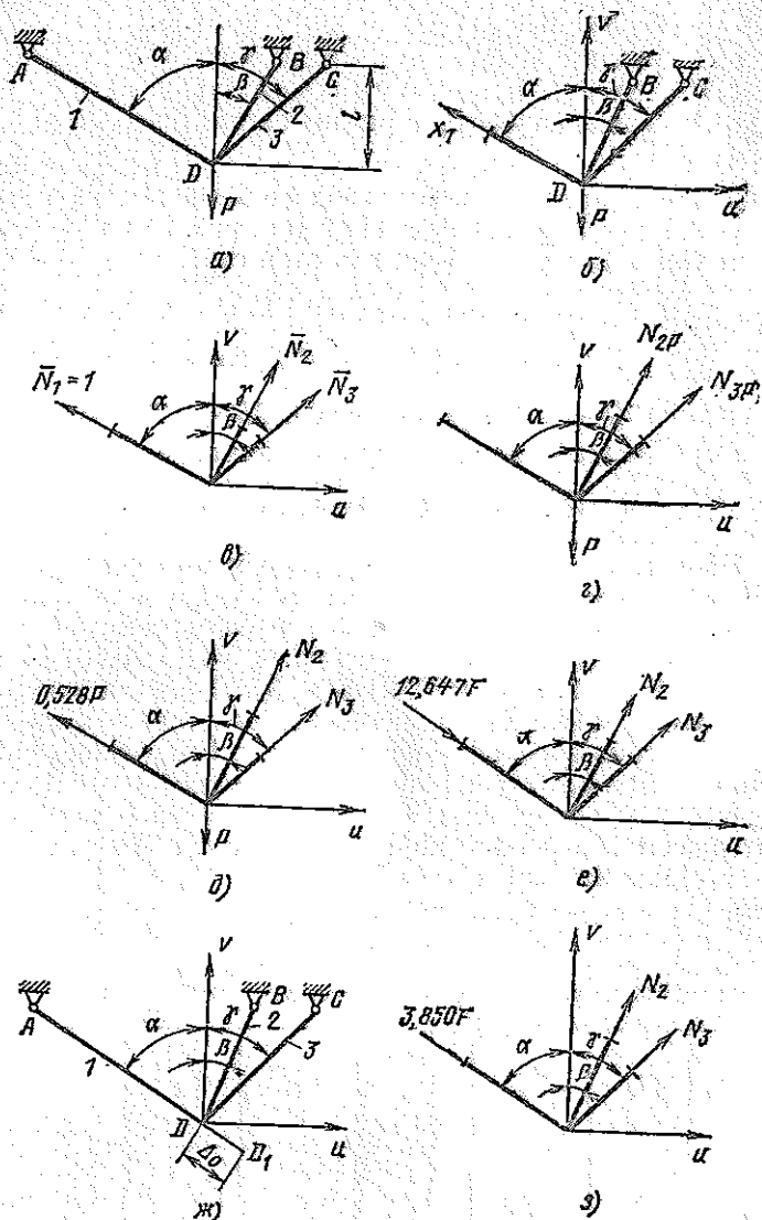
Рис. 2. Расчетная схема статически неопределимой плоской шарнирно-стержневой системы
