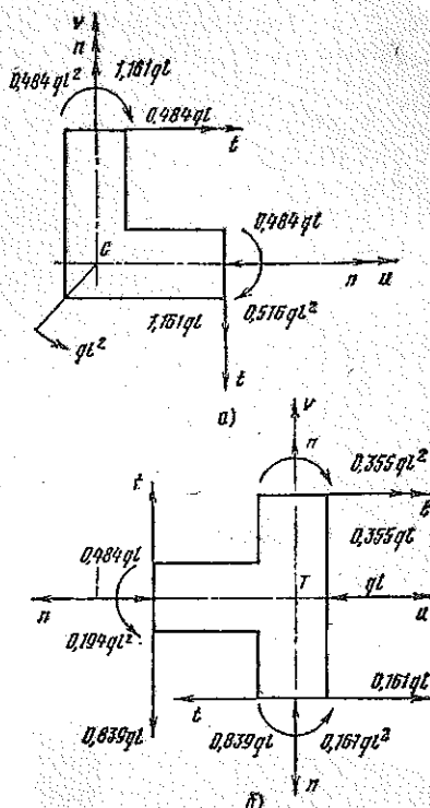
Рис. 15. Расчетная схема узлов дважды статически неопределимой плоской рамы
