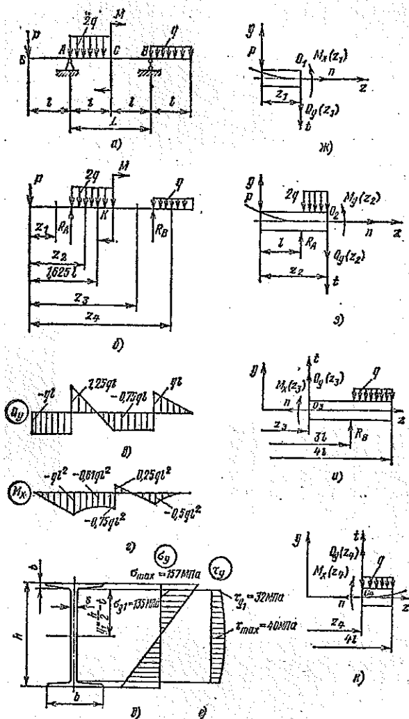
Рис. 8. Расчетная схема статически определимой балки
