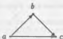
транзитивно
