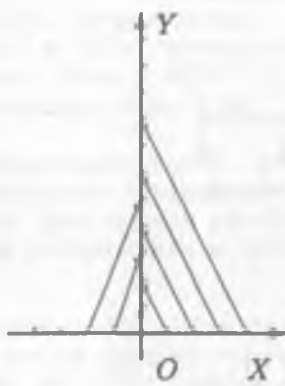
граф
