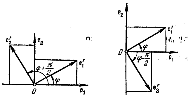
Рис. 14. Два случая взаимного расположения ортонормированных базисов на плоскости.
