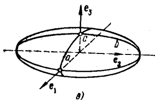
Рис. 46. а), б) Сжатый и вытянутый эллипсоиды вращения; в) эллипсоид.
