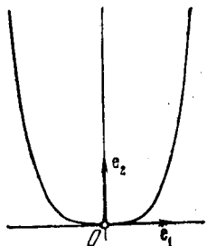
Рис. 27. Линия с уравнением y = x^4 .
