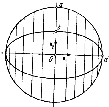
Рис. 29. Эллипс как сжатие окружности. Здесь b/a = 1/2 .
