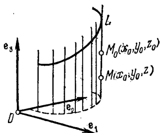
Рис. 16. L — направляющая, M_0M — образующая.
