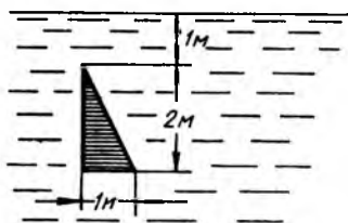
Прямоугольный треугольник
