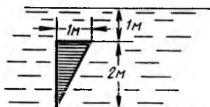
Прямоугольный треугольник
