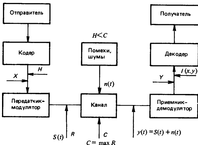
Блок-схема системы передачи информации
