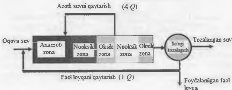
76-rasm. 5-bosqichli Bardenfo jarayoni sxemasi.
