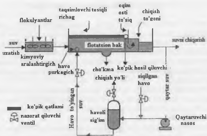
54-rasm. Ergan havoli flotatsiya qurilmasi sxemasi.
