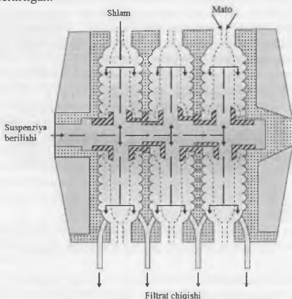
91-rasm. Belgilangan hajmli plastinali pressning ko'ndalang kesimining ko'rmishi
