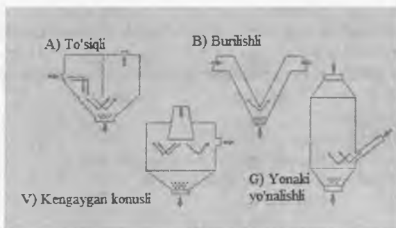
24-rasm. Inersion chang tutgichlar.
