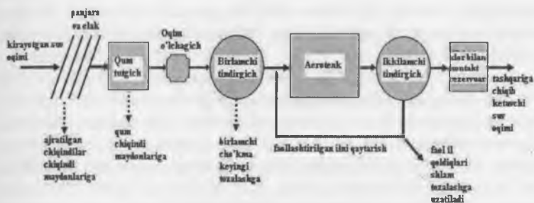
60-rasm. Ikkilamchi oqava suvlarni tozalash korxonalarida (WWTS) suyuqlikni qayta ishlash ketma-ketligi.
