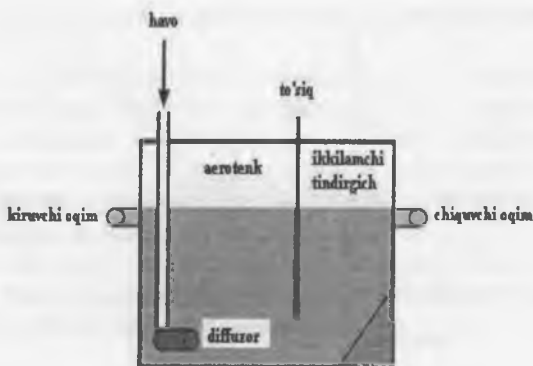
67-rasm. Faol il to'liq aralashuvchi laboratoriya reatori.
