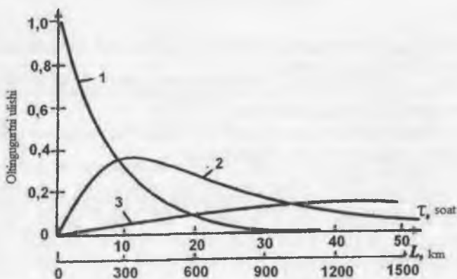
18-rasm. Atmosferada SO_2, H_2SO_4 va sulfatlarning miqdorini vaqt.
