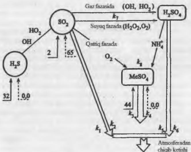
17-rasm. Oltingugurt birikmalarining atmosferadagi aylanma harakati sxemasi.
