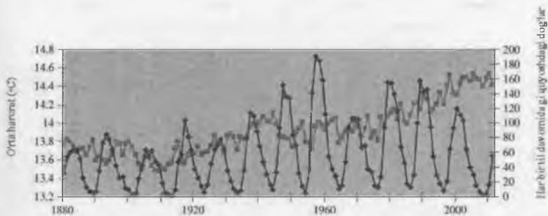
20-rasm. Quyoshdagi dog'larga nisbatan global harorat.
