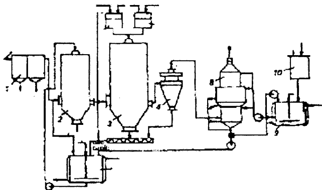
10.6-rasm. Tutun gazlarini azot va oltingugurt oksidlaridan tozalab gips hosil qiluvchi qurilma sxemasi:
