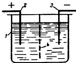
18.16-rasm. Elektrolizyor sxemasi:
