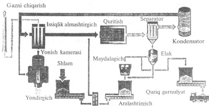
23.10-rasm. AHDRTZ firmasining shlamni qayta ishlab granulyat olish sxemasi.
