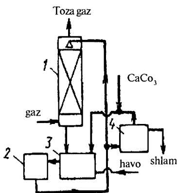
9.3- rasm. Oltingugurt dioksidini ohaktosh suspenziyasiga absorbsiyalash texnologik sxemasi (kalsiy sulfitni qurilmaning o‘zida oksidlash bilan):
