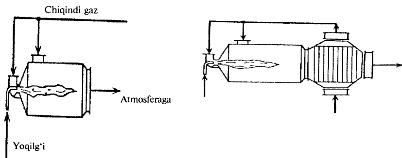
14.1-rasm. Sanoat chiqindi gazlarini termik zararsizlantirish (termik neytralizator) sxemasi:
