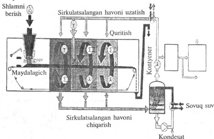
23.1-rasm. DORINER(Germaniya) firmasining shlamni sirkulatsiyalanadigan issiq havo bilan ishlov berish sxemasi:
