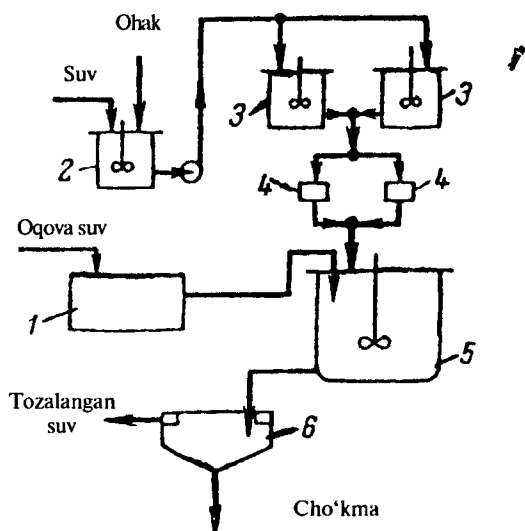
19.2-rasm. Kislotali oqova suvlarni kalsiy gidrooksidi ishtirokida neytrallash qurilmasi:
