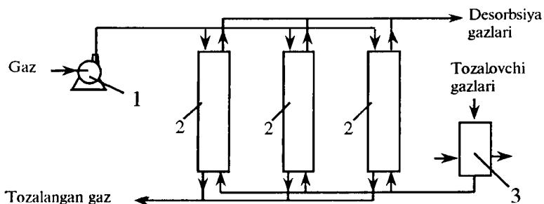
11.5-rasm. Seolit yordamida vodorod sulfidni adsorbsion usulda tozalash texnologik sxemasi:
