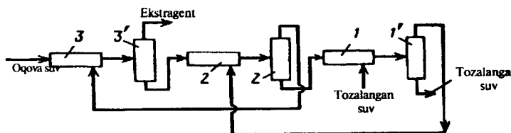
18.14-rasm. Ekstraktsion qurilma sxemasi: 1,2,3-aralashtirgich; 1',2',3'-tindirgich.
