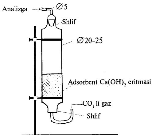
2-rasm. Absorber qurilmasi.
