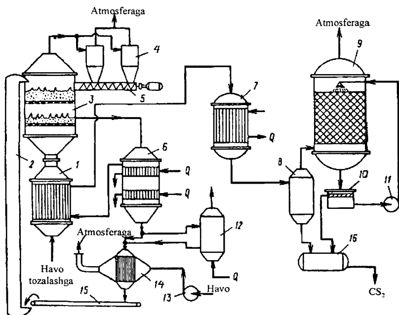
11.6-rasm. Viskoza sun'iy tola ventilatsion tashlamalarini CS_2 dan aktivlangan ko'mir yordamida absorbsion tozalash texnologik sxemasi:
