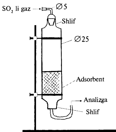
2-rasm. Absorber qurilmasi.
