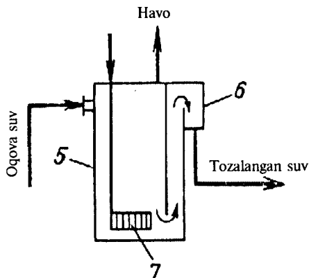
19.7-rasm. G'ovak plastinali barbotaj ozonlash apparati:
