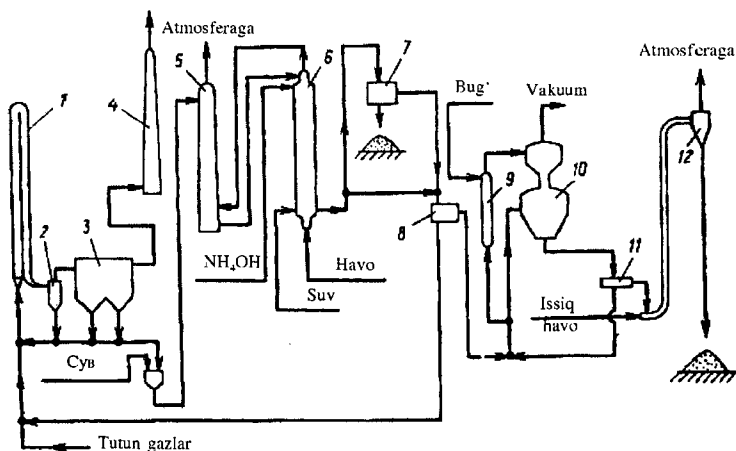
9.9-rasm. Tutun gazlarini oltingugurt dioksididan marganes oksidi asosidagi sorbent bilan tozalash texnologik sxemasi:
