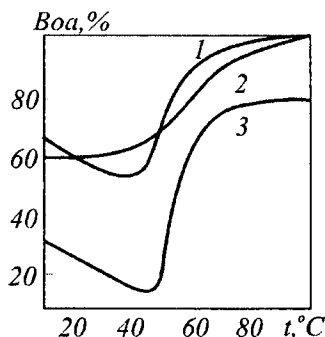
10.1-rasm. Tutun gazlarini azot oksidlaridan tozalash darajasining turli oksidlanish darajasidagi ( NO_x \alpha = [NO_2]/[NO+NO_2] ) haroratga bogʻliqligi:
