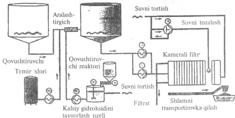
23.7-rasm. NETZSCH firmasining filtpressida ajratishga asoslangan shlamnlarni kimyoviy ishlov berish qurilmasi.
