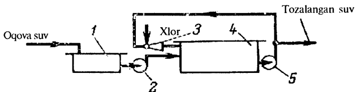
19.4-rasm. Oqova suvlarni xlorlash usulida tozalash:
