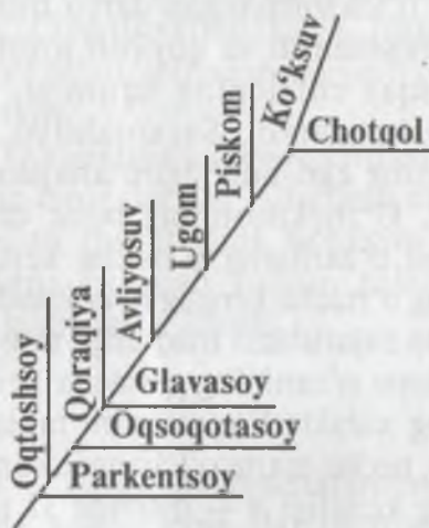
Chirchiq daryosining gidrografik tuzilishi.
