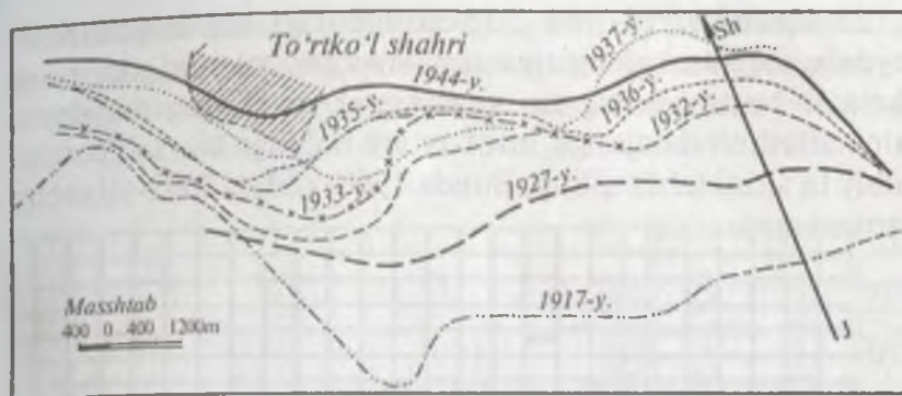
12-rasm. Degish natijasida To'rtko'l shahri yonida Amudaryo o'ng qirg'og'ining siljish sxemasi (1917—1944-yillar).
