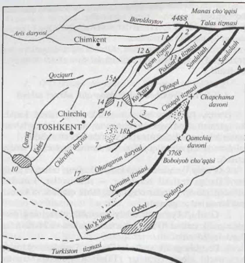
24-rasm. G'arbiy Tyanshan tabiiy-geografik okrugining orografik chizmasi.
