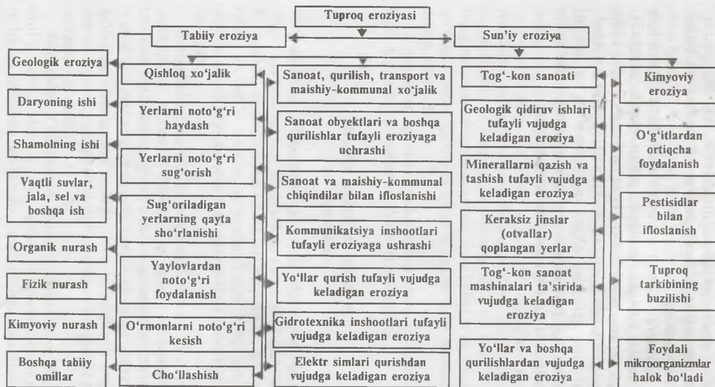
20-rasm. Tuproq eroziyasi va uning ifloslanishi.
