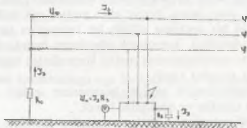
34-rasm. Yerga ulash chizmasi.
