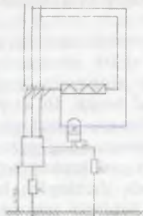
35-rasm. Muhofazalovchi o'chirish qurilmasi.
