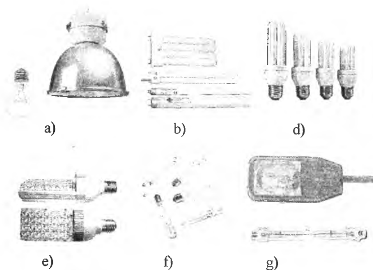
6.5-rasm. Yoritgichlar tuzilishi va turlari:
