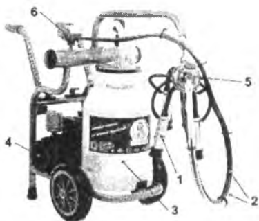
8.13-rasm. Ko'chuvchan sut sog'ish apparati:
