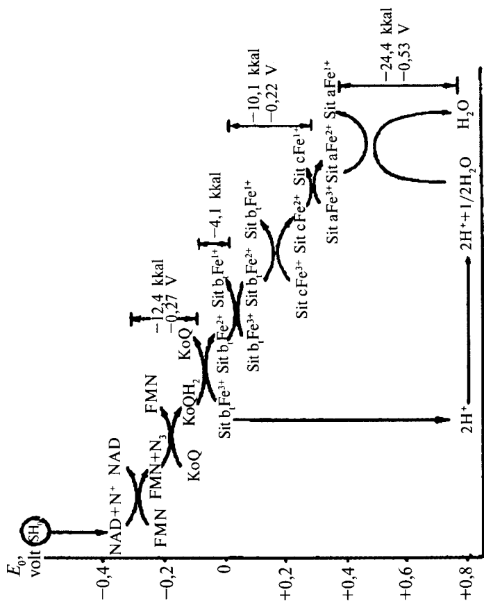
11-rasm. Elektronlarni olib o'tuvchilarning ketma-ket joylashishi.
