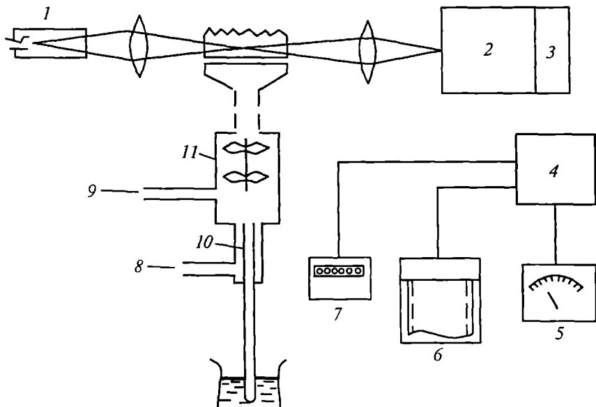
21-rasm. Atom-absorbsion spektrometrining blok-sxemasi.
