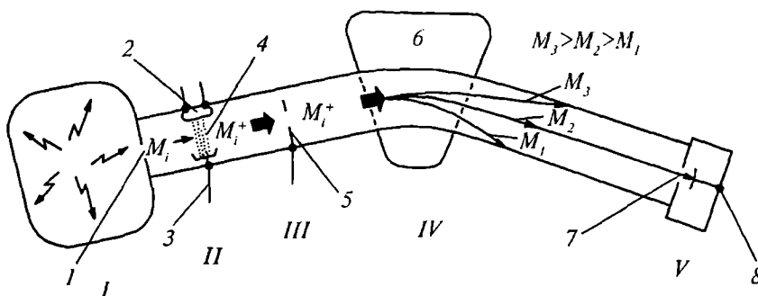
12-rasm. Bir martali fokusirovkali magnitli mass-spektrometr sxemasi;
