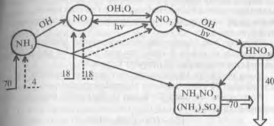
18-rasm. Azot birikmalarining atmosferadagi aylanma harakati:
