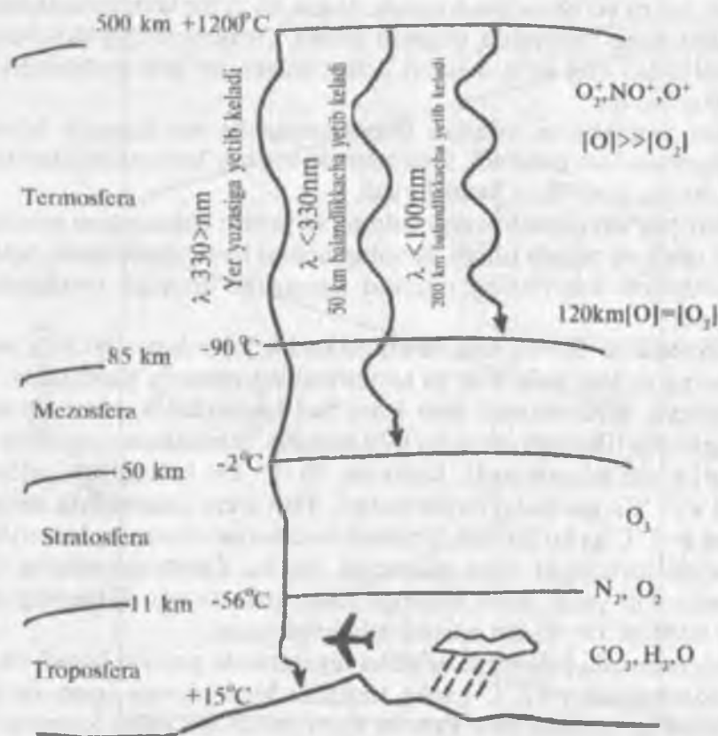
4-rasm. Atmosferaning tuzilishi sxemasi.
