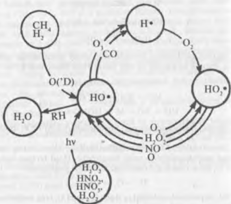
13-rasm. Gidroksil radikalining atmosferadagi kimyoviy o'zgarishlari.
