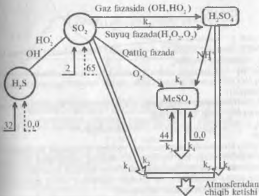
16-rasm. Oltिंगugurt birikmalarining atmosfera dagi aylanma harakati sxemasi.
