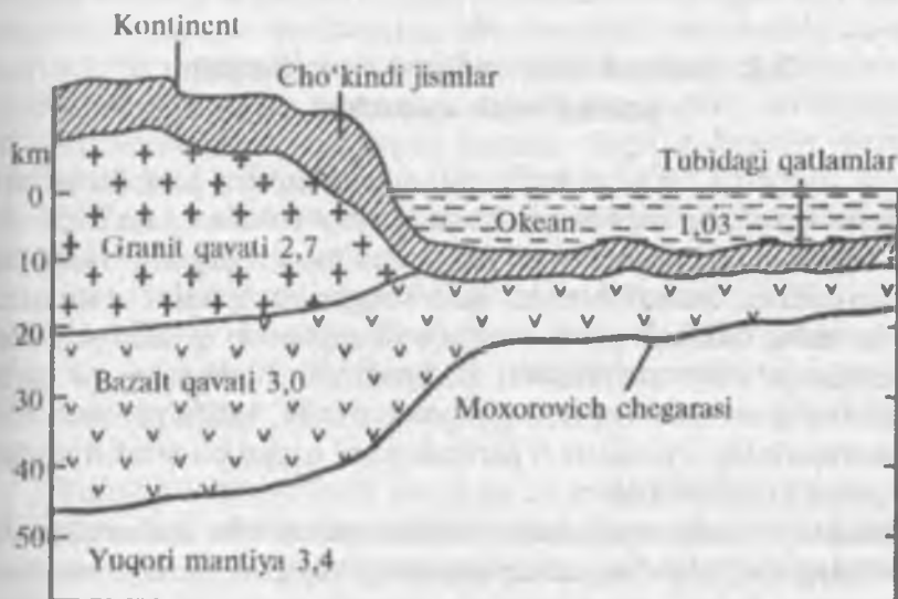
3-rasm. Yer qatlamining tuzilishi sxemasi. Keltirilgan sonlar moddaning zichligini \text{g}/\text{sm}^3 da ko‘rsatadi.
