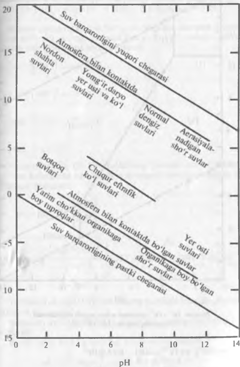
24-rasm. Suvning barqarorlik chegaralari.
