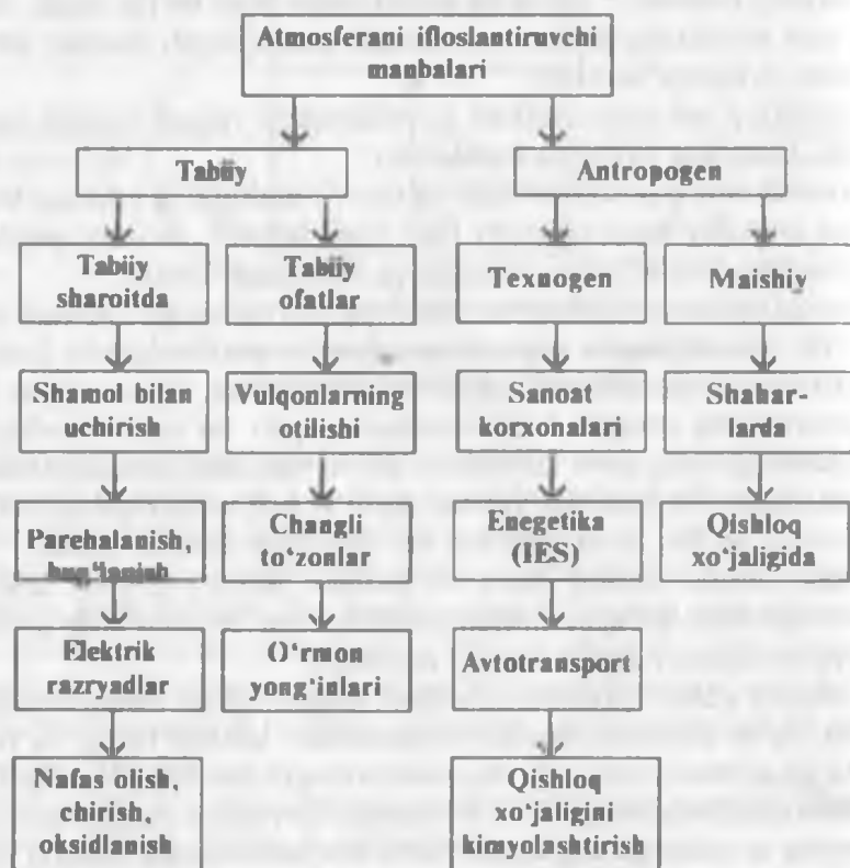
7-rasm. Atmosfera havosini ifloslantiruvchi manbalar.
