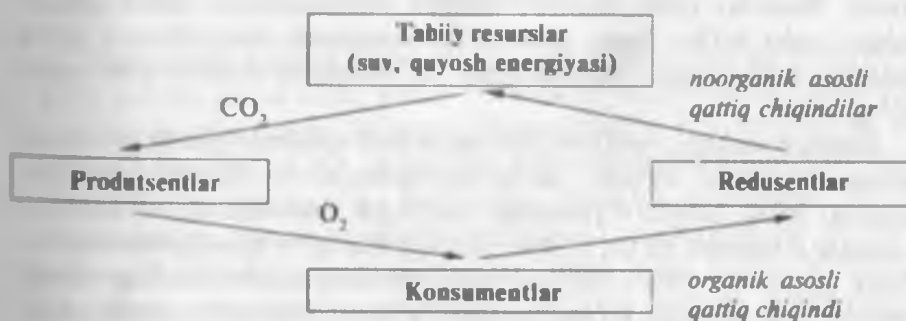
1-rasm. Biosferada moddalarning aylanma harakati.
