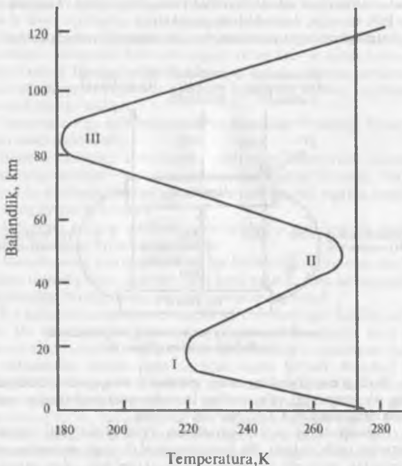
5-rasm. Atmosferada balandlik bo'yicha temperaturaning o'zgarishi.
