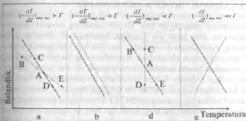
8-rasm. Atmosferadagi temperaturaning balandlik bo'yicha o'zgarishi:
