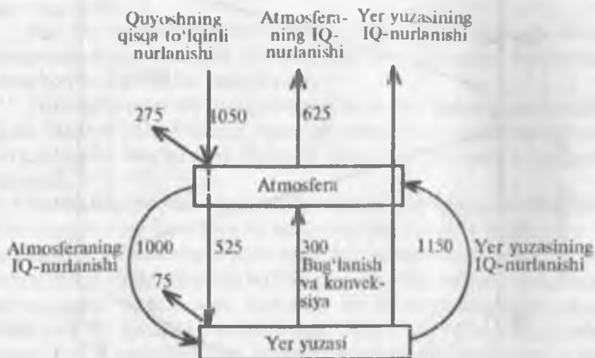
6-rasm. Atmosfera va yer yuzasining issiqlik balansi (radiatsiya oqimlari \text{qJ/sm}^2\text{-yil} )
