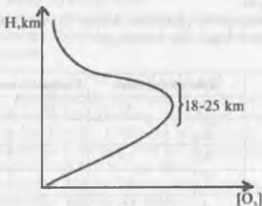
12-rasm. Ozonning miqdorini balandlik bo'yicha o'zgarishi.
