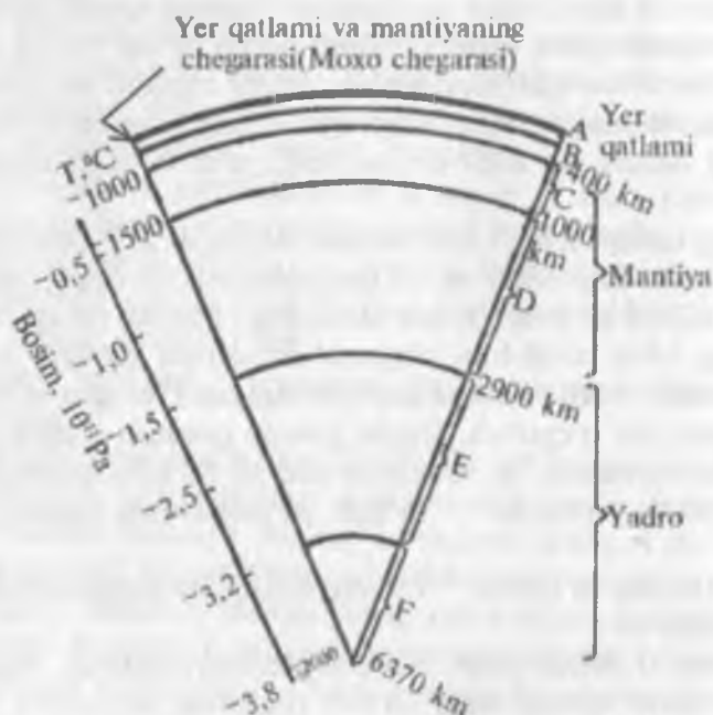
2-rasm. Yerning ichki tuzilishi sxemasi:
