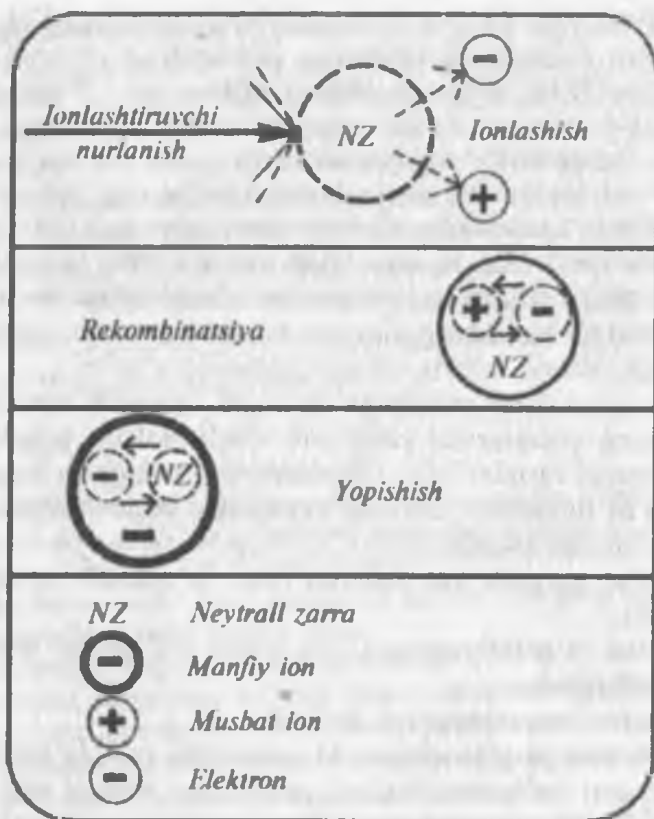
10-rasm. Yuqori atmosferada zarralarning o'zgarishi.
