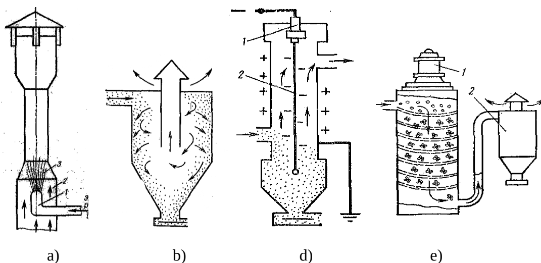
6.8-rasm. Ishlab chiqarish binolarida havoni tozalab beruvchi ejektorli (a), siklon (b) elektrli (d) va ultrotovshli (e) filtrlar.
