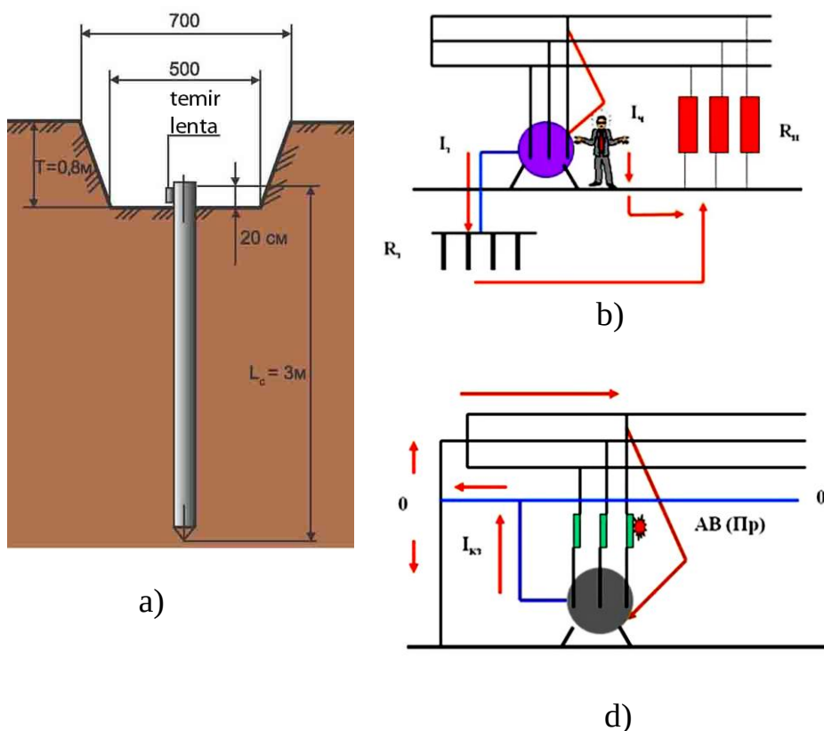
9.4-rasm. Uskuna va elektr qurilmalarni himoyalovchisini yerga a), b) va nolga d) ulash sxemasi
