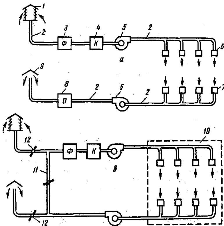
6.9-rasm. Mexanik ventilyatsiyalar sxemasi.
