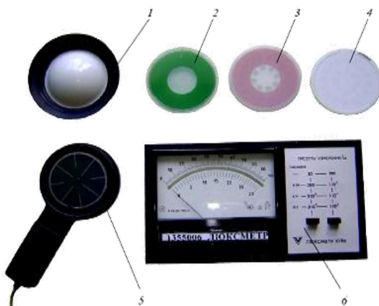
6.6 -rasm. IO-16 fotoelektrik lyuksometrning tashqi ko'rinishi. 1 – yarim sfera shakldagi biriktirish halqasi; 2,3,4 – turli yoru'g'likni pasaytiruvchi koeffitsientga ega bo'lgan membranalar; 5 - fotoelement; 6 millivolmetr.
