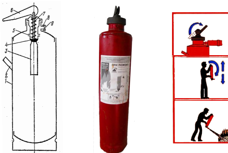
10.7 -rasm. OXP -10 o't o'chirgichi tuzilishi va undan foydalanish tartibi: 1-korpus; 2-tutqich; 3-stakan (ishqor turadigan); 4-rezinali klapan (stakan og'zini germetik yopish uchun); 5-stakan kanallari; 6- klapan holatini o'zgartiruvchi dastak; 7-klapan shtoki; 8- sepbish kanali; 9-yopgich membranasi.
