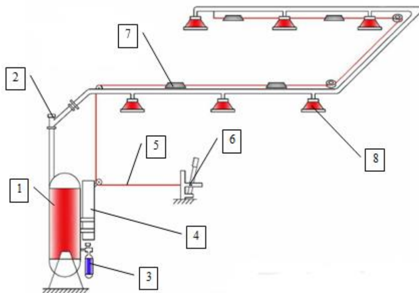
10.1-rasm. Mahalliy yong'inni o'chiruvchi avtomatik kukunli yong'in o'chirgich sxemasi Belgilar: 1 – o't o'chirgich; 2 - pnevmatik klapan; 3-Siqilgan gazli ballon; 4-yo'naltiruvchi quvur; 5-simarqon; 6 – qo'lda qo'shish dastasi; 7 - yengil eruvchi qulf; 8 – sochuvchi jikler.
