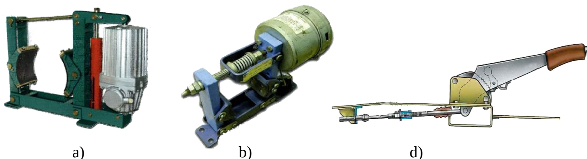
8.2-rasm. Kolodkali (a), elektromagnitli (b) va mexanik yuritmal (d) tormozlar
