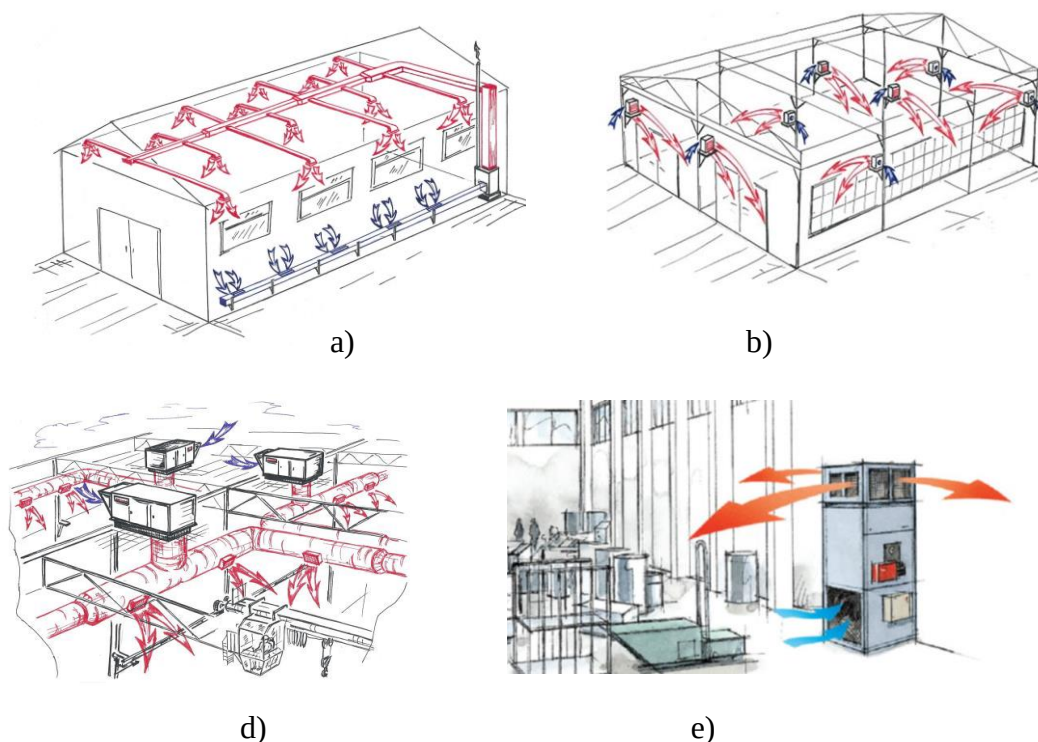
6.7–rasm. Bino va ish joylarini isitish tizimi. a, b -to'la mahalliy isitish; d-tug'ridan-to'g'ri binoni to'la isitish; e- mahalliy isitish
