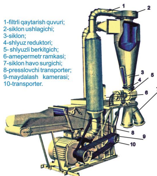
8.12-rasm. КДУ-2 dag'al ozuqa maydalagichi
