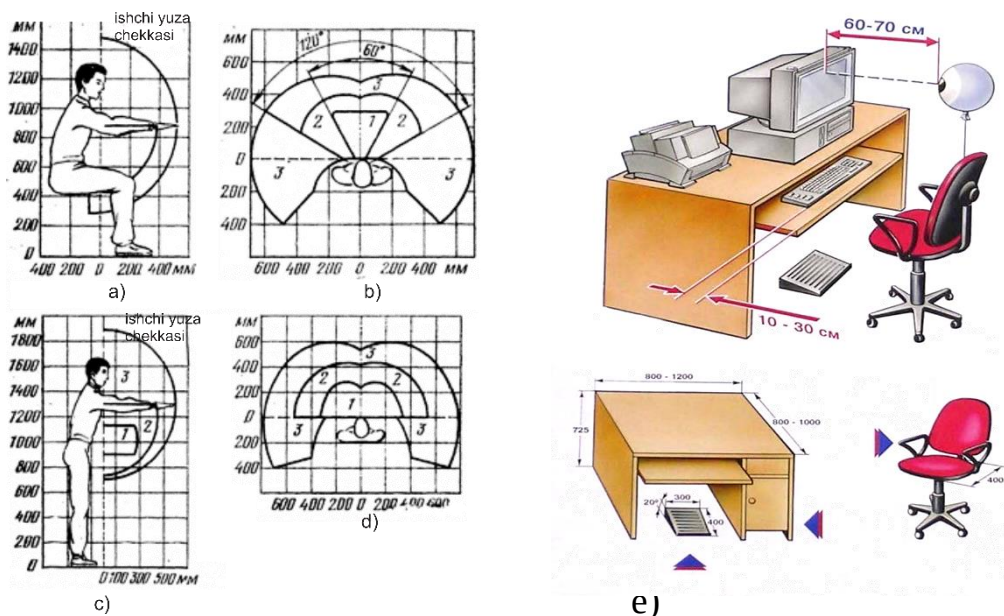
1.3-rasm. O’rta bo’yli odamni boshqaruv a’zolarini joylashtirish uchun harakatlar maydoniga yoyish doirasi va ish o’rni. a) va b) – o’tirgan holatda vertikal va gorizontal teksilikda yoyish doirasi; c) va d) – tik turganda vertikal va gorizontal tekislikda yoyish doirasi; e) – kompyuter operatorinig ish o’rni geometrik o’lchamlari: 1 – tez-tez ishlatiladigan va muhim boshqaruv organlari joylashuvi; 2 – tez-tez ishlatiladigan va muhimligi kam bo’lgan boshqaruv organlari; 3- kam ishlatiladigan boshqaruv organlari.
