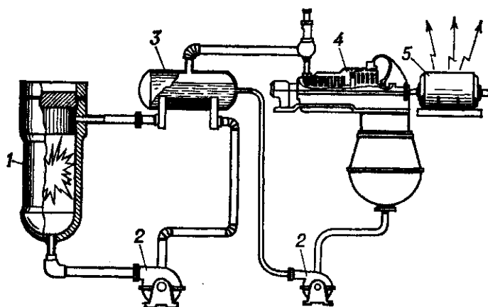
11.1-rasm. Atom elektrostansiyasi tuzilishi.
