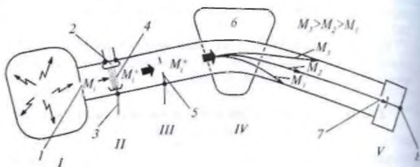
12-rasm. Bir martali fokusirovkali magnitli mass-spektrometr sxemasi; I—namuna rezervuari; II—ionizatsiya zonasi; III—tezlashish zonasi; IV—analizator; V—detektor. 1—tomizuvchi; 2—qizdiriladigan katod; 3—anod; 4—elektronlar tutami; 5—elektrodlar; 6—magnit; 7—kollektor teshigi; 8—elektrik datchik.
