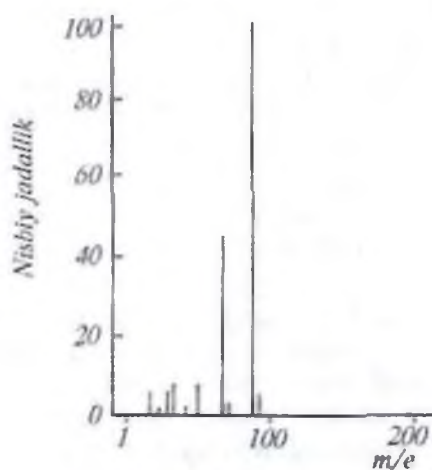
13-rasm. Oltinugurt tetraftoridining mass-spektri.
