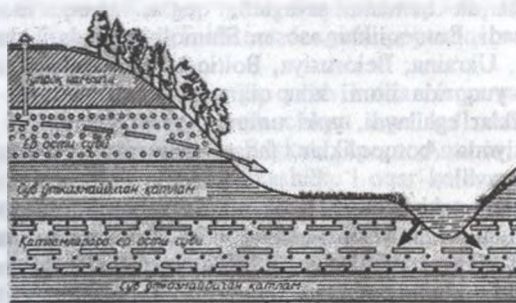
Yer osti suvlarning joylashish sxemasi.
