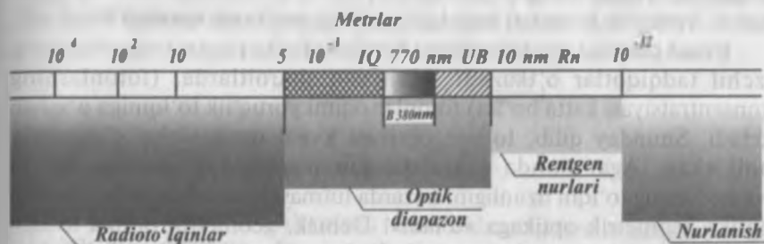
38-rasm. Elektromagnit to'liqlar shkalasi.
