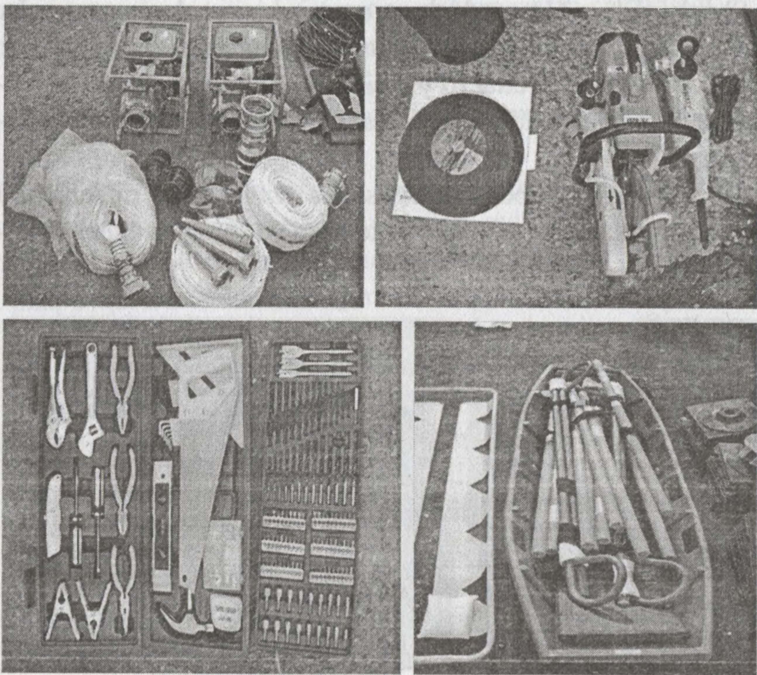
20-rasm. AQI maxsus jihozlari.
