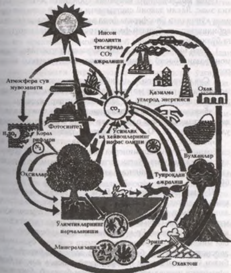
10-расм. Биосферада \text{CO}_2 нинг айланиш ҳаракати.
