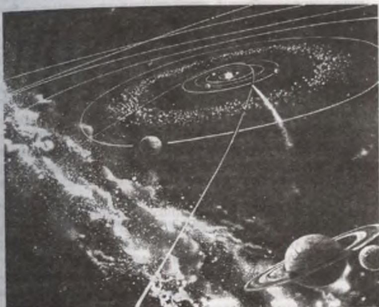
2-расм. «Сомон йўли» Галактикаси, Қуёш тизими (14)
