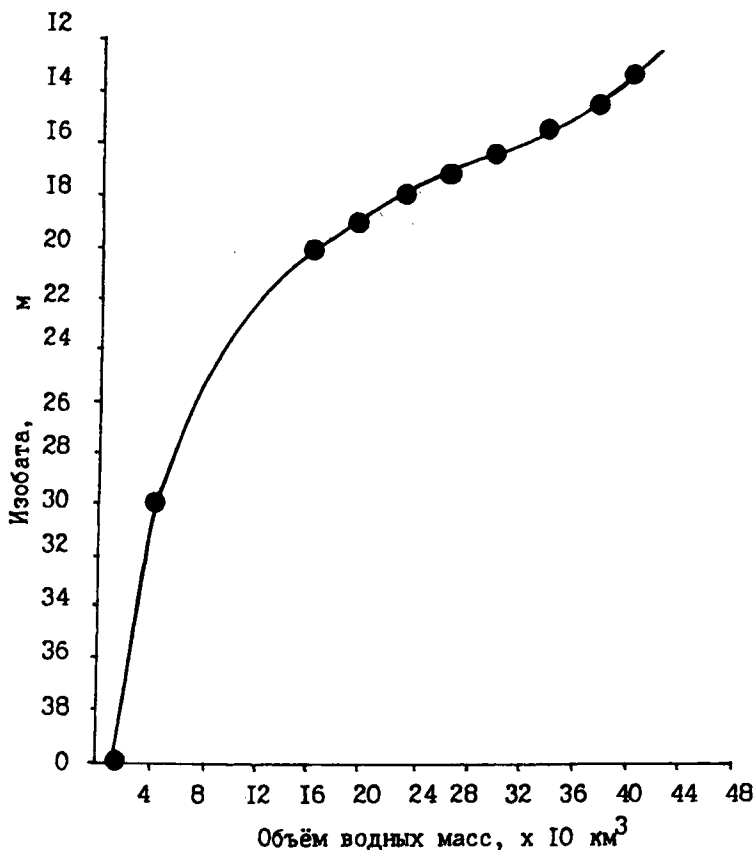
Рис.3.12. Зависимость объема водных масс Аральского моря от изобат (абсолютной отметки зеркала воды)
