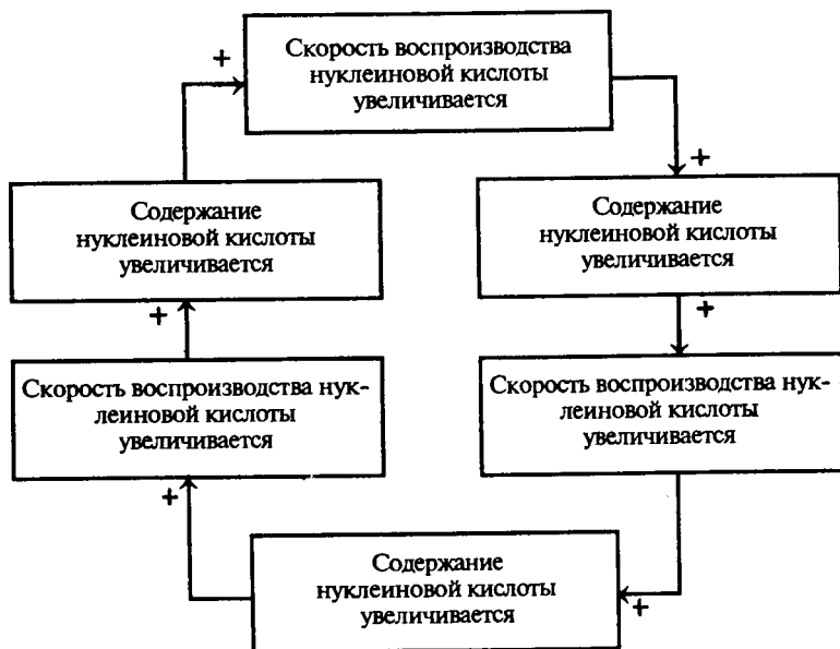
Рис. 2.20. Схема связей в циклической системе белково-нуклеиновых молекул (по М. Эйгену, 1973)
