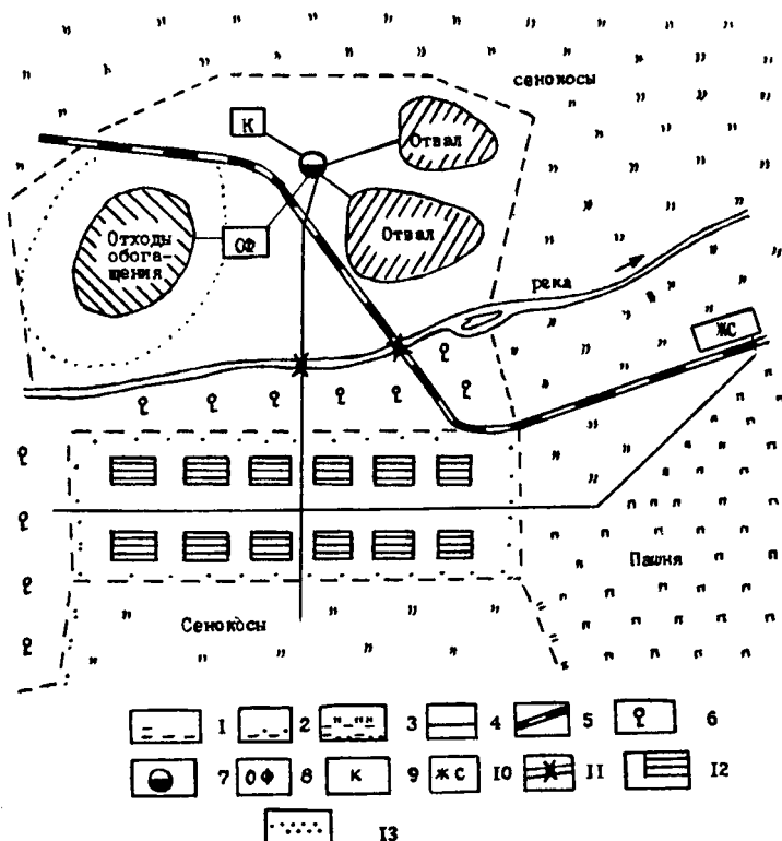
Рис. 1. Экологическая карта-схема:
