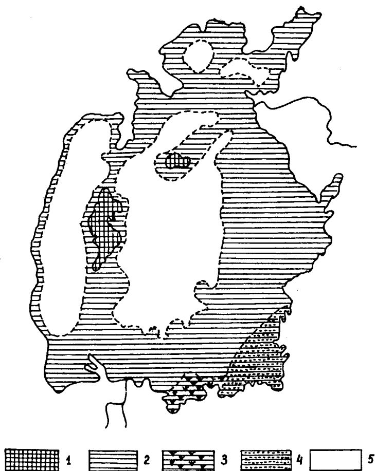
Рис.3.10. Изменение берегов Аральского моря в результате снижения его уровня (в течение 1961—2000 гг.)
