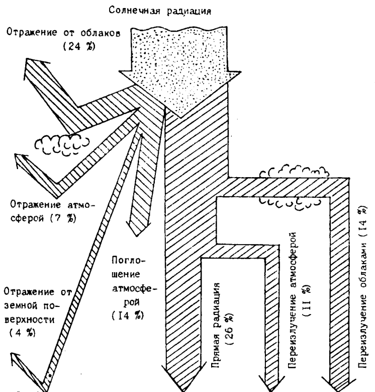
Рис. 2.12. Солнечная радиация в системе Земля — атмосфера
