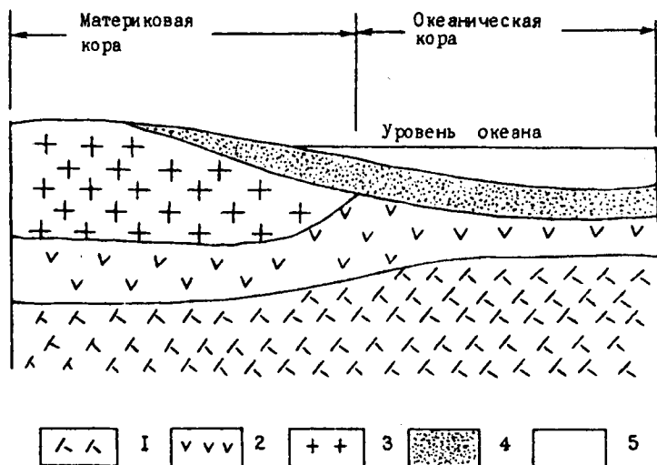
Рис. 3.1. Строение земной коры: 1—верхняя мантия; 2—базальтовый слой; 3—гранитный слой; 4—осадочный слой; 5—толща океанической воды
