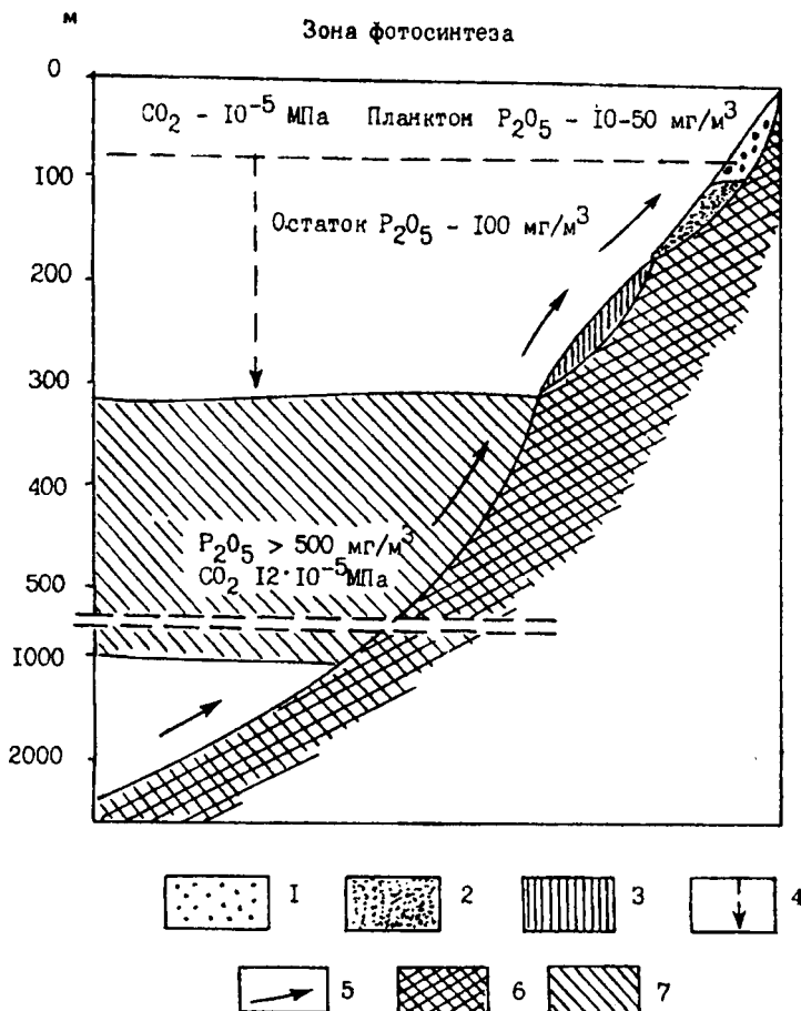
Рис. 2.23. Схема фосфоритообразования (по А.В. Казакову) 1—фашия береговых отложений; 2—фосфоритно фашия; 3—фашия известковых осадков; 4—падение остатков планктона; 5—направление течений; 6—коренные породы дна моря; 7—зона максимума \text{CO}_2 и \text{P}_2\text{O}_5 в растворе
