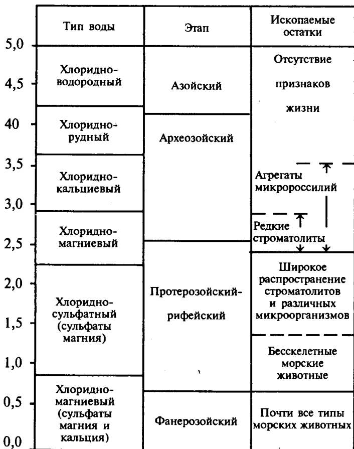
Рис. 3.8. Эволюция химического состава гидросферы и ее связь с нахождением остатков ископаемых организмов
