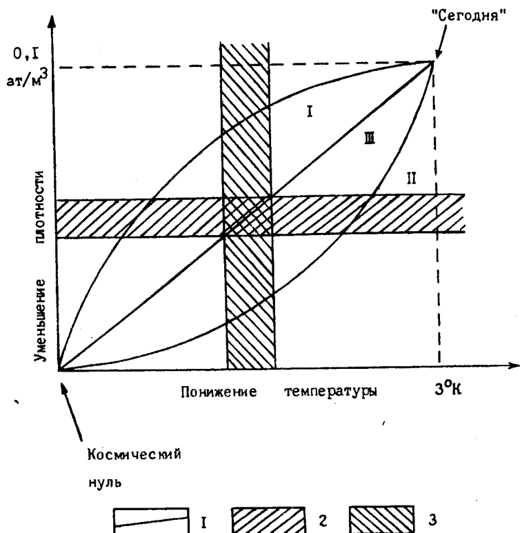
Рис.3.4. Модель расширяющейся Вселенной в связи с возможностью существования первого космологического периода:
