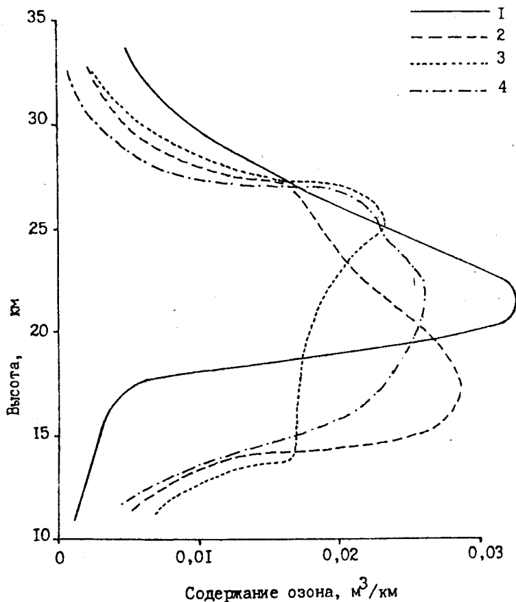
Рис.3.14. Вертикальное распределение озона в атмосфере над Нью-Мексико (Regener, 1950):
