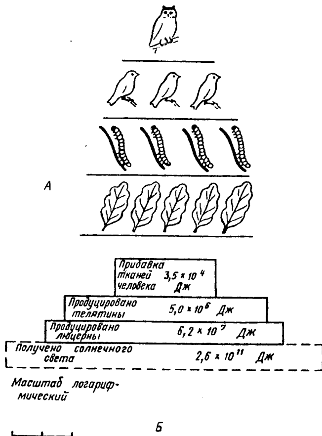
Рис. 2.14. А — Классическая пирамида чисел Элтона (Elton, 1927). Б — Энергетический вариант пирамиды для конкретной сельскохозяйственной системы (пересчитано в системе СИ; данные Ю. Одума, 1975)
