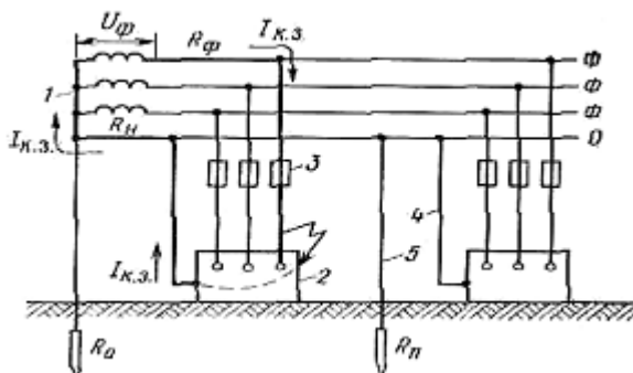
1- трансформатор нейтрал; 2- электр токи қабул қилувчи ускунанинг қобиғи; 3- эрувчан сақлагичлар; 4- нол билан уловчи ўтказгич; 5- нолинчи симни қайта ерга улагич. 10-расм. Нол сим ёрдамида ҳимоялаш схемаси:
