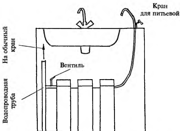
Рис. 6. Стационарный фильтр из трех патронов
