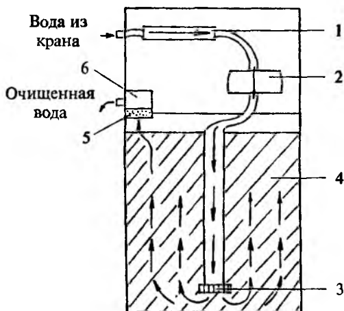
Рис. 10. Схема очистки воды в фильтрах компании «ЭКО-АТОМ»
