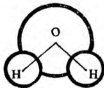
Рис. 1. Молекула воды
