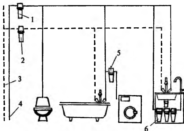
Рис. 8. Полифункциональный комплект водоочистительного оборудования 1 — предфильтр для холодной воды; 2 — предфильтр для горячей воды; 3 — труба подачи горячей воды; 4 — труба подачи холодной воды; 5 — предфильтр для стиральной машины; 6 — стационарный фильтр.
