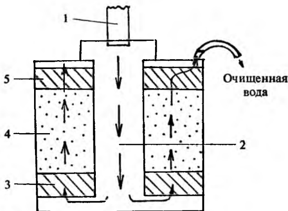
Рис. 7. Разрез фильтра «Аквафор В300»
