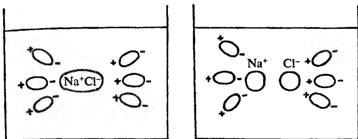
Рис. 2. Процесс диссоциации
