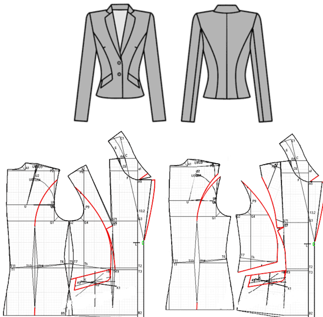
44-rasm. Ayollar pidjagi konstruksiya baza asosiga model xususiyatlarini qo'chirish
