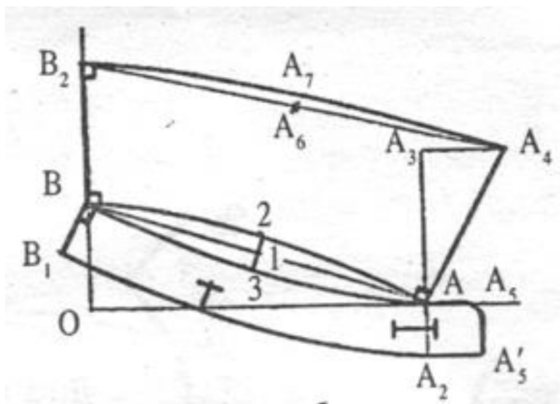
65-rasm. Kesma tik asosli qaytarma yoqa
