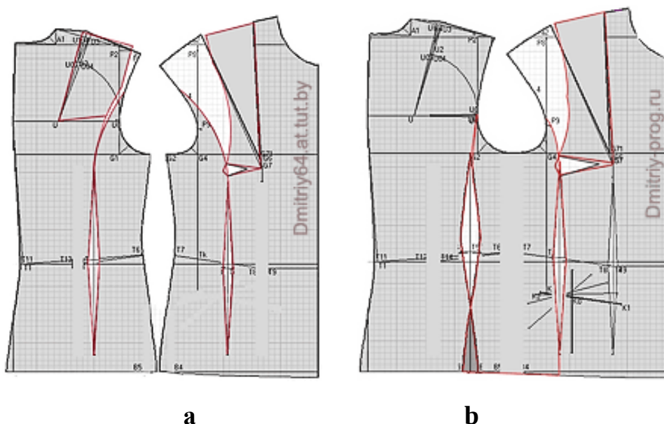
22-rasm. Bel vitochkalarini bo'rtma choklarga o'tkazish: a- yon choklari mavjud kiyim; b- yon choklarsiz kiyim
