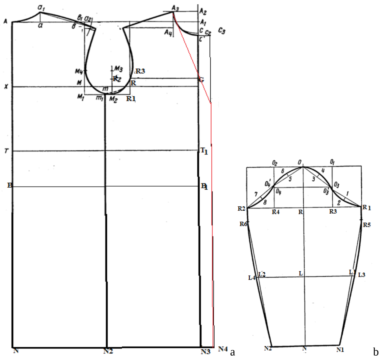
200-rasm. Erkaklar chopononing konstruksiya chizmasi:a-old va orqa detallari, b-yeng detali
