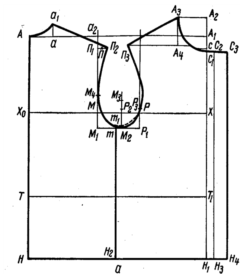
153-rasm. Sport va dam olish uchun mo'ljallangan jaketning konstruksiyasi jaketning old va ort detallari
