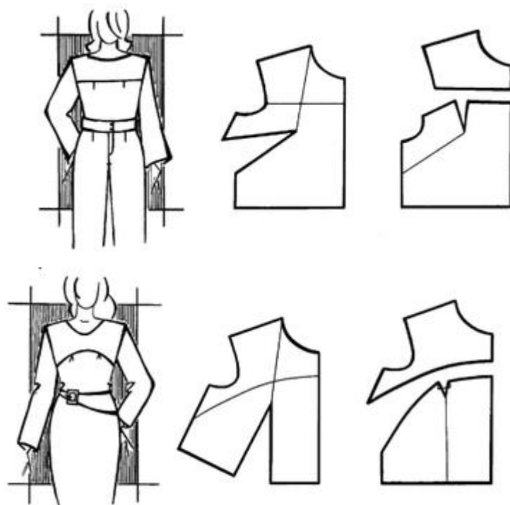
20-rasm. Ayollar kiyimining old bo'lagining yuqori qismini gorizontal bo'laklash usulini qo'llab koketkalar hosil qilish
