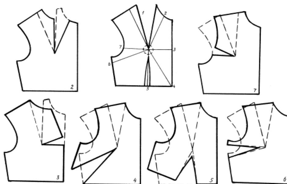
13- rasm. Ko'krak vitochkasini ko'chirish yo'nalishlari
