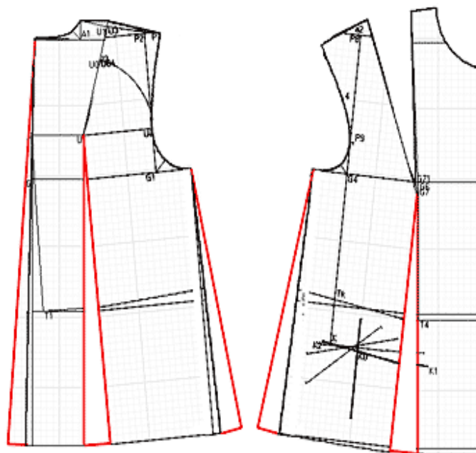
38-rasm. Ayollar kiyimini konussimonsimon kengaytirish
