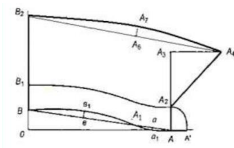
66-rasm. Tik asosi bilan yaxlit bichilgan qaytarma yoqa
