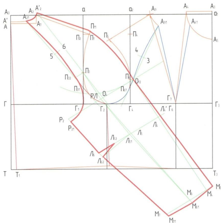
52- rasm. Reglan bichimli yengning orqa bo'lagining konstruksiya chizmasi
