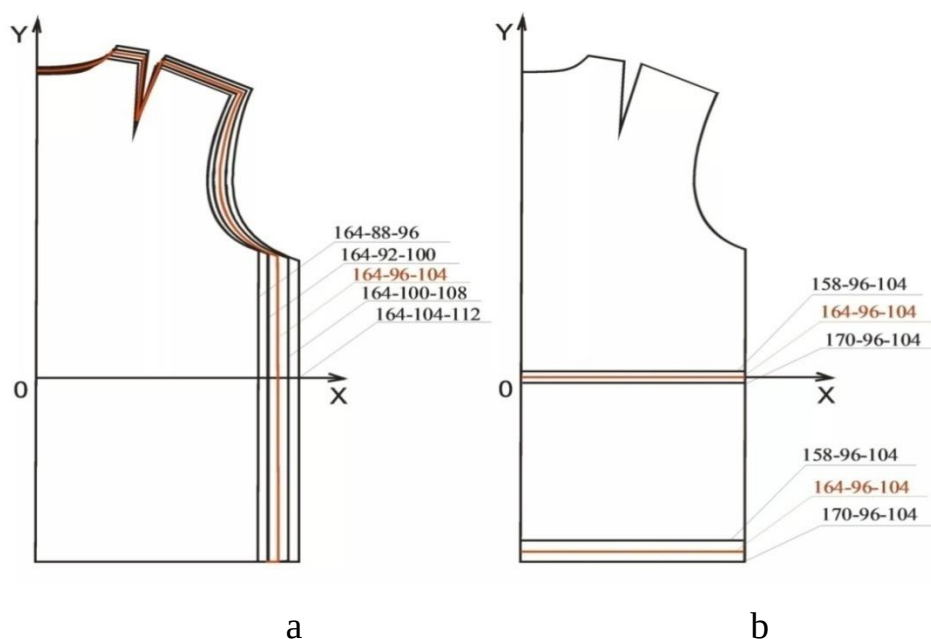
118-rasm. Andazalarni gradatsiyasining proporsional- hisoblash usuli a- razmerlar bo'yicha; b- bo'ylar bo'yicha
