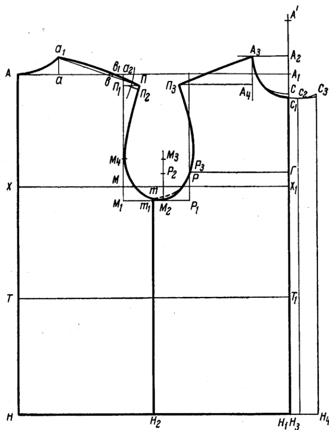
139-rasm. Jemperring orqa va old bo'lak chizmasi
