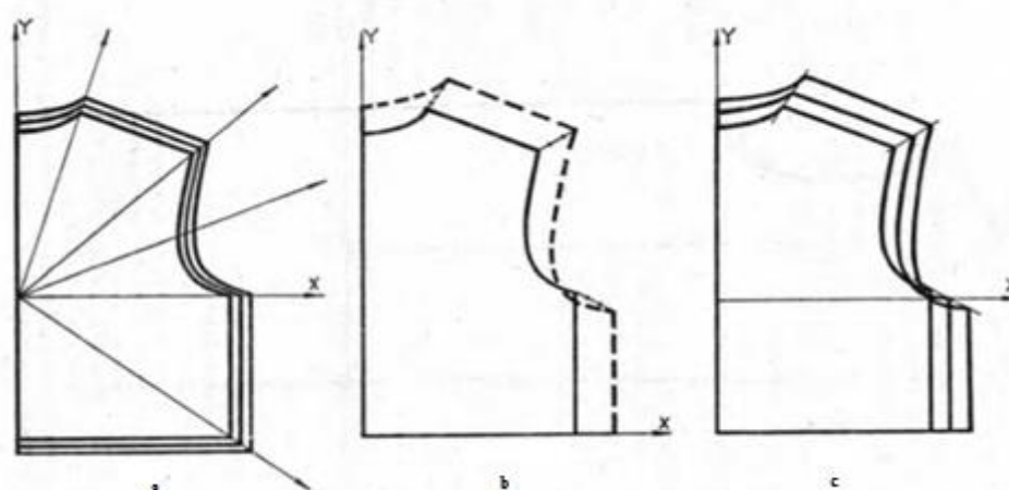
117-rasm. Andazalarni turli usulda gradatsiyalashda konstruktiv nuqtalari surilishi: a — guruhlash; b — nurlar; c — proporsional hisoblash usullari
