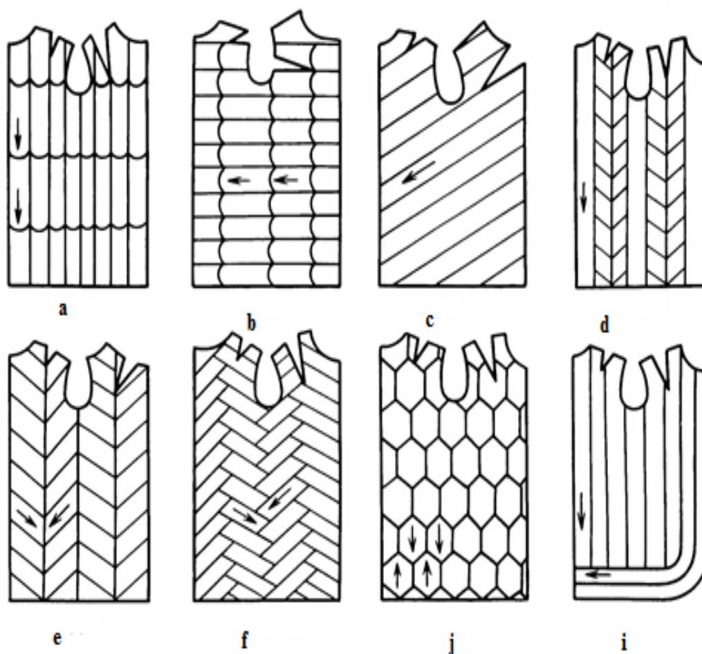
207 - rasm. Buyumlarda terilarning joylanishi: a - bo'ylama; b - ko'ndalang; c - diagonal bo'yicha; d - archasimon; f - parketsimon; j – shaxmatli; i – Kombinatsiyalashtirilgan
