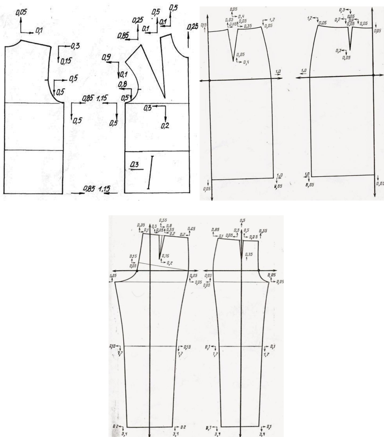
119-rasm. Kiyim detallarini razmerlar bo'yicha (X -strelkali belgilangan) bo'ylar bo'yicha (Y- aylanali strelka bilan belgilangan) gradatsiyasining sxemasi
