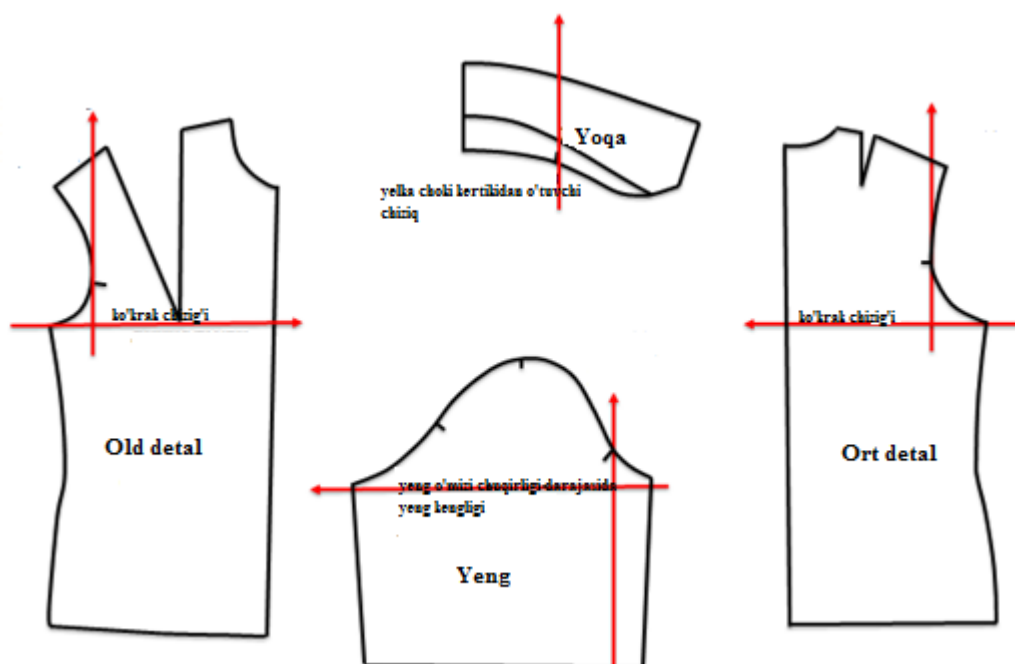
122-rasm. Ayollar kiyimi detallarida gorizontaal va vertikal orttirmalar yo'nalishi
