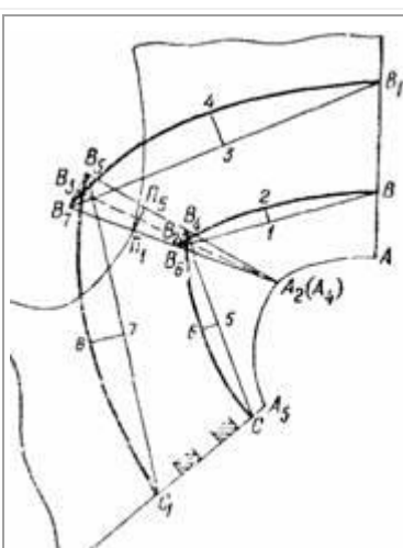
82-rasm. Bo'yindan uzoqroq fantastiy ayoqani modellastirish chizmasi
