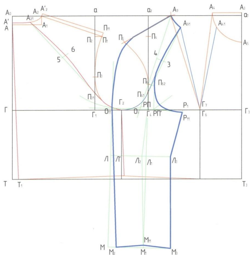
51- rasm. Reglan bichimli yengning old bo'lagining konstruksiya chizmasi
