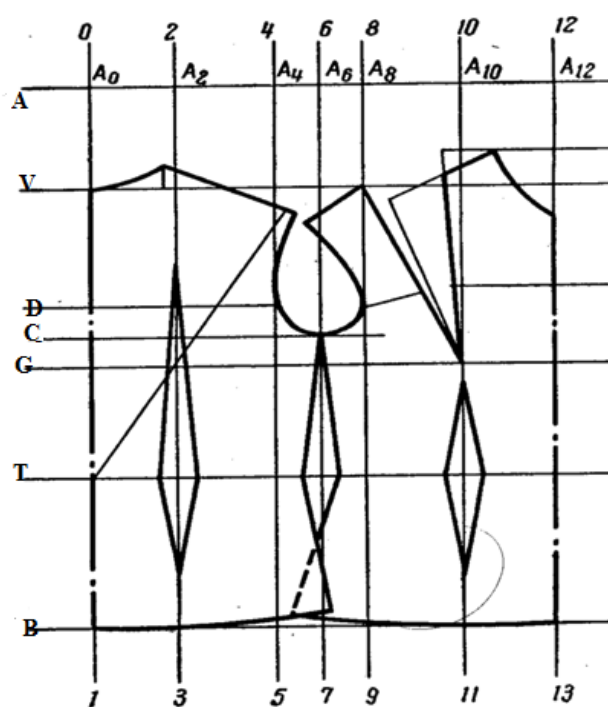
135-rasm. Ayollar trikotaj kiyimining konstruksiya chizmasi
