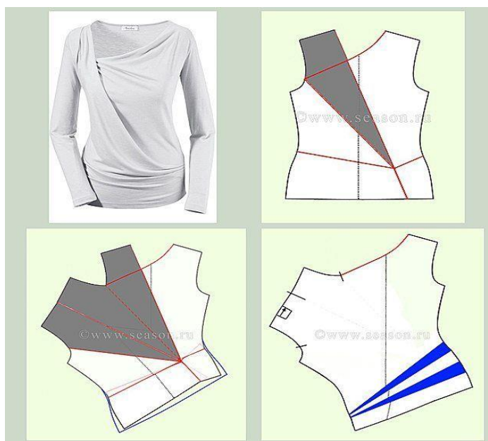
158-rasm. Trikotajdan ayollar kiyimini modellashtirish: detallarni konussimon kengaytirish
