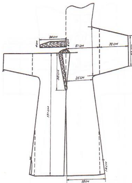
173-rasm Erkaklar milliy zardo'zlik buyumlarining bichimi
