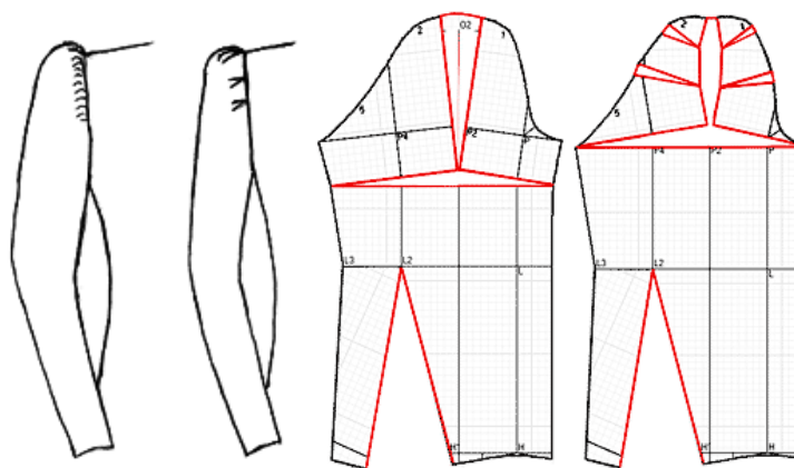
29-rasm. Ustki qismi kattalashtirilgan hajmli yeng
