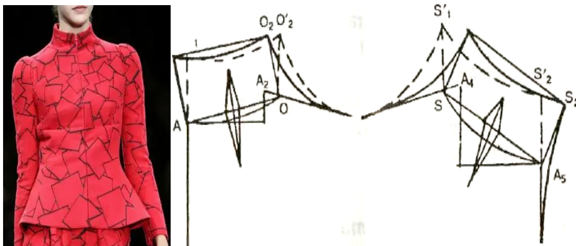
68-rasm. Old va orqa bo'laklar bilan yaxlit bichilgan tik yoqa
