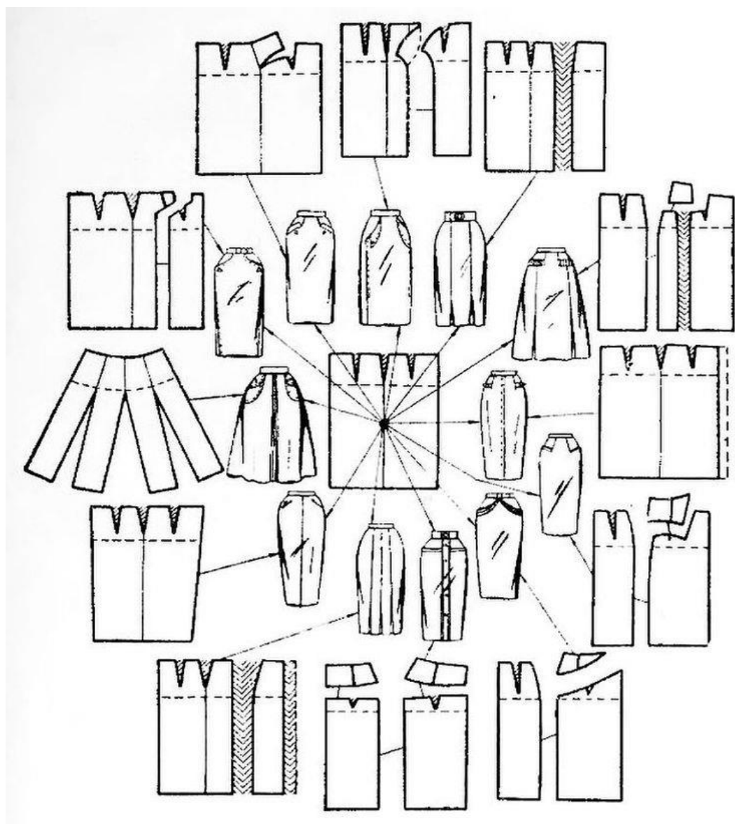
91-rasm. Ayollar yubkasini konstruktiv modellash
