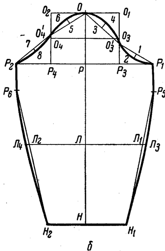
153-rasm. Sport va dam olish uchun mo'ljallangan jaketning konstruksiyasi
