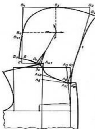
84-rasm. Kapyushon konstruksiya chizmasi
