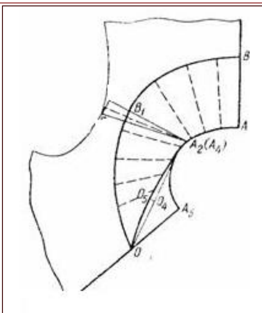
74-rasm. Kokilye yoqaning konstruksiya chizmasi
