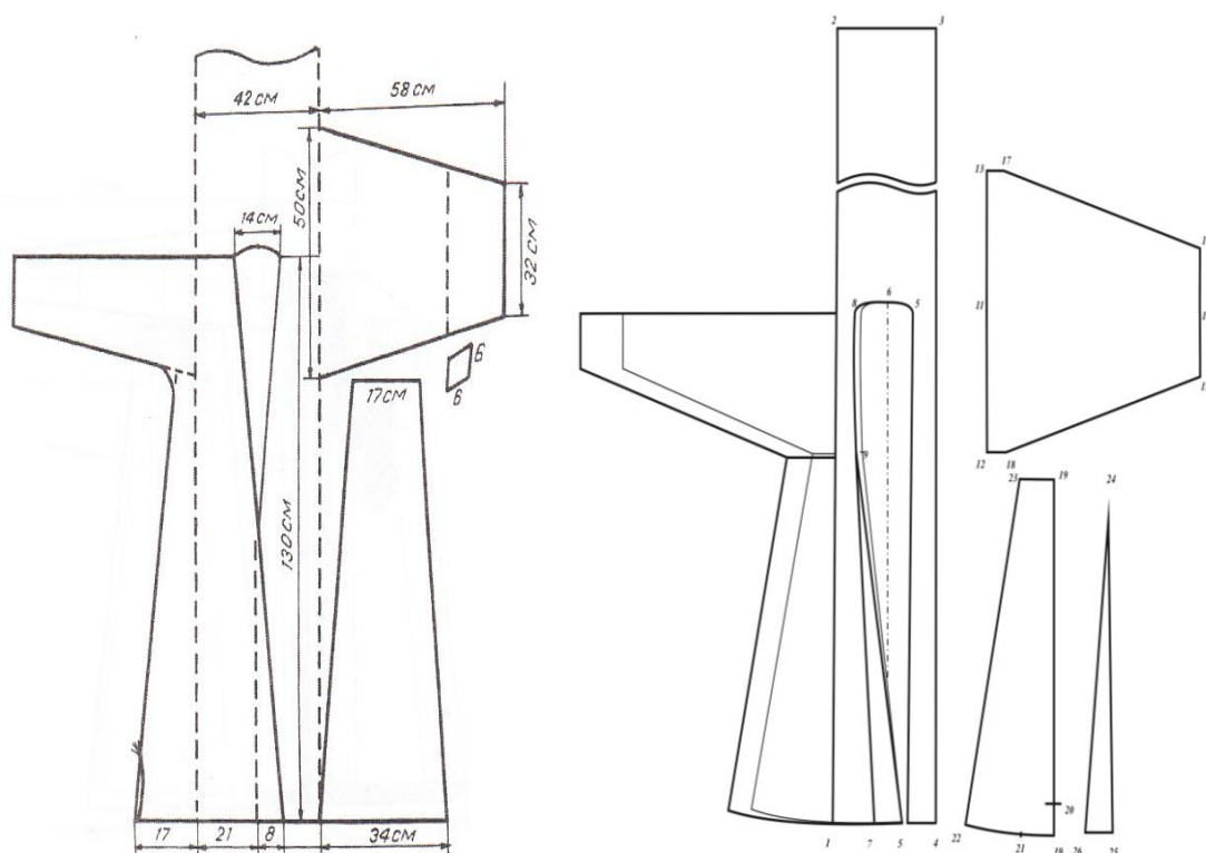
177-rasm. Ayollarning an'anaviylik buxorcha "peshkurtali" milliy ko'ylagi va lozimi
