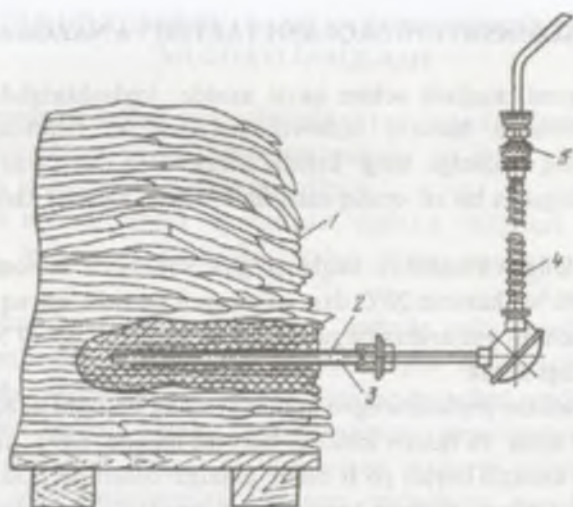
67-rasm. Qarshilik termometrini taxlovda joylashtirish tasviri: 1-taxlov; 2-himoyalovchi gilza; 3-qarshilik termometri; 4-shlangli chiqish yo'li; 5-shtepselli ajratma.
