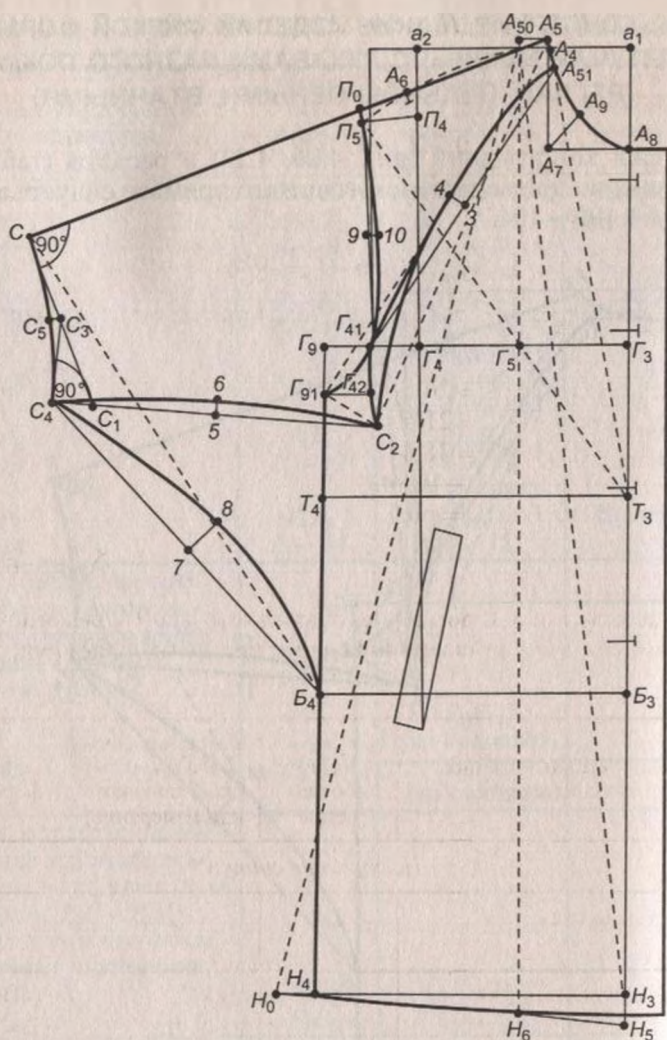
Рис. 4.27. Чертеж конструкции женского пальто прямого силуэта (полочка) с рукавами разного покроя (реглан, цельнокроеными, втачными)
