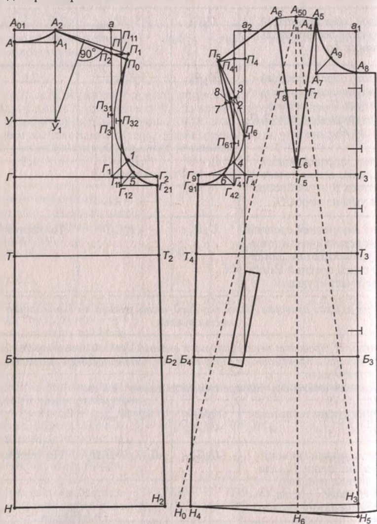
Рис. 4.19. Чертеж конструкции женского мехового пальто прямого силуэта (полочка и спинка) с углубленной проймой
