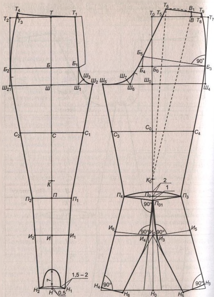
Рис. 5.27. Чертеж конструкции брѹк брѹдѹи с допѹлнительным членением нижней части
