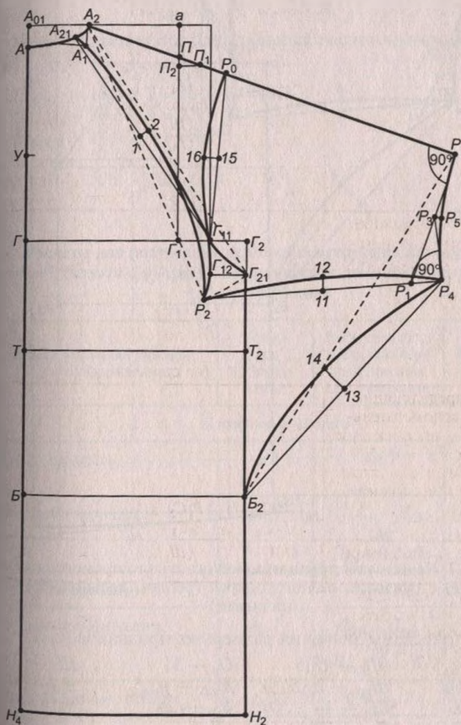
Рис. 4.26. Чертеж конструкции женского пальто прямого силуэта (спинка) с рукавами разного покроя (реглан, цельнокроеными, втачными)
