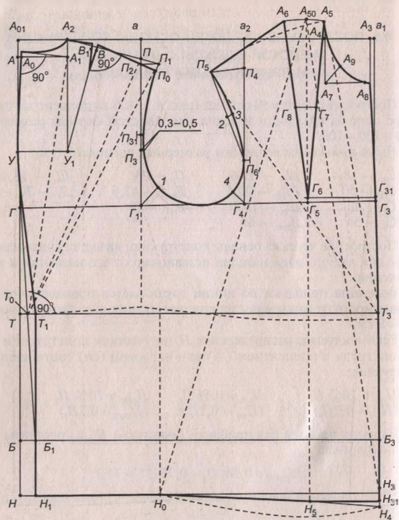
Рис. 4.1. Чертеж основы конструкции плечевой одежды
