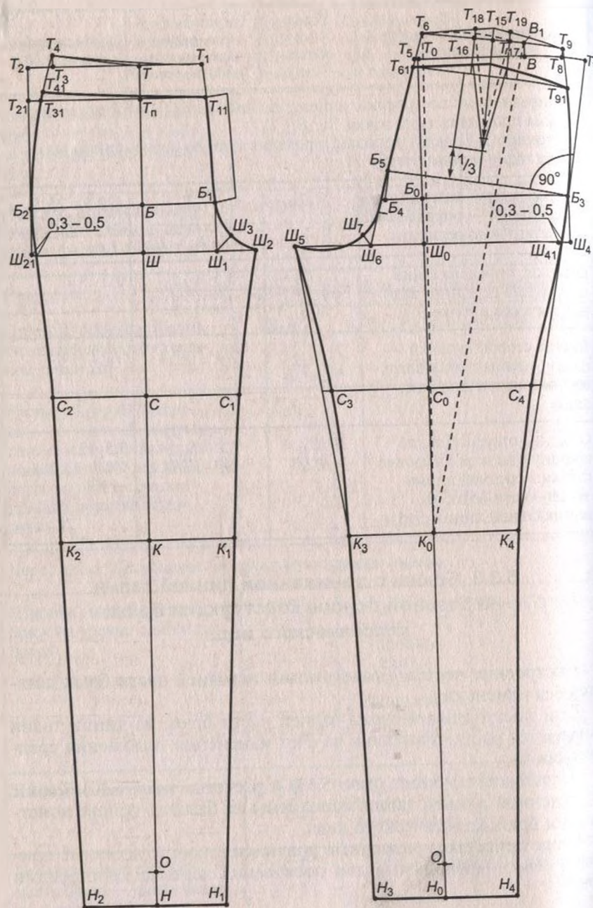
Рис. 5.13. Чертеж конструкции брюк с пониженной линией талии на базовой основе классических брюк
