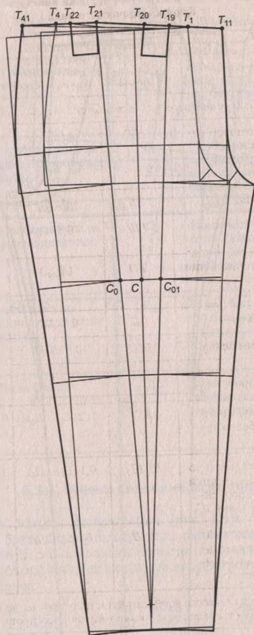
Рис. 5.11. Схема дополнительного расширения передней части брюк на уровне середины бедра
