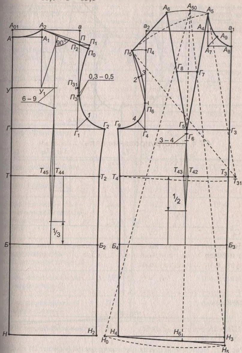
Рис. 4.34. Чертеж конструкции женского платья (вариант I) на фигуру с большим выступом живота
