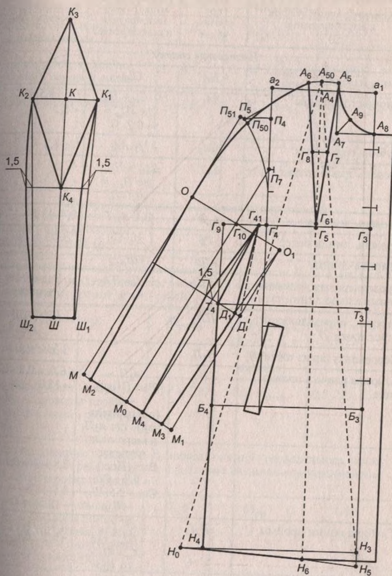
Рис. 4.13. Чертеж конструкции женского пальто прямого силуэта (полочка) с цельнокроеными рукавами и ластовицей, переходящей в рукав
