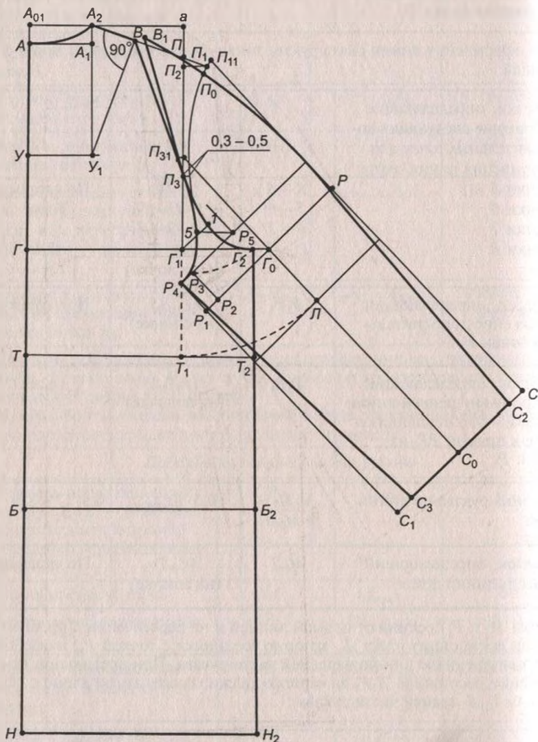
Рис. 4.17. Чертеж конструкции женского пальто прямого силуэта (спинка) с рукавами покрой полуреглан на базовой основе изделий с цельнокроеными рукавами
