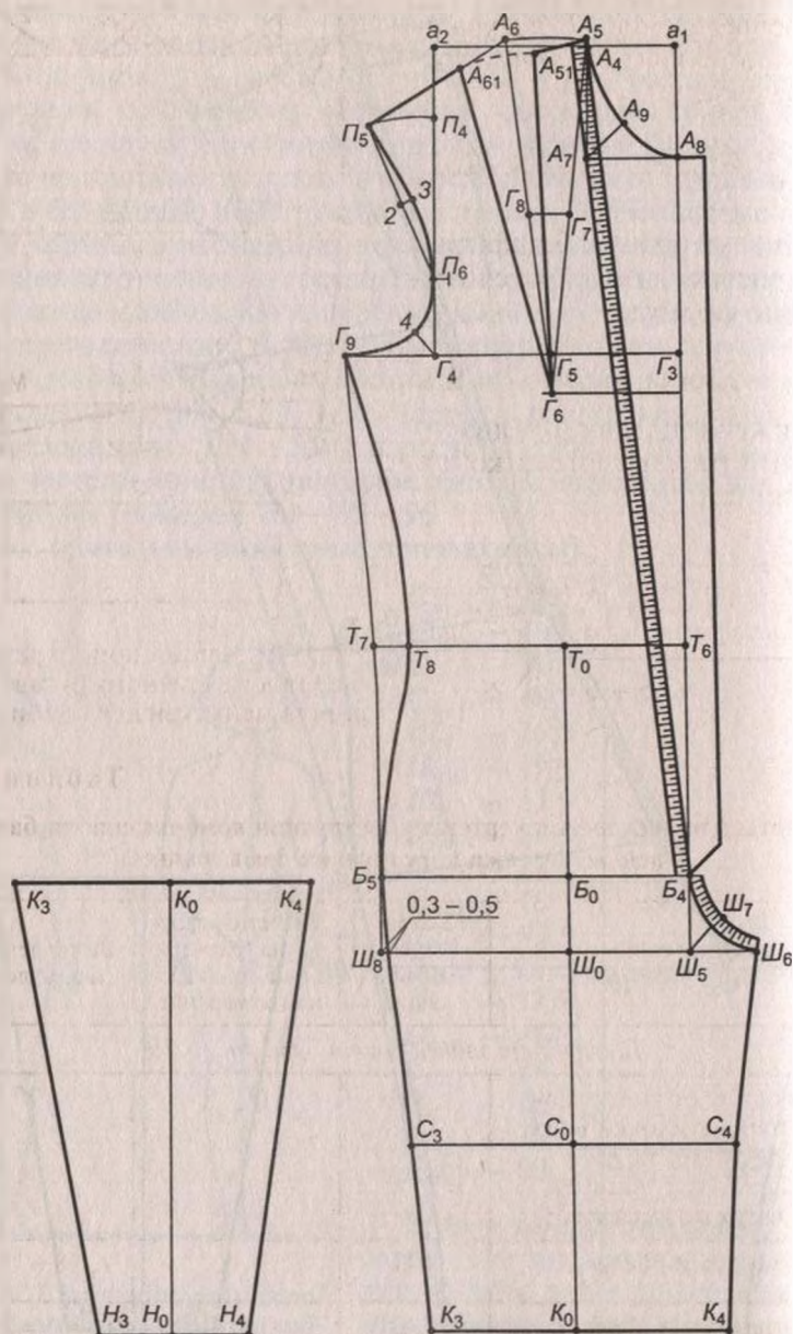
Рис. 5.20. Чертеж конструкции передней части комбинезона
