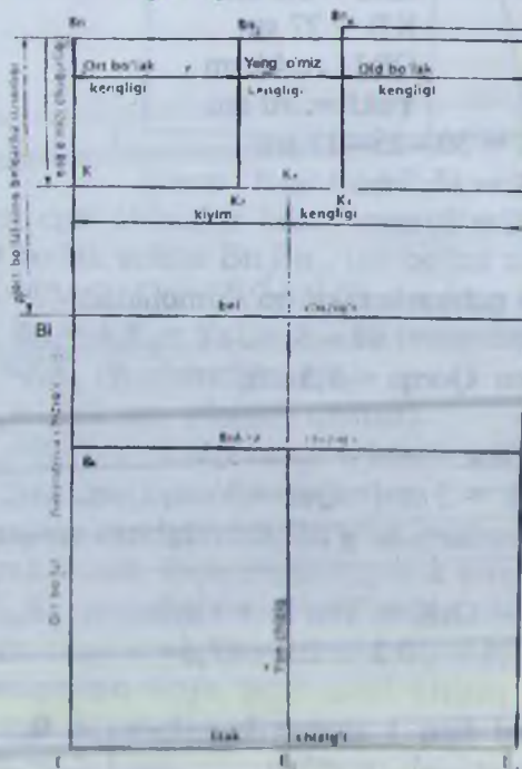
24-rasm. Ko'ylakning to'r qismi
