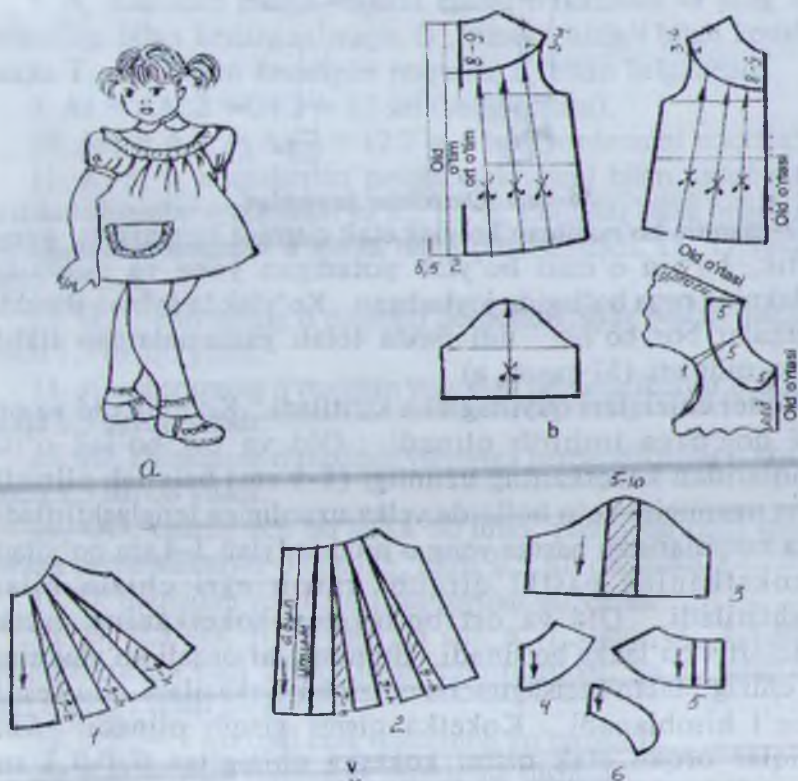
57-rasm. Qiz bolalar ko'ylagini modellashtirish
