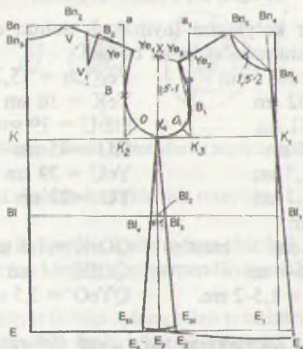
60-rasm. O'g'il bolalar ko'ylagining chizmasi
