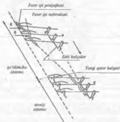
88-rasm. Futer to'qimasida nabroska hosil qilish tartibi.
