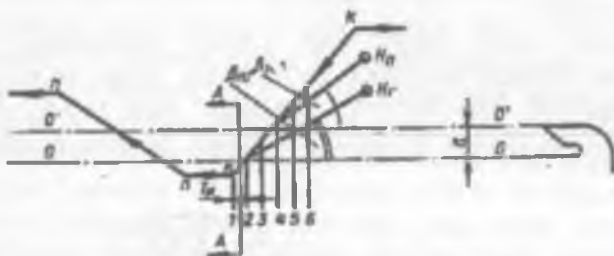
84-rasm. Igna ilgagi eng yuqori nuqtasining harakat trayektoriyasi.
