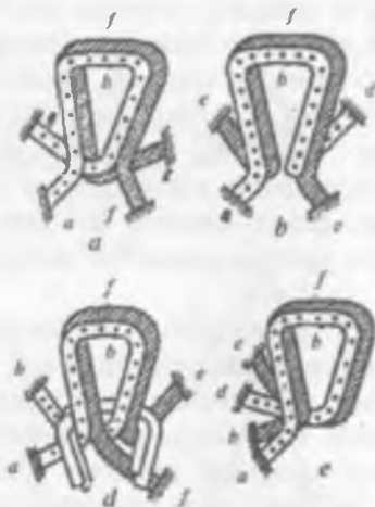
70-rasm. Yopqichli tanda trikotaj to'qimasi halqa tuzilishi.
