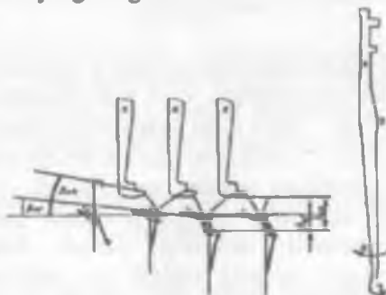
85-rasm. Ikki ignadonli avtomatda tukli halqalarni hosil qilish sxemasi.
