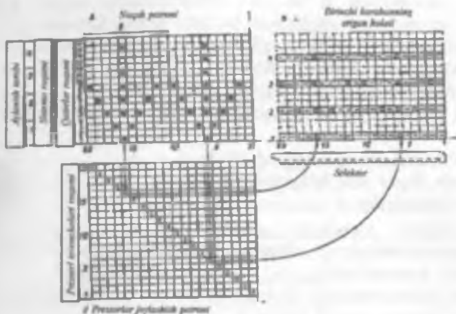
45-rasm. Ajur naqshi uchun sanoq-programma qurilmasining grafik hisoblash sxemasi.
