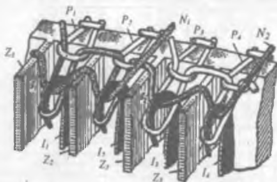
54-rasm. Kiper trikotaj to'qimasini olishda egish operatsiyasi.
