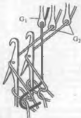
105-rasm. Arqoq trikotajini to'qishda arqoq ipini qo'yish.
