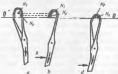
72-rasm. Igna ilgagi ostida iplar o'rmini almashtirish sxemasi.
