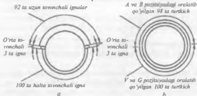
118-rasm. NOR paypoq to'quv avtomati ignalari, turtkichlari va platinalari.
