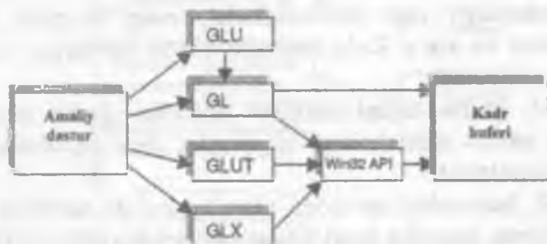
3.1-rasm. OpenGL kutubxonalarining tashkil etilishi.
