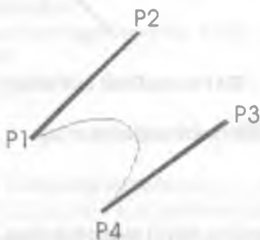
2.12-rasm. Beze egri chizig'i.
