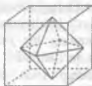
2.4-rasm. Oktaedr.
