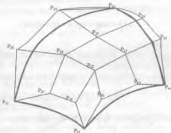
2.14-rasm. Beze splayn sirti.
