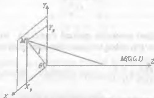
2.8-rasm. Qiya burchakli proeksiya.
