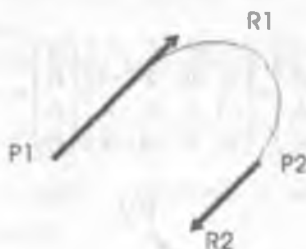
2.11-rasm. Ermit egri chizig'i.
