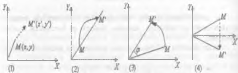
2.2-rasm. Tekislikdagi (ikki o'lchovli) almashtirishlar.
