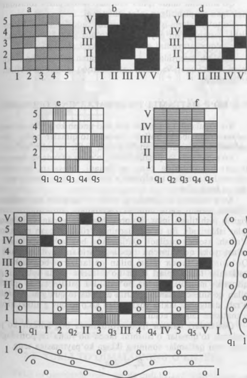
7.9-rasm. Sarja 4/I asosida qo'shimcha tandali ikki yarim qatlamli to'qima o'rilishining tasviri va tuzish bosqichlari.
