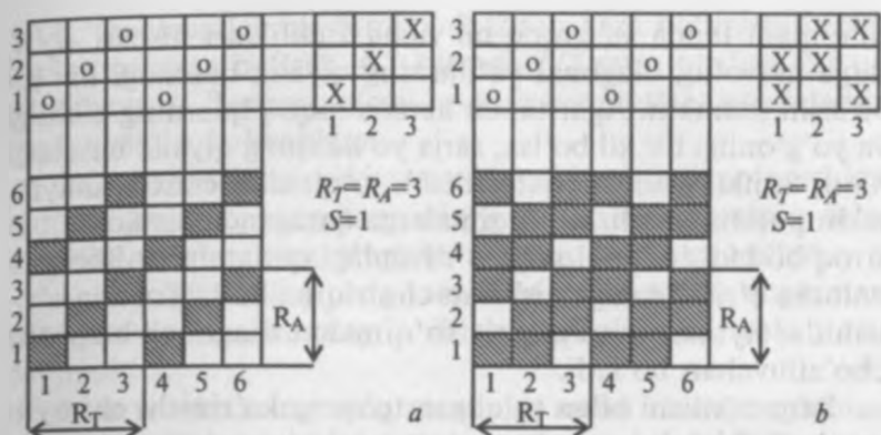
4.6-rasm. Sarja o'rilishini to'liq taxtlash dasturi.
