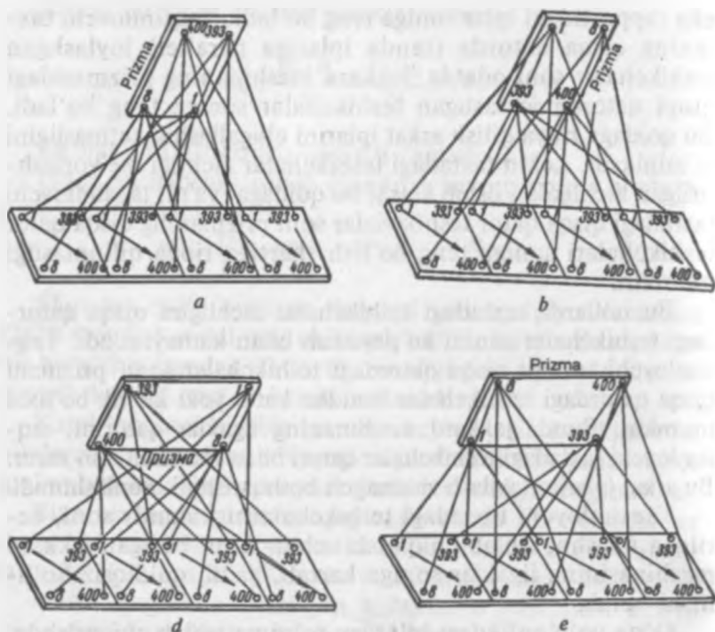
8.2-rasm. Prizmani tanda iplari va jakkard mashinasiga nisbatan joylashishi.
