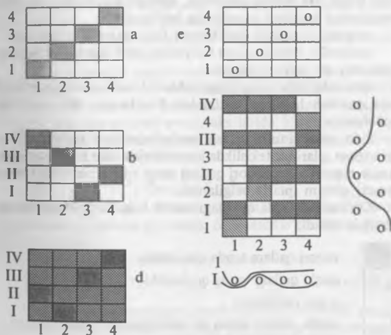
7.2-rasm. 1/3 va to'rt shodali satin asosida ikki tomonli qo'shimcha arqoqli bir yarim qatlamli to'qima o'rilishini taxtlash dasturi. a — yuqori qatlam sirt o'rilish tasviri; b — pastki qatlam sirt o'rilish tasviri; d — pastki qatlam ichki o'rilish tasviri; e — o'rilishni taxtlash dasturi.
