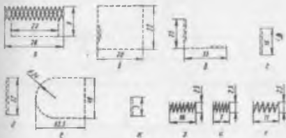
Рис. 69. Виды строчек, выполняемых на машине 820 кл.
