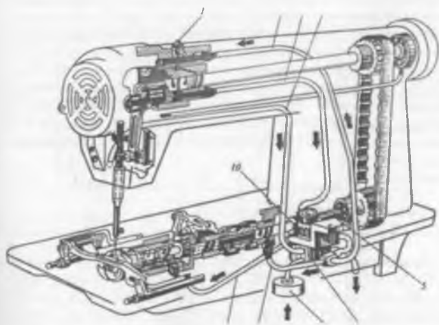
Рис. 28. Схема централизованной системы смазывания механизмов
