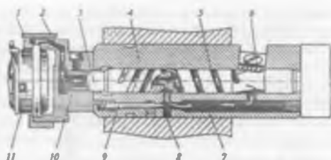
Рис. 34. Схема системы смазывания деталей в механизме челнока.
