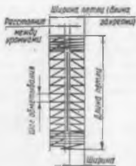
Рис. 79. Изготовление петли на машине 25—1 кл.
