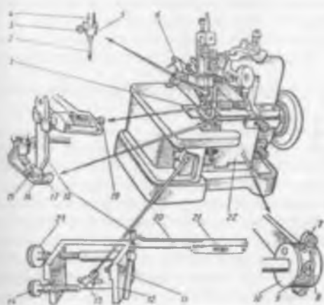
Рис. 64. Внешний вид машины 51 кл.
