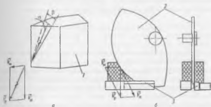
Рис. 14. Схемы раскроя ткани способами пидления с использованием пластинчатого ножа и комбинированным с использованием дискового ножа
