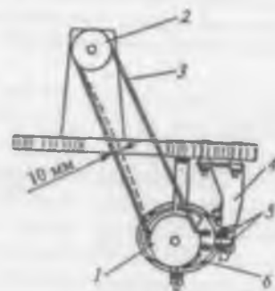
Рис.3. Схема установки электропривода на промышленном столе
