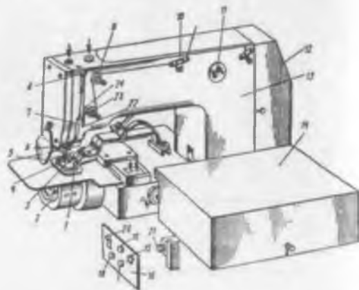
Рис. 68. Внешний вид машины 820 кл.
