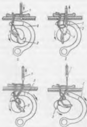
Рис. 72. Образование однопоточного цепного переплетения с помощью колеблющегося отводчика в машине 1095 кл.
