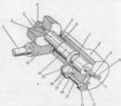
Рис.30. Схема устройства для намотки челночной нитки
