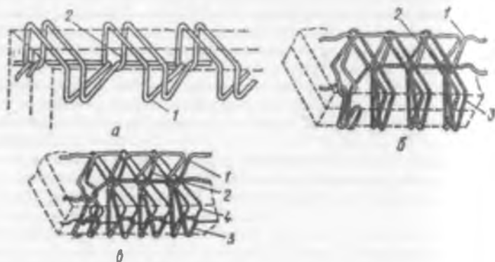
Рис. 60. Виды обметочных строчек
