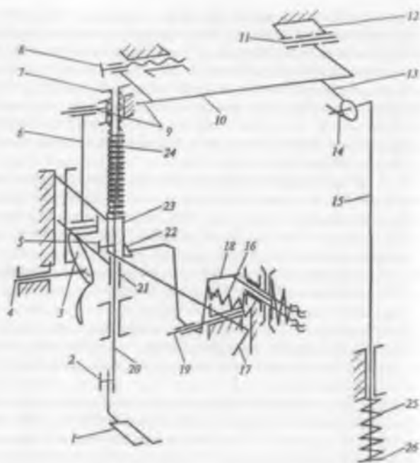
Рис.33. Кинематическая схема узла прижимной лапки.
