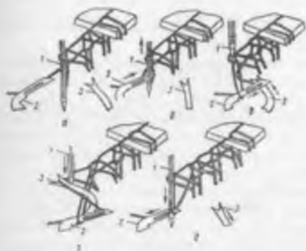
Рис. 61. Образование двух ниточного цепного обметочного переплетения
