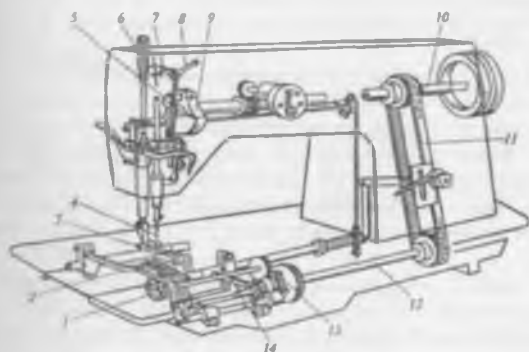
Рис.31. Схема машины класса 1022М
