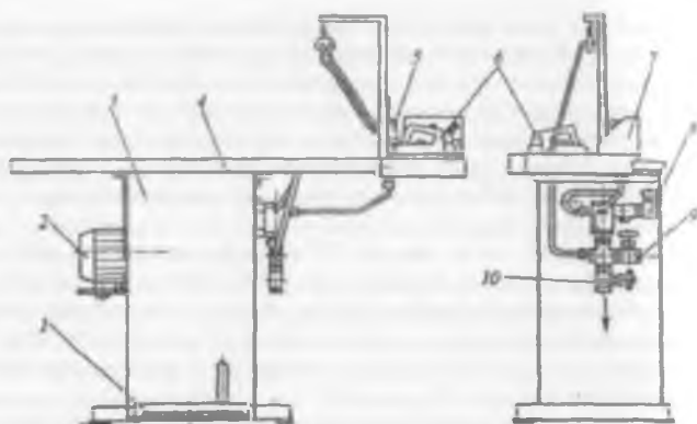
Рис. 92. Утюжильный стол модели СУ—М—1
