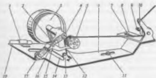
Рис.23. Моталка челночной нитки на шпульку к швейной машине
