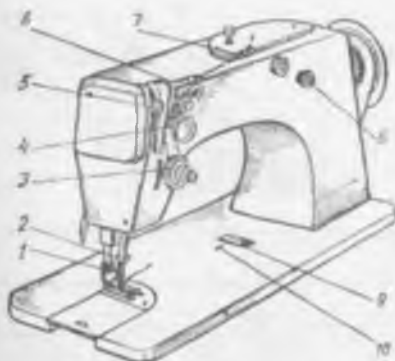
Рисунок. 45 Внешний вид машины.
