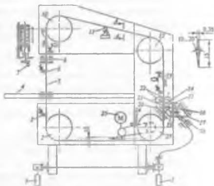
Рис. 15. Кинематическая схема стационарной раскройной машины
