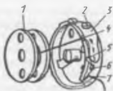
Рис. 55. Заправка нижней нитки в машине 335 кл.
