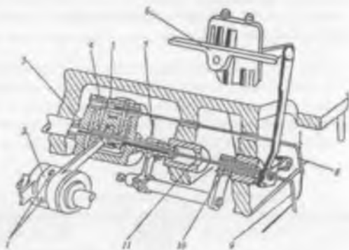
Рис.39. Схема установки рукоятки регулятора длины стежка по калибрам для швейных машин конструктивно-унифицированных рядов 31 и 131
