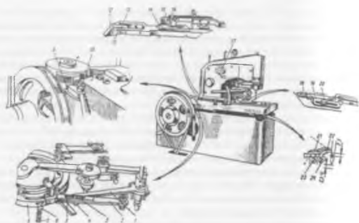
Рис. 85 Выполнение основных регулировок на машине 73401—РЗ кл.
