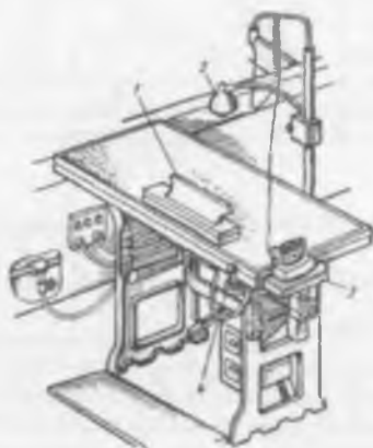
Рис 91 Рабочее место утюжильщицы
