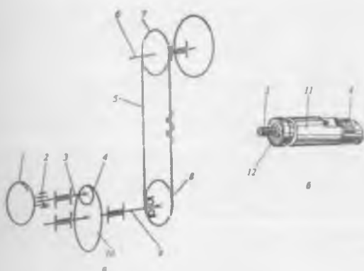
Рис. 25. Челнок к швейной машине класса 97—А
