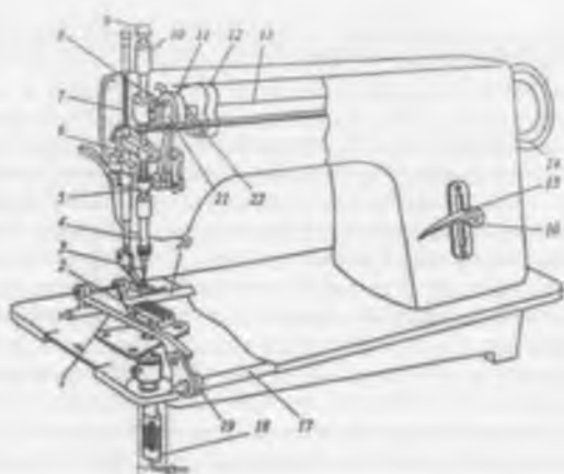
Рис. 87. Безниточная швейная машина БШМ—2.
