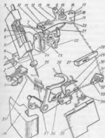
Рис. 63. Заправка ниток в машине 51 кл.
