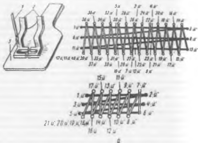
Рис. 65. Изготовление малой (а) и большой (б) закрепок
