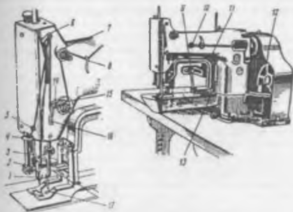
Рис. 66. Внешний вид машины 220—М кл.
