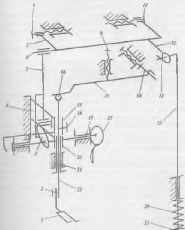
Рис 27 Кинематическая схема узла подъема прижимной лапки
