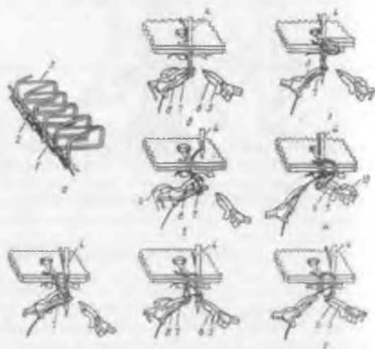
Рис. 83. Процесс образования стежка на машине 73401—РЗ кл.
