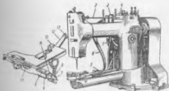
Рис. 75. Внешний вид машины 59—А кл.
