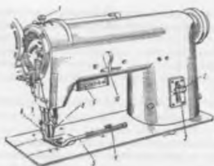
Рис 42 Внешний вид машины 297 кл
