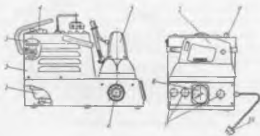
Рис.89. Парогенератор марки МП—4
