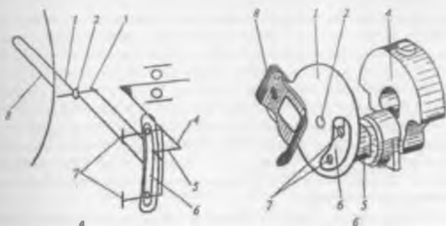
Рис. 24. Нитепритягиватель ротационного типа
