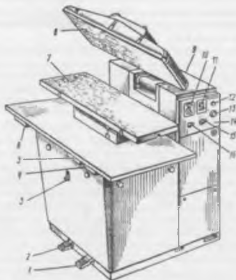
Рис. 93. Пресс ППУ—2
