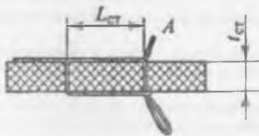
Рис. 44. Однострочный цепной стежок типа 10I
