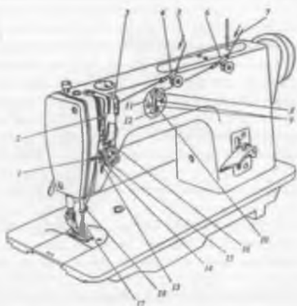
Рис. 29. Схема заправки игольной нитки
