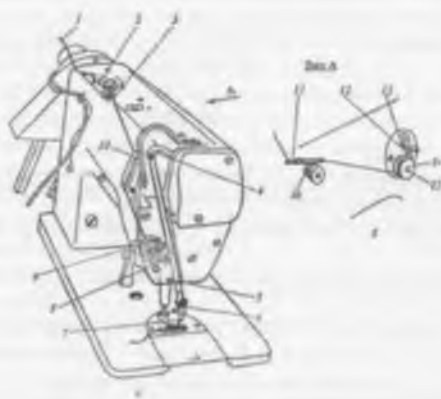
Рис.35 Общий вид швейной машины класса 31—12+3, схема заправки игольной нитки при образовании строчки (а) и челночной нитки при ее наматывании на шпульку (б)
