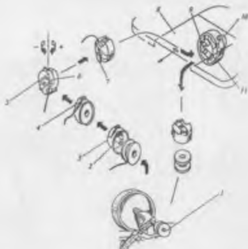
Рис. 22. Схема последовательной перезаправки челночной нитки.
