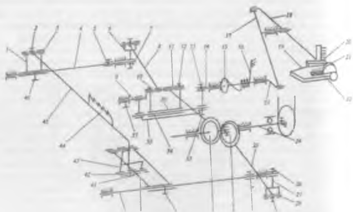
Рис. 32. Кинематическая схема механизма перемещения зубчатой рейки.
