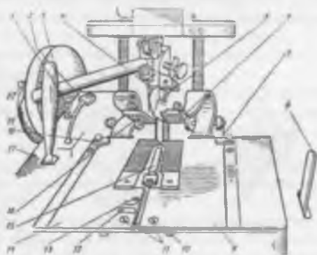
Рис.81. Платформа машины 73401—РЗ кл.
