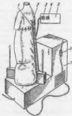
Рис. 96. Паровоздушный манекен МПВУ
