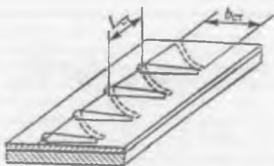
Рис. 46. Однониточный потайной цепной стежок
