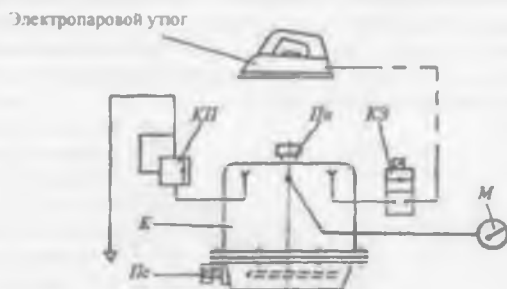
Рис.90. Схема парогенератора марки МП—4
