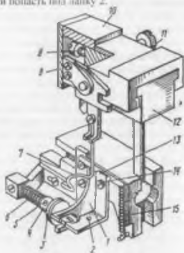
Рис. 73. Держатель пуговицы машины 1595 кл.
