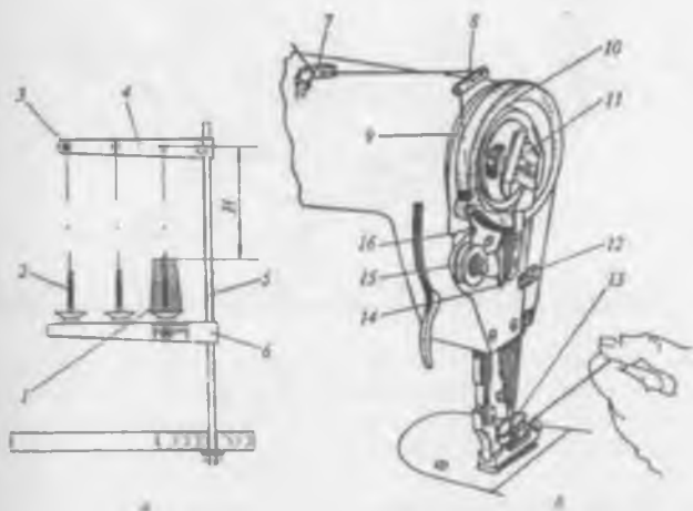
Рис. 21 Схема заправки игольной нитки.
