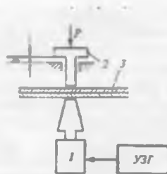
Рис 86 Блок-схема ультразвуковой сварки текстильных материалов
