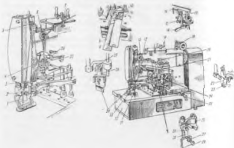
Рис. 80. Выполнение основных регулировок в машине 25—1 кл.
