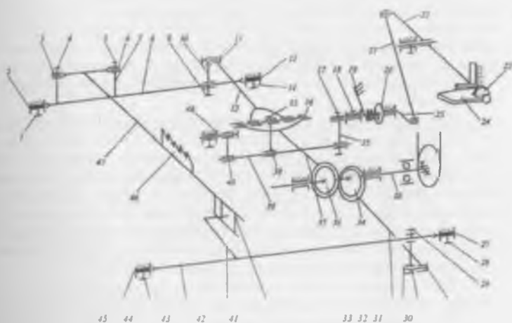
Рис. 26. Кинематическая схема механизма перемещения рейки
