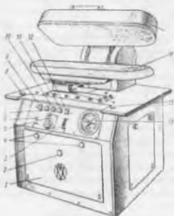
Рис. 94. Пресс Cs—311AK
