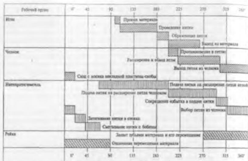
Рис.20. Циклограмма работы машины
