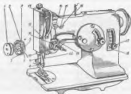
Рис. 52. Внешний вид машины 26 кл.
