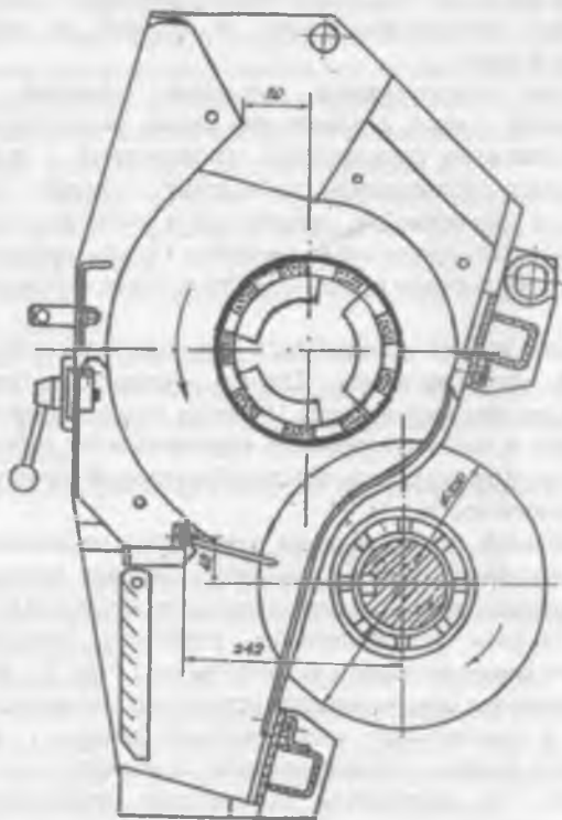
Рис 3.16. Рабочая камера с дополнительным семявыводящим устройством (Патент РУз. №4372).
