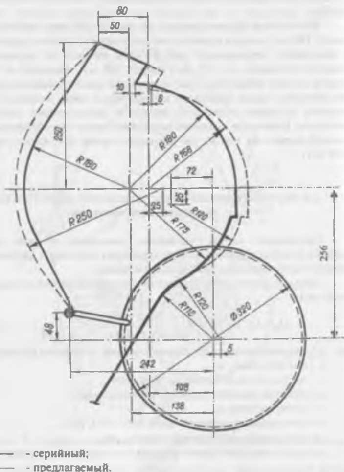
Рис. 2.8. Профиль предлагаемой - рациональной формы рабочей камеры.
