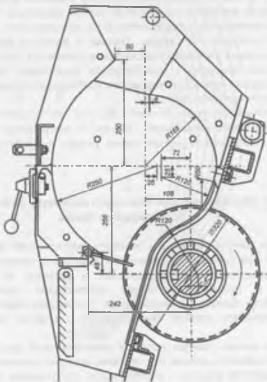
Рис.2.7. Профиль существующей рабочей камеры пильного джина.
