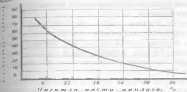
51-Расм. Пахта намлигини ускунанинг тозалаш самарадорлигига таъсири графиги
