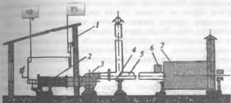
40-расм. ТТ-1,5 иссиқлик генератори билан таъминланган чигитли пахтани қуритиш жараёни схемаси.
