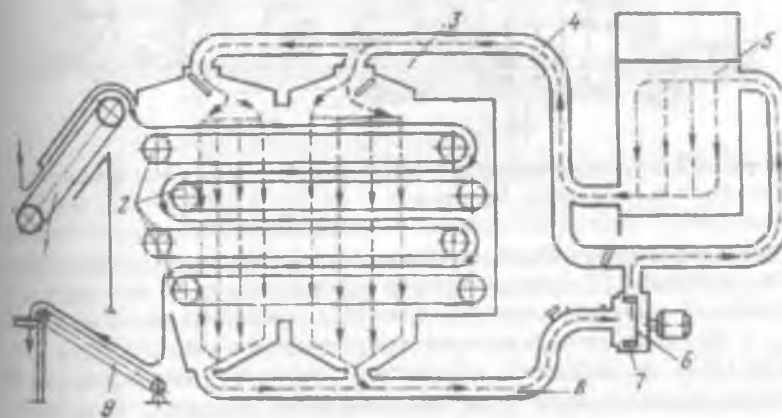
130-расм. КСК-4,5 қўриитиш дастгоҳи схемаси
