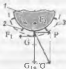
50-расм. Барабан қозигининг пахта бўлакчасига таъсир қилиш схемаси 1-қозикчали барабан; 2-қозикча; 3-тўрли юза; F_1 -чигитли пахта бўлағига тўрли сиртга ишқатаниш кучи, G_1 -марказдан қочма куч; G -чигитли пахта бўлағининг оғирлиги; F_2 -чигитли пахта бўлағининг қозик сиртига ишқатаниш кучи; P -камера ичидаги ҳаво оқимининг қаршилиги.
