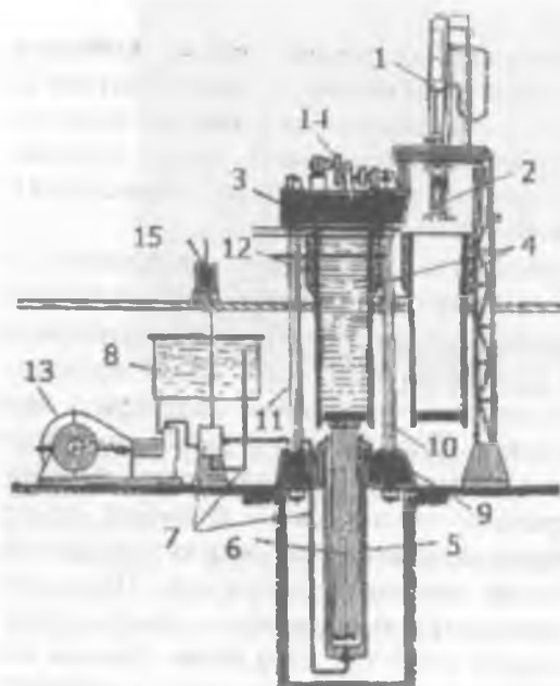
106-расм. К20.801 гидроаппарат шиббалагичнинг умумий қўриниши. 1,5-гидроцилиндр; 2-шиббалаги плитаси; 3-кросс-траверс; 4-пресслаш яшиги; 6-поршень; 7-суюқлик узатувчи қувур; 8-суюқлик баки; 9-пастки траверс; 10,11-пресснинг ён колонналари; 12-пресс қўтиси эшиги; 13-гидронасослар системи; 14-пресс камерасини ҳаракатга келтирувчи электр юритма; 15-бошқарув қўрилмаси.
