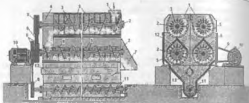
56- расм. 6А-12М русумли шнекли пахта тозалаш ускунасининг схемаси 1- шахта; 2- айлантирувчи шнек; 3,6-валдаги парралар; 4-вертикал шахта; 5-тўрли юза; 7-тозаланган пахтани тушириш нови; 8- шкивлар; 9- тасма; узатма; 10- электродвигател; 11-ифлослик шег; 12-тўсиқ; 13-чангли ҳавони узатиш қубури
