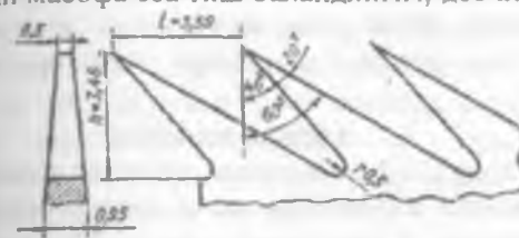
75-расм. Жин аррасининг ўлчамлари
