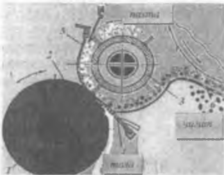
83-расм. Чигитни қаттиқ уриш қисми
