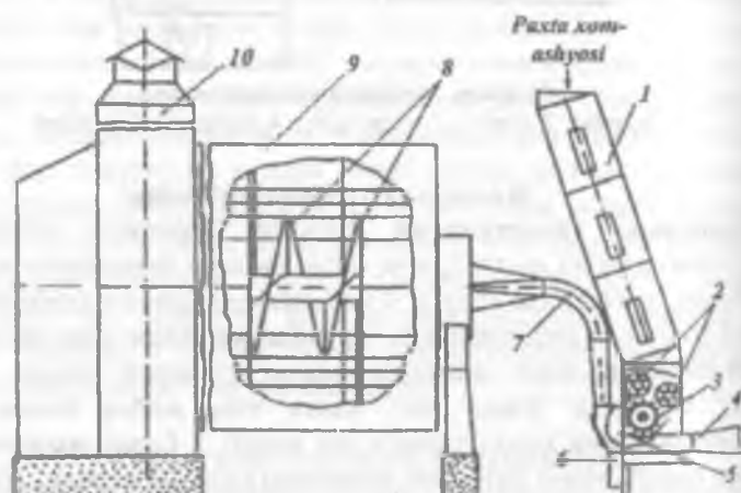
48-расм. Титувчи қисмли ва тўпловчи сизимли ПРС русумли қуритгич таъминлагичи 1-қия тўпловчи шахта, 2- таъминловчи валиклар, 3-титувчи барабан, 4-иссиқ ҳаво қувури, 5-турли юза, 6-огир ифлос аразашмаларни ушлаб қолувчи қувур, 7-иссиқ ҳаво билан аразашган пахта ҳаракатланувчи қувур, 8-шнек, 9-қуритиш барабани, 10-мури.
