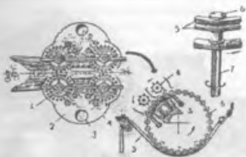
7-Расм. Ишчи апаратынинг асосий схемаси.
