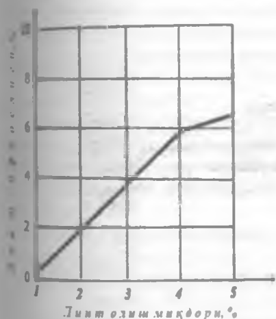
104-расм. Линт ифлослигининг линт олиш миқдориға таъсири
