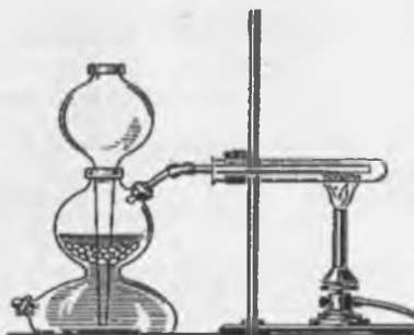
18.1-rasm. CuO ni vodorod yordamida qaytarish.
