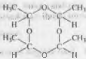
metaldegid
