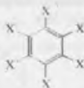
geksa-X-benzol
