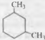
1,3-dimetilsiklogeksan
