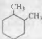
1,2-dimetilsiklogeksan
