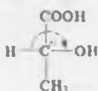
D-sut kislotasi
