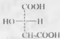
(S)-(-)-olma kislota
