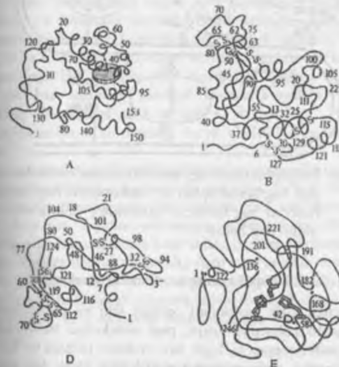
37-rasm. Mioglobin (A), lizotsim (B), ribonukleaza (D) va ximotripsinogen (E) oqsillarining uchlamchi strukturasi
