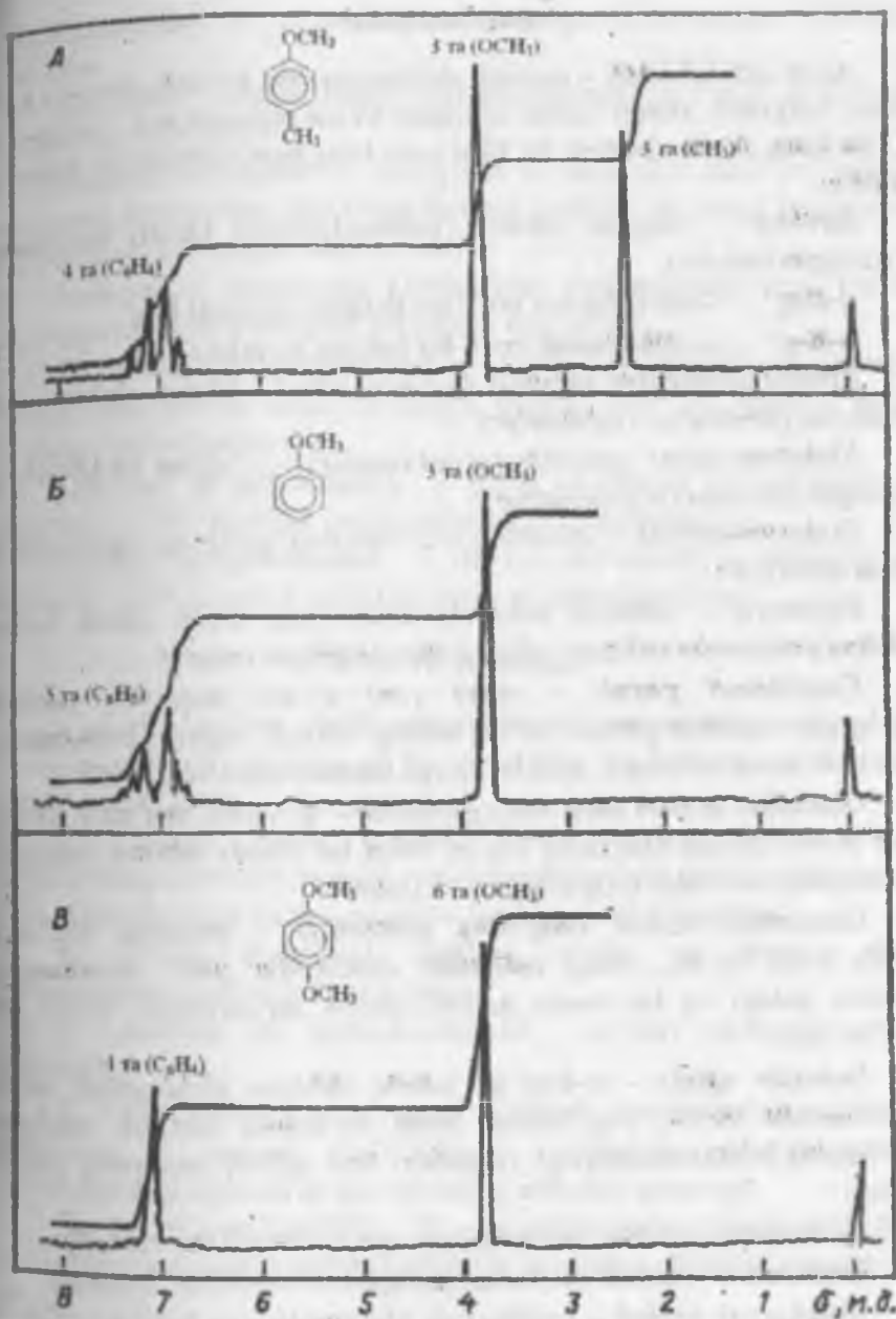
20-rasm. 1-metoksi-4-metilbenzol (A), metoksibenzol (B) va 1,4-dime- toksibenzol (V) ning PMR spektrlari.
