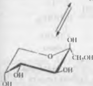
\beta -D-fruktopiranoza
