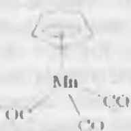
siklopentadiyenil- marganetstrikarbonili
