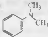
N, N-dimetilanilin
