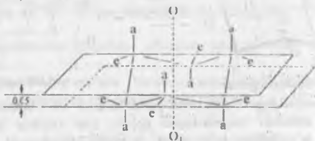
41- rasm. Siklogeksanning kreslo konformatsiyasi
