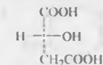
(R)-(+)-olma kislota
