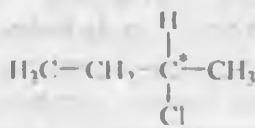
2-xlorbutan
