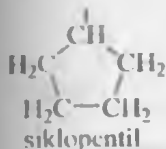
siklopentil
