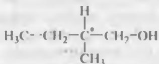
2-metilbutanol-1
