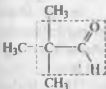
trimetilsirka aldegid
