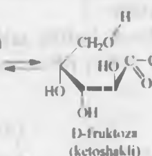
D-fruktoza (ketoshakli)
