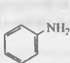
anilin
