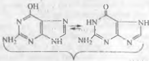
guanin (2-amino-6-gidroksipurin)
