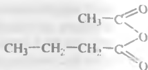
sirka-moy ангидрид
