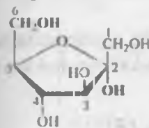
\alpha -D-fruktofuranosa
