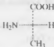
L-alanin
