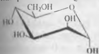
\alpha -D(+)-mannopiranoza
