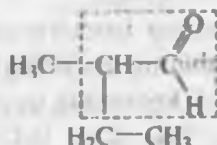
etilmetilsirka aldegid
