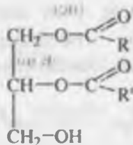
1,2-diglitserid (1,2-diatsilglitserin)
