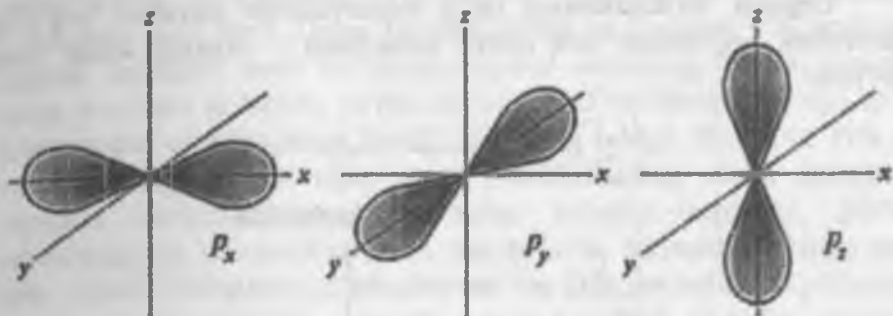
2-rasm. Uglerodning p-atom orbitallari.
