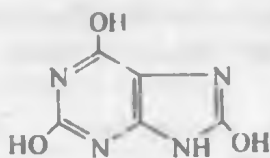
2,6,8-trigidroksipurin
