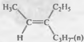
(E)-3-etil-2-geksen
