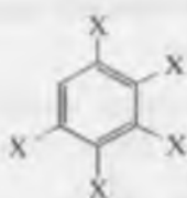
penta-X-benzol
