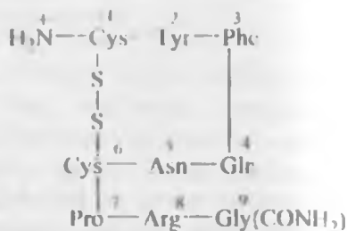
Vazopressin
