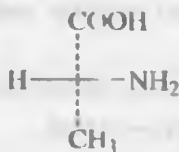
D-alanin
