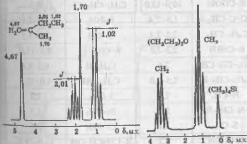
19-rasm. Dietil efirining PMR spektri
