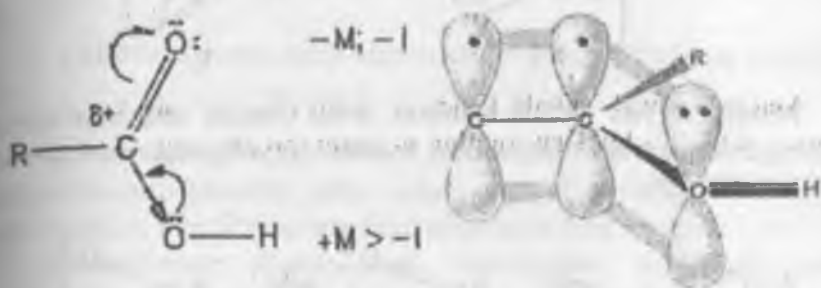
32-rasm. Karboksil guruhining elektron tuzilishi va p,π-tutashish.
