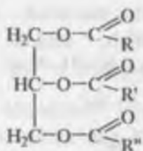
triglitserid (triatsilglitserin)
