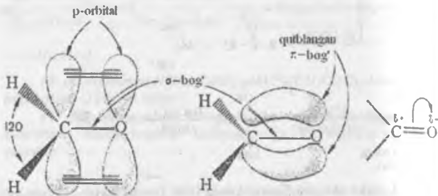
31-rasm. Chumoli aldegid molekulasiining elektron tuzilishi
