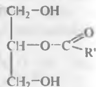
2-monoglitserid (2-atsilglitserin)
