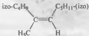
(Z)-2,4,8-trimetil-4-nonen
