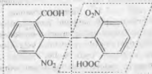
26-rasm. o,o'-dinitrodifenikislota atropizomeri.
