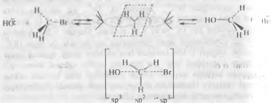
28- rasin. O'tish holatining hosil bo'lish sxemasi.
