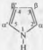
pirrol
