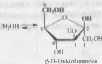
\beta -D-fruktofuranosa
