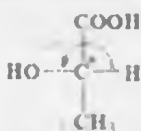
L-sut kislotasi
