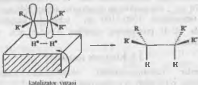
21-rasm. Geterogen katalitik reaksiyalarda vodorodning alkenlarga sin-birikish sxemasi
