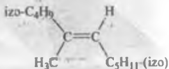
(E)-2,4,8-trimetil-4-nonen
