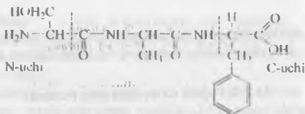
serilalanilfenilalanin (Ser-Ala-Phe)
