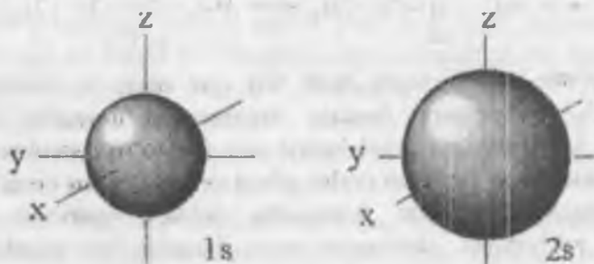
1-rasm. s-Orbital shakli.
