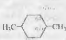
1,4-dimetilsiklogeksan
