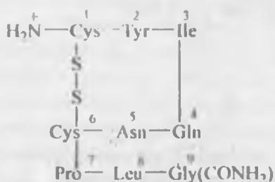
Oksitotsin
