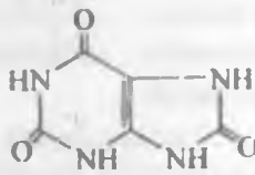
2,6,8-triketogeksagidropurin
