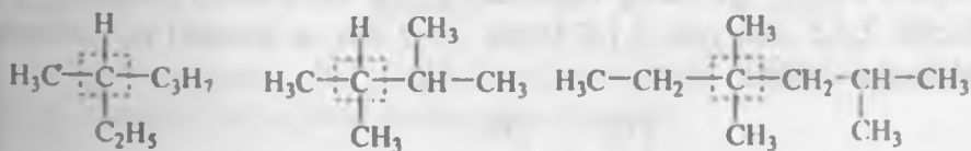
etilmetilpropilmetan
