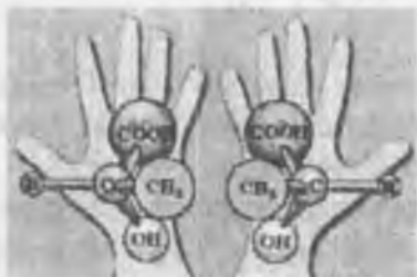
D-sut kislotasi
