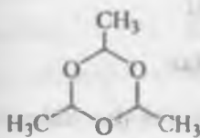
paraldegid
