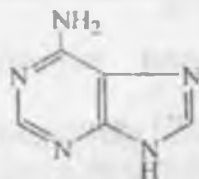
adenin (6-aminopurin)
