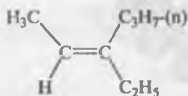
(Z)-3-etil-2-geksen
