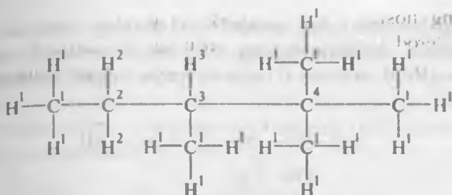
2,2,3-trimetilpentan
