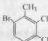
1-brom-2-metil- 3,4-dixlorbenzol
