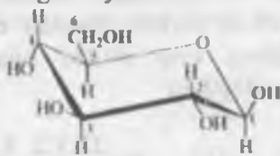
\beta -D-glyukopiranoza
