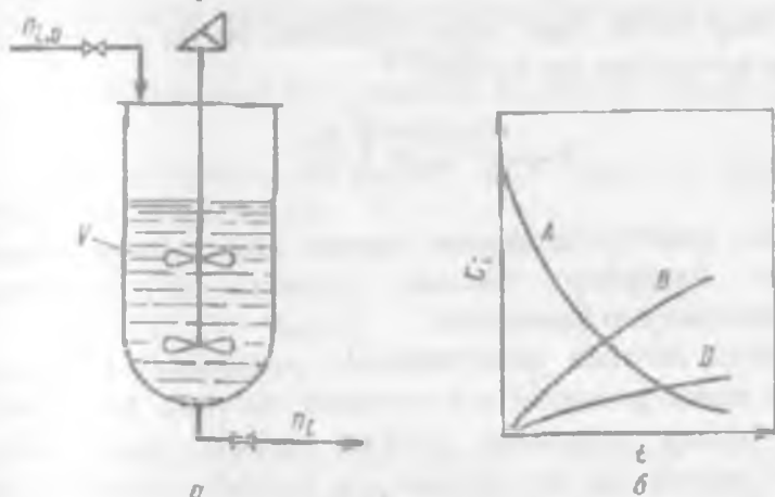
4.4-Rasm. Davriy ravishda ishlovchi ideal reaktorlar sxemasi va kinetik o'zgarishlar grafigi.
