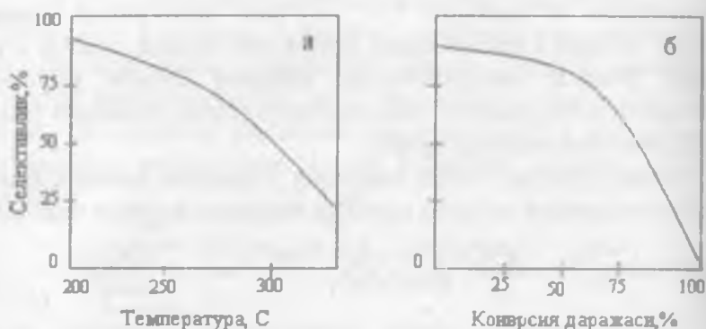
5.9-Rasm. Etilenni oksidlanish reaksiyasi selektivligini temperaturaga (a) va konversiya darajasiga (b) bog'liqligi.
