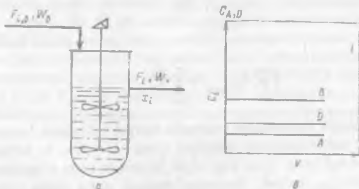
4.6-Rasm. Reaksiyon massani to'liq holda o'rin almashtirish mumkin bo'lgan reaktorlar
