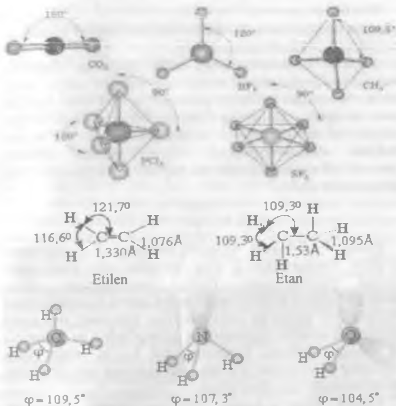
1.1-Rasm. Kimyoviy birikmalarda valent burchaklari
