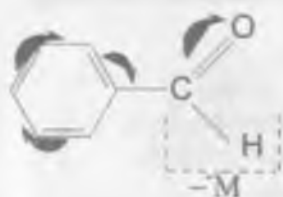
benzaldegid
