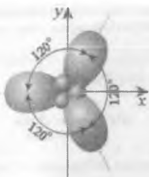
1.7-Rasm. Etilen molekulasida gibril orbitallarning hosil bo'lishi
