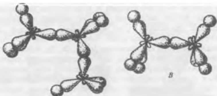
1.6-Rasm. Etil spirt A va metilamin B molekularining elektron tuzilishi
