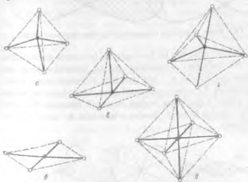
5.5–Rasm. O'zgaruvchan valentli metallarni ligandalar bilan hosil qilgan komplekslarini fazoviy joylashishi: a-tetraedr; b-kvadrat; v-tetragonal piramida; g-trigonai bipiramida; d-oktaedr.
