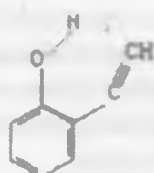
o-kresol
