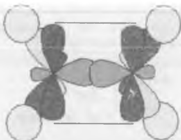
1.7-Rasm. Etilen molekulasida gibril orbitallarning hosil bo'lishi
