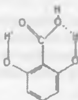
2,6-diglycidilbenzoic kislota
