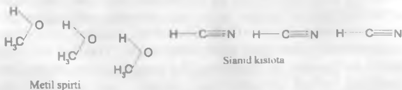
1.2-Rasm. Molekulararo vodorod bog'lar
