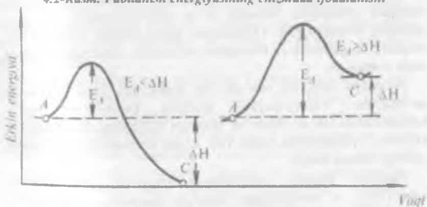
4.3-Rasm. Ekzotermik A va endotermik B reaksiyalarning faollanish energiyalari
