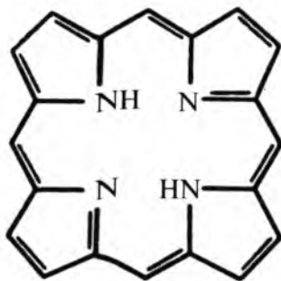
Porfirin
