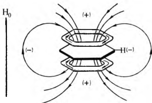
3.22-rasm. Aromatiklikni YaMR-spektroskopiya yordamida aniqlash.
