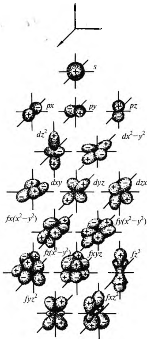
2.8-rasm. s , p , d , f -elektronlar bulutining shakllari va fazodagi yo'nalishlari. Musbat va manfiy belgilar shu sohalardagi to'liq funksiyaning ishorasini bildiradi.
