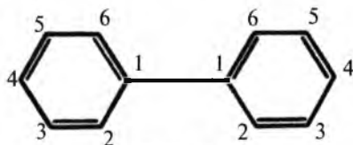
Difenil
