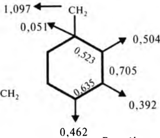
Benzil
