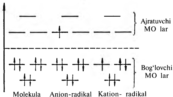
6.9-rasm. Benzol molekulasi, kation hamda anion radikallari MO larining energetik pog'onalari va elektronlar bilan to'lishi.
