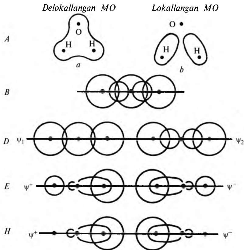
2.38-rasm. Delokallangan MO larni lokallangan MO larga aylantirish:
