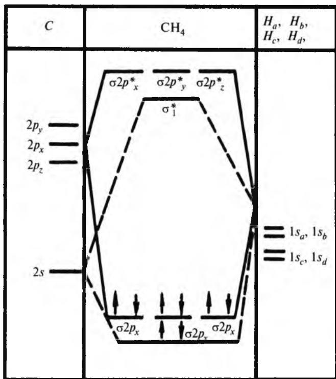
2.37-rasm. Metan molekulasining MO lari va ularning energetik pog'onalari.
