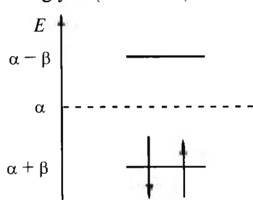
2.23-rasm. Etilen molekulasidagi bog'lovchi va ajratuvchi MO larning energetik pog'onolari. Ikkala \pi - elektron ham bog'lovchi MO da joylashgan.
