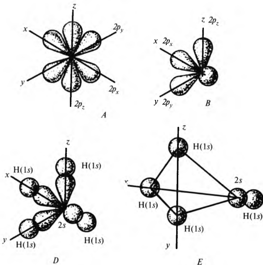
2.39-rasm. Uglerodning 2s va 2p va vodorodning 1s AO laridan metan molekulasining hosil bo'lishi. Qulaylik uchun B va D chizmalarda p -orbitalning yarmi ko'rsatilgan.
