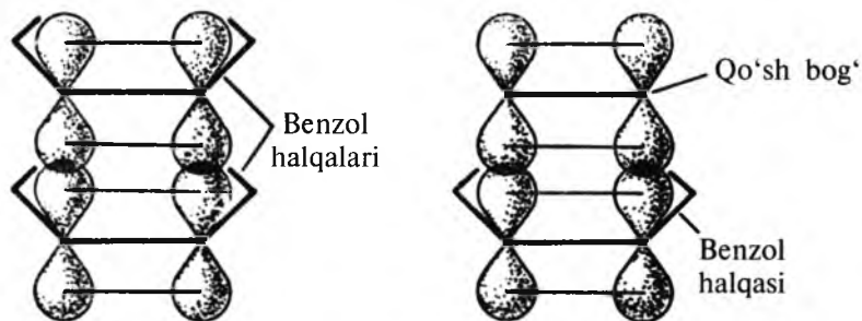
6.15-rasm. \pi -komplekslar hosil bo'lishidagi elektronlar bulutlari qoplanishining ko'rgazmali ifodalanishi.
