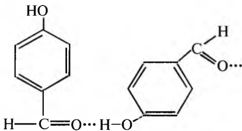
p- oksibenzaldegid
