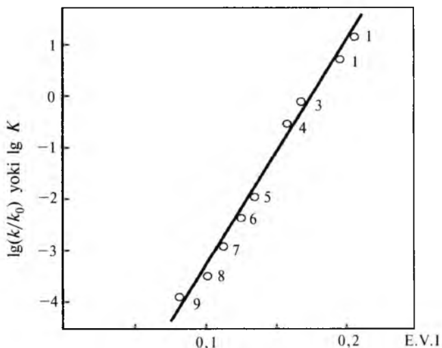
4.21-rasm. Aromatik radikallar va \text{CCl}_3 radikali o'rtasidagi reaksiyaning nisbiy tezlik konstantasi bilan erkin valentlik indeksleri orasidagi bog'lanish: 1—naftatsen; 2—antratsen; 3—stilben; 4—piren; 5—xrizen; 6—naftalin; 7—fenantren; 8—difenil; 9—benzol.
