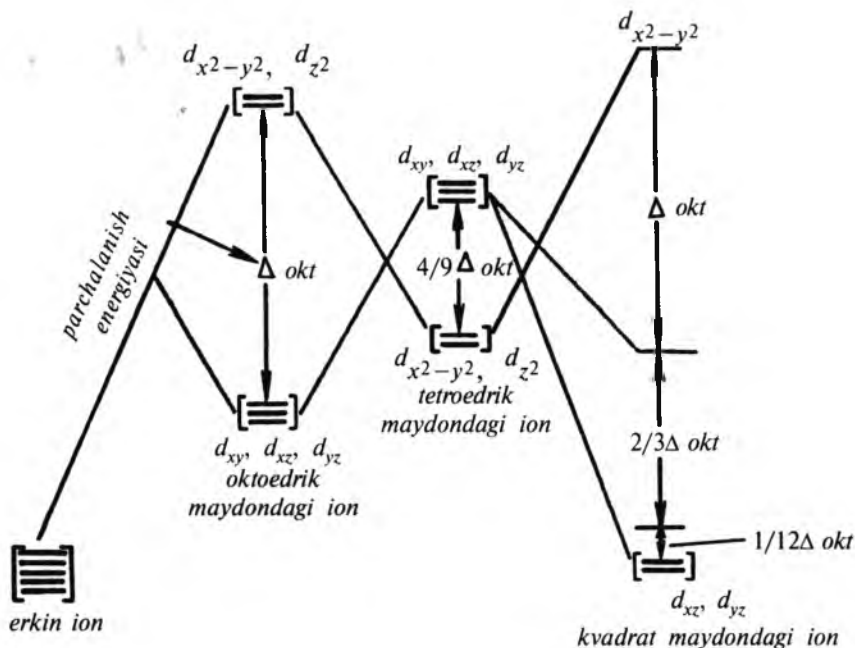
2.61-rasm. Oktaedrik, tetraedrik va kvadrat komplekslardagi metall d - orbitallarining energetik pog'onalar.
