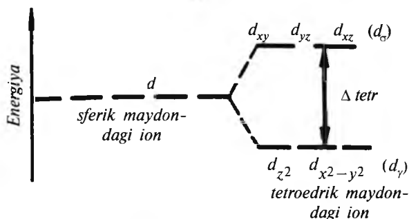
2.60-rasm. Metall d -orbitalari energetik pog'onalarining tetraedrik kompleks ligandlari maydonida ajralishi.
