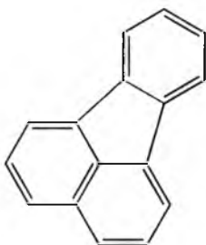
Fluoranten
