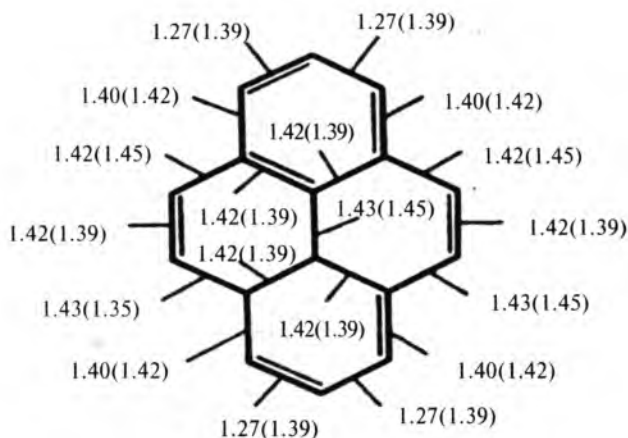
Piren
