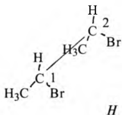
Eritro(sis)-2,3-dibrombutan
