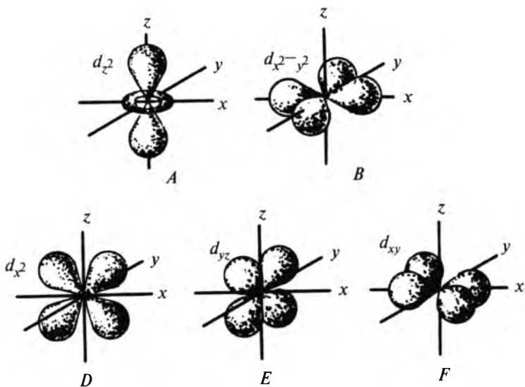
2.56- rasm. d -orbitallarning fazoda joylashishi.
