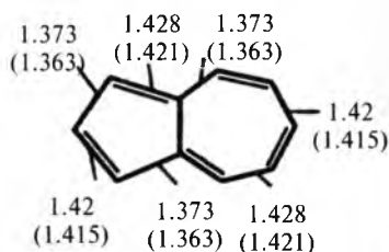
Azulen
