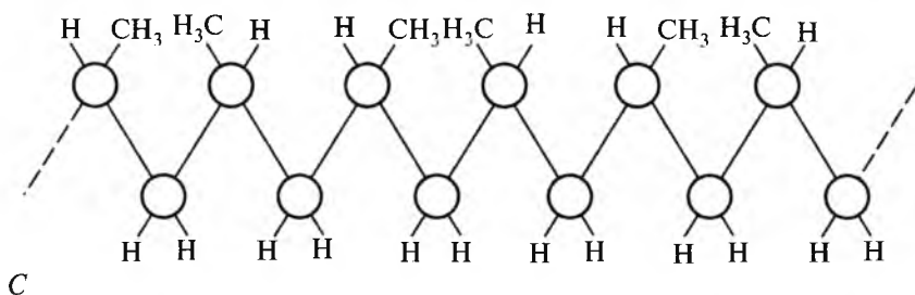
6.8-rasm. Ataktik A, izotaktik B va sindiotaktik C polipropilen.
