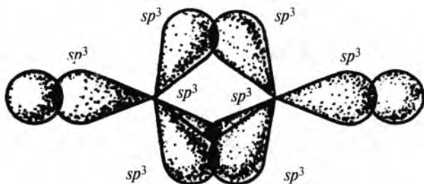
2.52-rasm. Atsetilen molekulasining Poling tavsiya etgan modeli.
