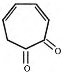
Keto-forma
