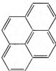
Piren
