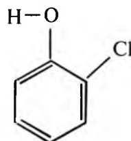
Trans-ortoxlorfenol
