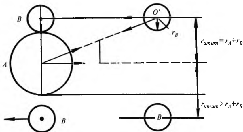
4.5-rasm. Molekulalar o'lchamlarining to'qnashishlar ehtimolligi bilan bog'liqligi.
