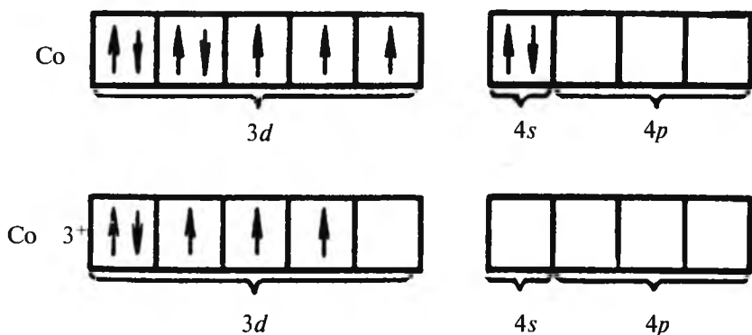
2.62-rasm. Oktedrik komplekslarda ligandlarning kuchsiz va kuchli maydoni ta'sirida metallning d -orbitallarida elektronlarning joylashishi.
