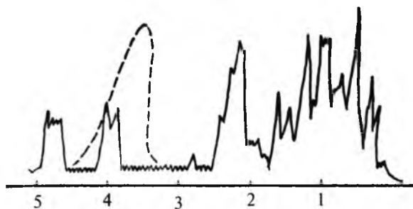
6.4-rasm. Norbornil fluoridning CCl_4 (tutash chiziq) va SbF_5 (punktir chiziq) da olingan YaMR spektrlari.
