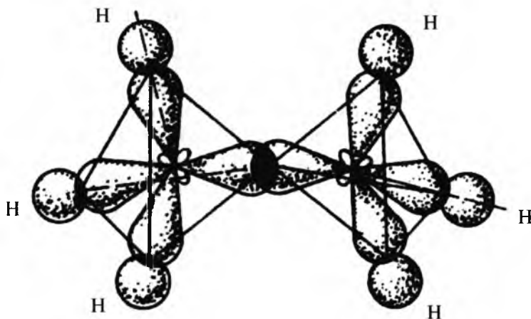
2.42-rasm. Etan molekulasining elektron tuzilishi.
