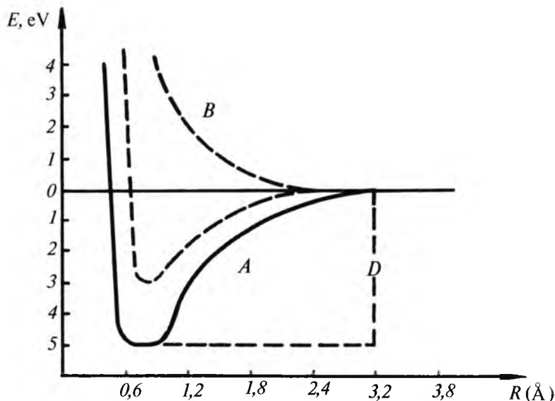
2.13-rasm. Simmetrik ( A ) va antisimmetrik ( B ) funksiyalar uchun energiyaning R ga bog'liqligi. (Uzuq chiziq bilan tajriba ma'lumotlari) ko'rsatilgan.
