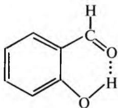
Salitsil aldegid
