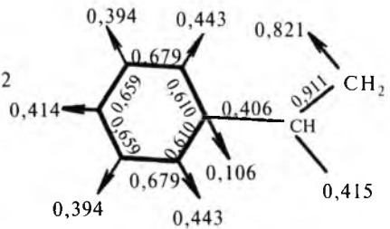
Stirol
