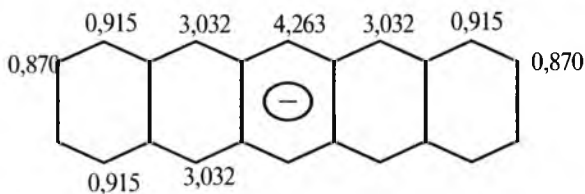
Pentatsen anion-radikali
