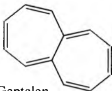
Geptalen
