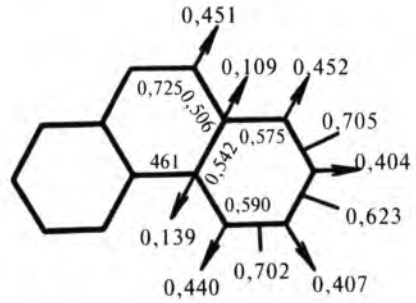
Fenaktren
