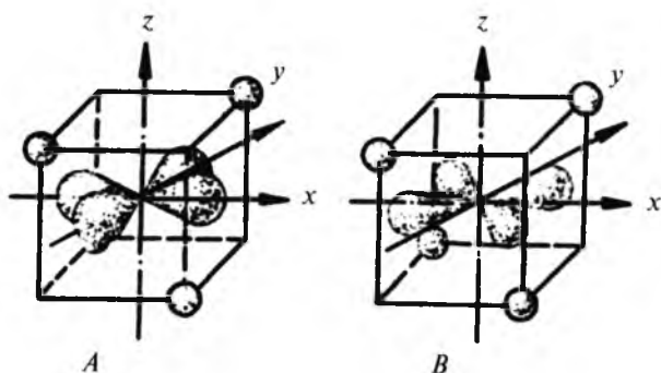
2.59-rasm. Metall d_{x^2-y^2} va d_{xy} orbitalarining ligandlarning tetraedrik maydonida joylashishi.
