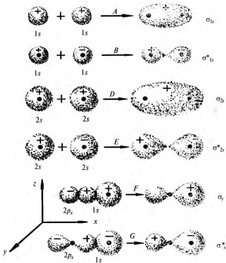
2.16-rasm. Turli AO lardan bog'lovchi va ajratuvchi MO larning hosil bo'lishi. Nuqtalar bilan yadrolar ko'rsatilgan. Musbat va manfiy belgilar shu sohalaridagi to'liq funksiyaning ishorasini bildiradi
