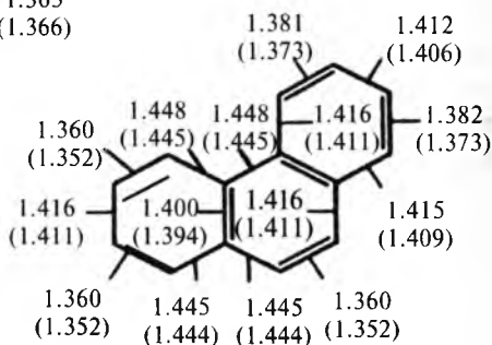
Fenantren
