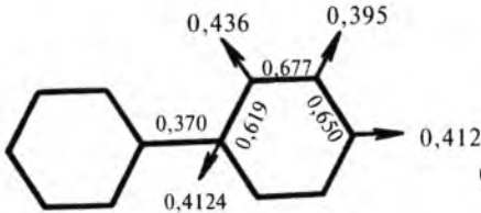
Difenil
