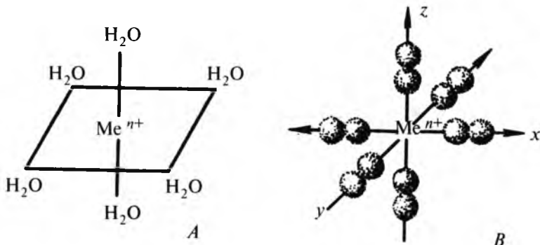
2.63-rasm. Oktaedrik kompleksda metall atomi va ligandlarning (A) hamda [\text{Me}(\text{H}_2\text{O})_6]^{n+} komplekslarda kislorod 2p_x AO larining fazoda joylashishi.
