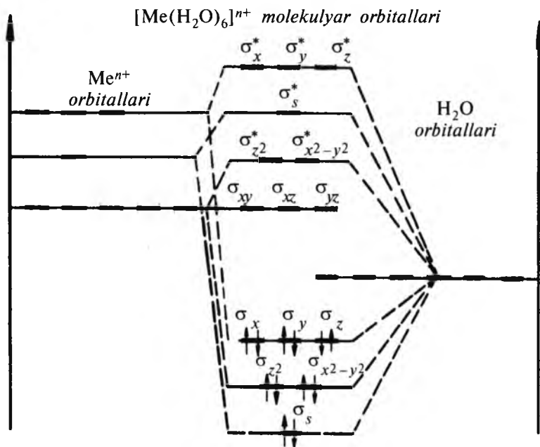
2.65-rasm. [Ti(H_2O)_6]^{3+} kompleksi MO larining energetik pog'onalari va ularning elektronlar bilan to'lishi.
