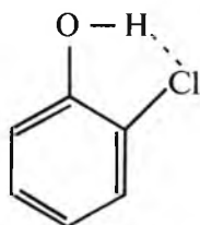
Sis-ortoxlorfenol
