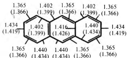
Atracen
