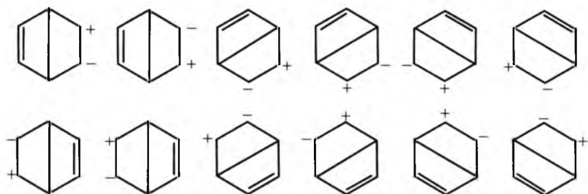
3.1- rasm. Benzolning qutbli rezonans tuzilishlari.
