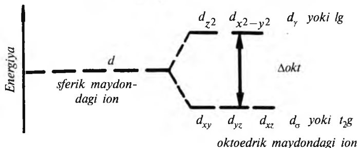
2.58-rasm. Metall d -orbitallari energetik pog'onalarning oktaedrik kompleks ligandlari maydonida ajralishi.
