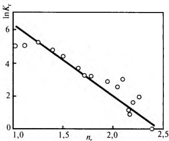
4.20-rasm. AU larni nitrolash reaksiyalarida \lg K_r va n_r ning o'zaro bog'liqligi.
