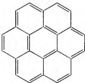
Koronen
