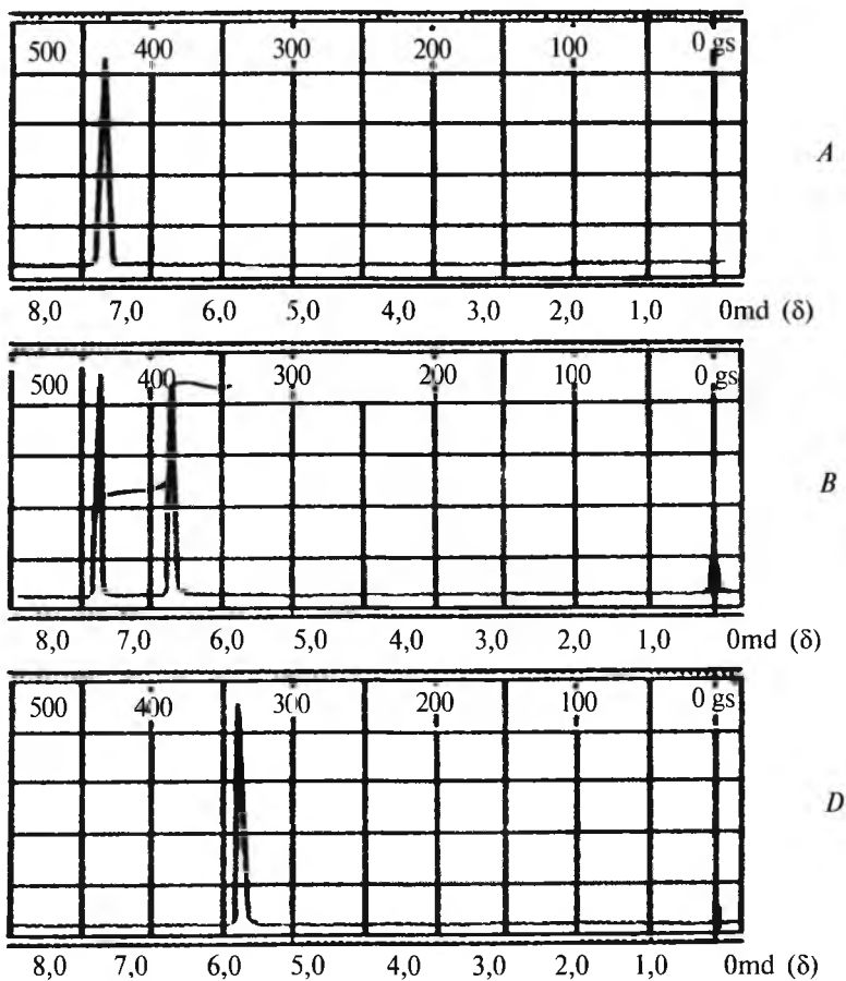
3.23-rasm. Aromatik birikmalar – benzol A , furan B va noaromatik siklooktatetrayen C ning YaMR-spektrlari.
