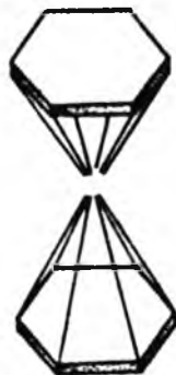
Dibenzolxrom
