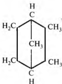
(6.42) Norbornan
