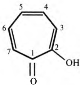
Enol-forma
