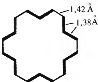
3.18-rasm. \text{C}_{18}\text{H}_{18} makrosikldagi bog'lar alternatsiyasi.
