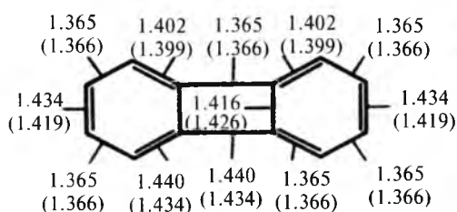
Difenilen
