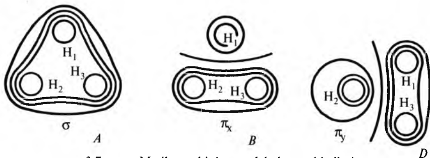
3.7-rasm. Metil guruhining molekulyar orbitalari.
