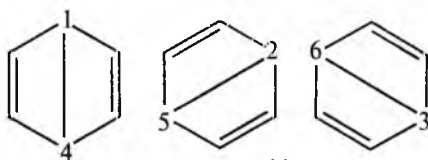
J. Dyuar (1866- y)
