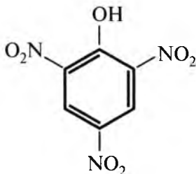
2,4,6-trinitrofenol
