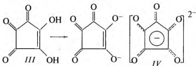
Krokonat kislota
