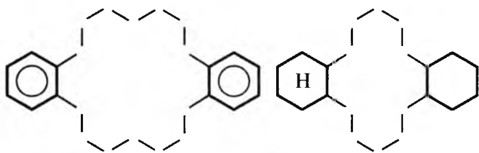
Dibenzo-18-kraun-6
