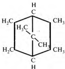
(6.44) Kamfan
