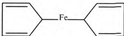
Temi siklopentadiyenil
