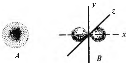
2.7-rasm. s -( A ) ba p -( B ) elektron bulutning ko'rinishi.
