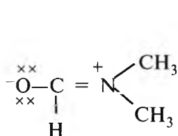
Dimetilformamid
