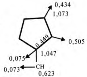
Fulven
