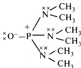
Geksametilfosfotriamid
