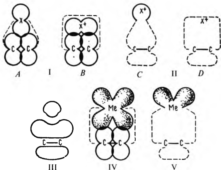
6.11-rasm. I — elektrofil ( X^+ ) ning bo'sh p -orbitalining etilendagi \pi -orbital bilan ikki xil qoplanishi (A, B); II — bu qoplanishda vujudga keladigan bog'lovchi C, D va III — ajratuvchi MO lar; IV — metallning bo'sh d -orbitali bilan qo'shbog' \pi -orbitalining qoplanshsh va V — bunda hosil bo'ladigan bog'lovchi MO.
