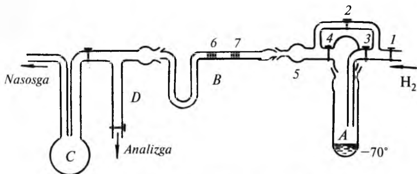
6.6-rasm. Panet usulida radikallar hosil qilish qurilmasi.
