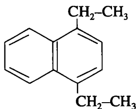
p-dietil-naftalin
