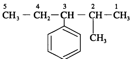
2-metil-3-fenilpentan
