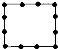
siklododekan
