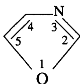
oksazol
