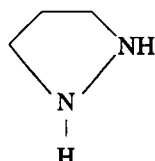
pirazolidin
