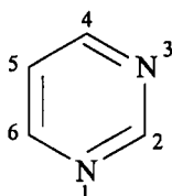
pirimidin ( 1,3 – diazin )
