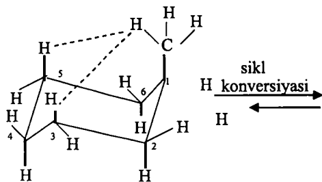
\alpha – metilsiklogeksan
