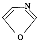
oksazol
