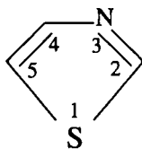
tiazol
