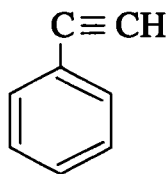
etinilbenzol, fenilatsetilen
