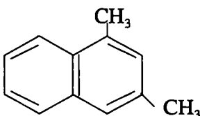
m-dimetil-naftalin
