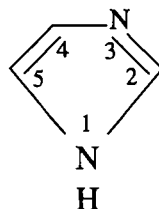
imidazol
