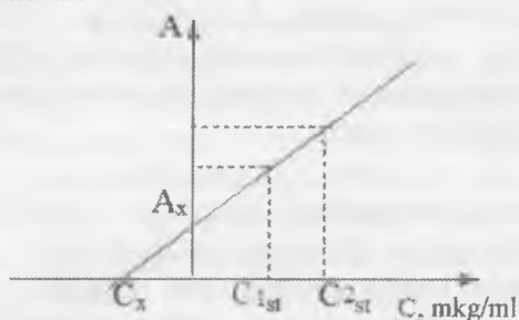
24.15-rasm. Qo'shilmalar qo'shish metodini grafigi
