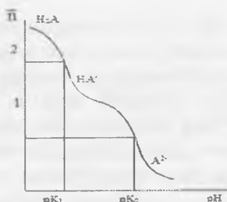
5.2-rasm. Ko'p protonli kislotalarda alohida formalarning pH ga bog'liqligining hosil bo'lish egrisi
