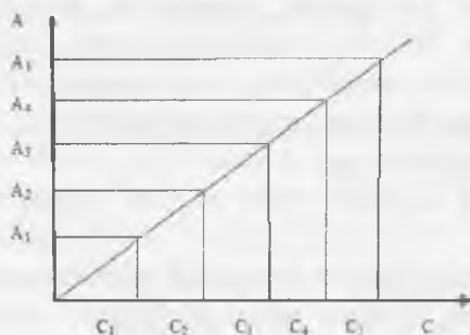
24.5-rasm. Darajalangan grafik
