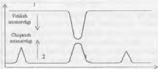
26.2-rasm. Atom-absorbsion spektroskopiyada chiqarish va yutilish spektrlari. 1 – namunaning yutish spektri; 2 – yorug'lik manbasining chiqarish spektri.
