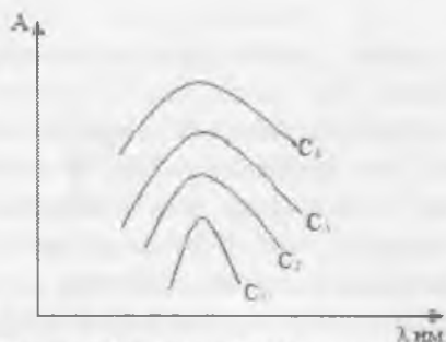
24.4-rasm. Nur yutilishining to'liqin uzunligiga bog'liqligi
