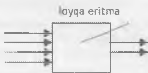
24.9-rasm. Turbidimetrik aniqlashda nur dastasining o‘tishi.
