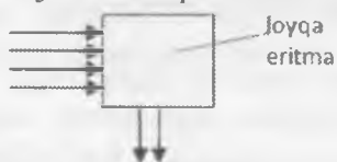
24.8-rasm. Nefelometrik aniqlashda nur dastasining o‘tishi.
