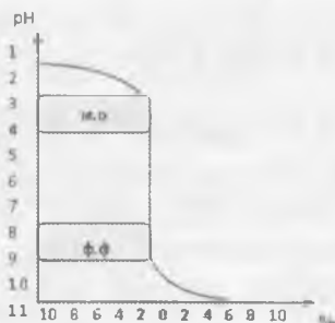
20.1-rasm. Kuchli kuchli kislotani asos bilan titrlash egrisi
