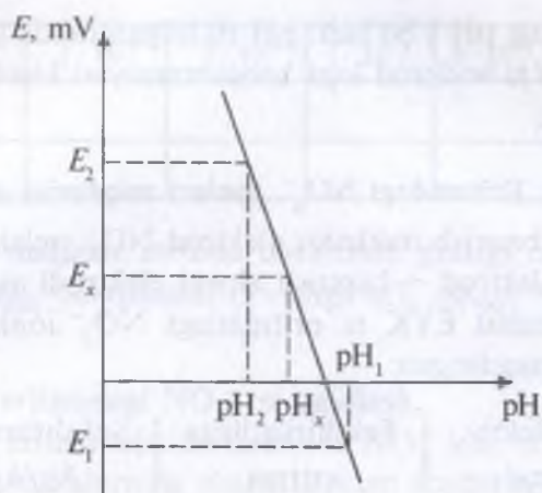
12- rasm. Darajalash grafigi.
