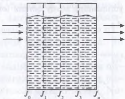
20- rasm. Yorug'lik oqimi jadalligining yutuvchi qatlam qalinligiga bog'liq holda o'zgarishi.
