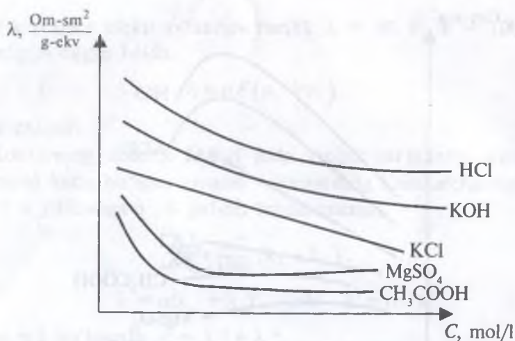
15- rasm. Ekvivalent elektr o'tkazuvchanlikning konsentratsiyaga bog'liqligi.
