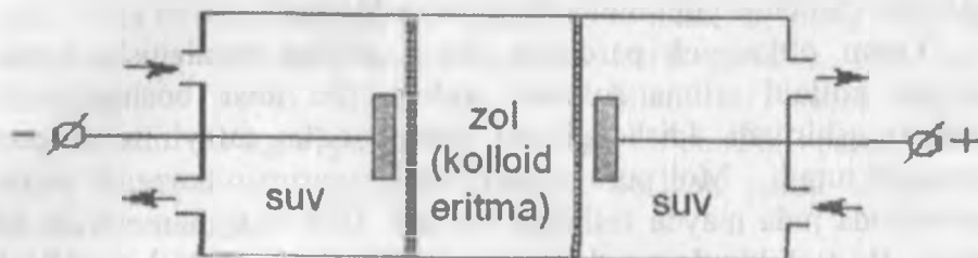
Rasm. Elektrodializator sxemasi
