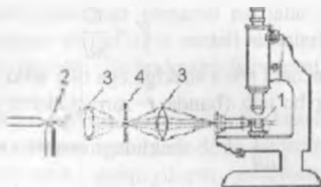
Ultramikroskop sxemasi.
