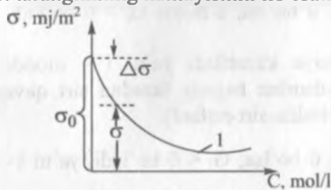
Sirt taranglik izotermasi
