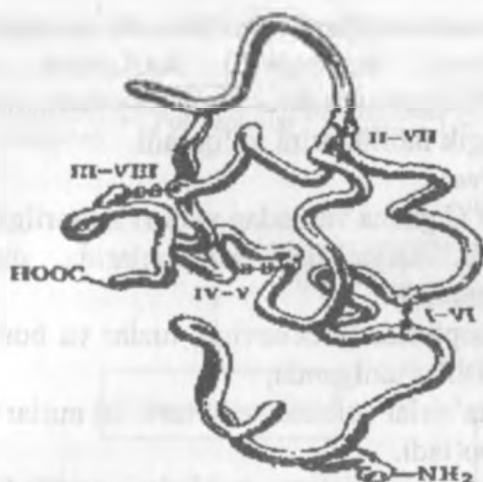
Ribonukleazaning uchlamchi strukturasi rim raqamlari bilan sistein qoldig'idagi S-S bog'ları ko'rsatilgan
