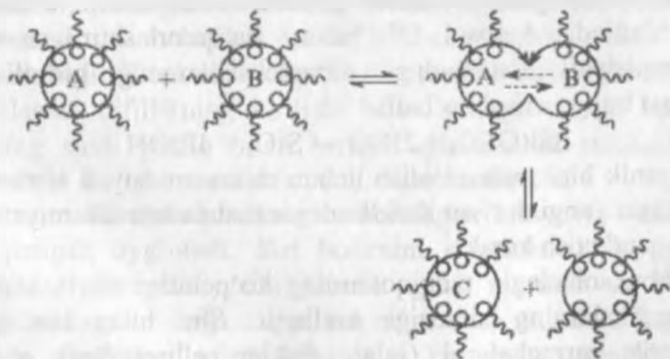
2-rasm. Teskari mikroemulsiyali sistemada boradigan reaksiya sxemasi
