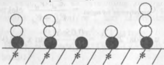
BET nazariyasiga ko'ra polimolekulyar adsorbsiya sxemasi
