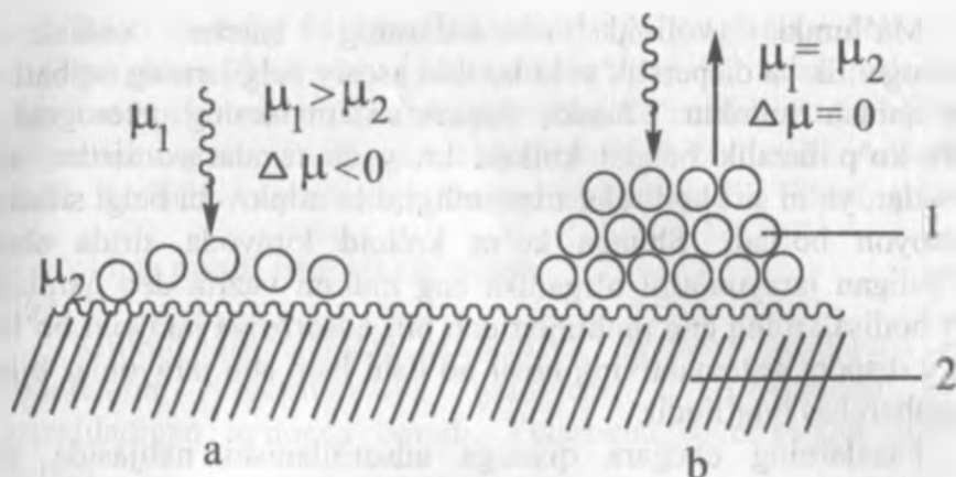
Rasm. Jarayonning boshida (a) va muvozanat vaqtidagi (b) adsorbsiya
