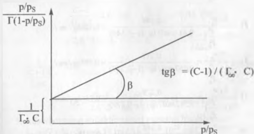
Rasm. Polimolekulyar adsorbsiya izotermasi
