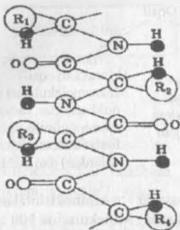
Oqsilning birlamchi strukturasi
