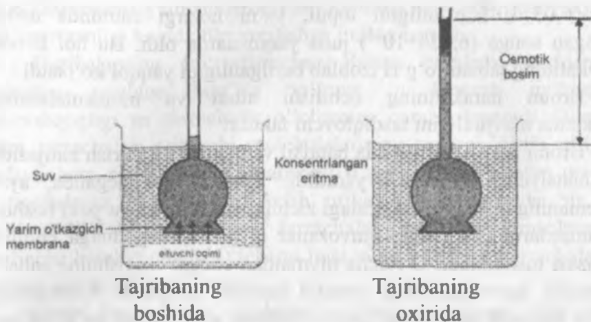
Rasm. Osmotik bosimning ta'sirini ko'rsatuvchi tajriba
