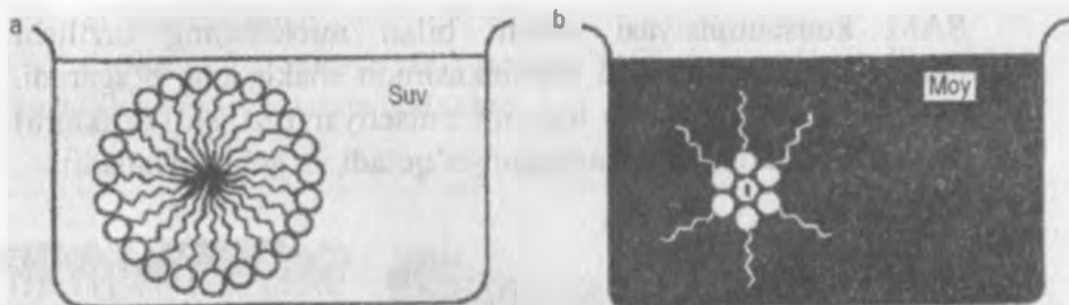
To'g'ri mitsella yadrosi
