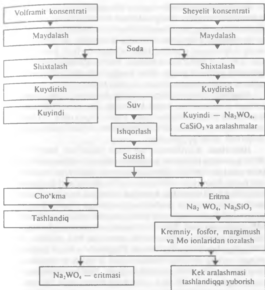
1- chizma. Volfram yoki sheyelit konsentratlarini kuydirish texnologiyasi.
