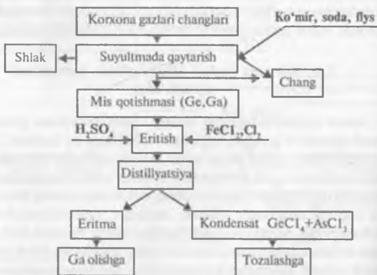
9- chizma. Korxona gazlari va changidan germaniyni olish texnologik sxemasi.
