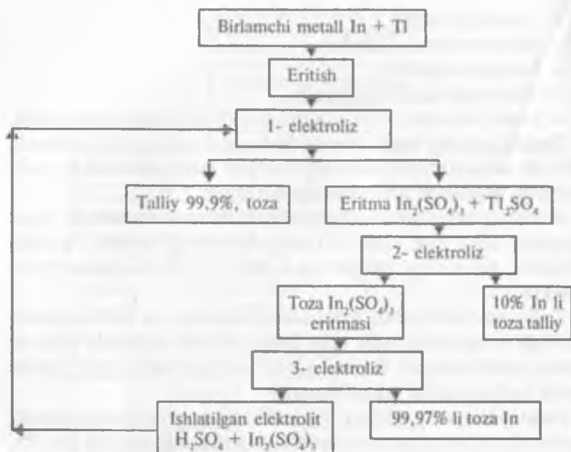
14-chizma. Indiyni elektrokimyoviy usulda olish.
