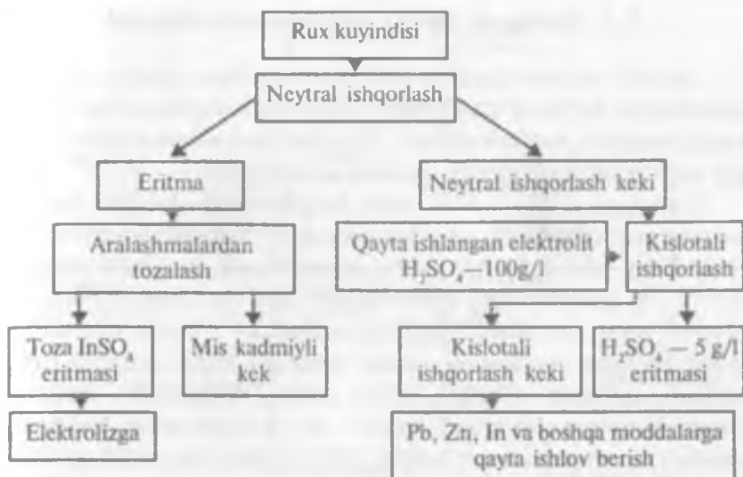
11- chizma. Rux ishlab chiqarishning gidrometallurgik texnologiyasu.
