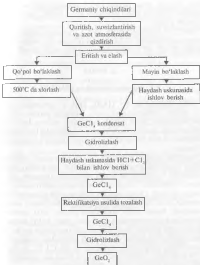
10-chizma. Germaniy IV oksidini chiqindilardan olish.
