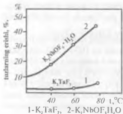
1- grafik. Kaliy fiortantalat fiorksninobat tuzlarining 1% li plavik kislotasi va harorat o'zgarishi.
