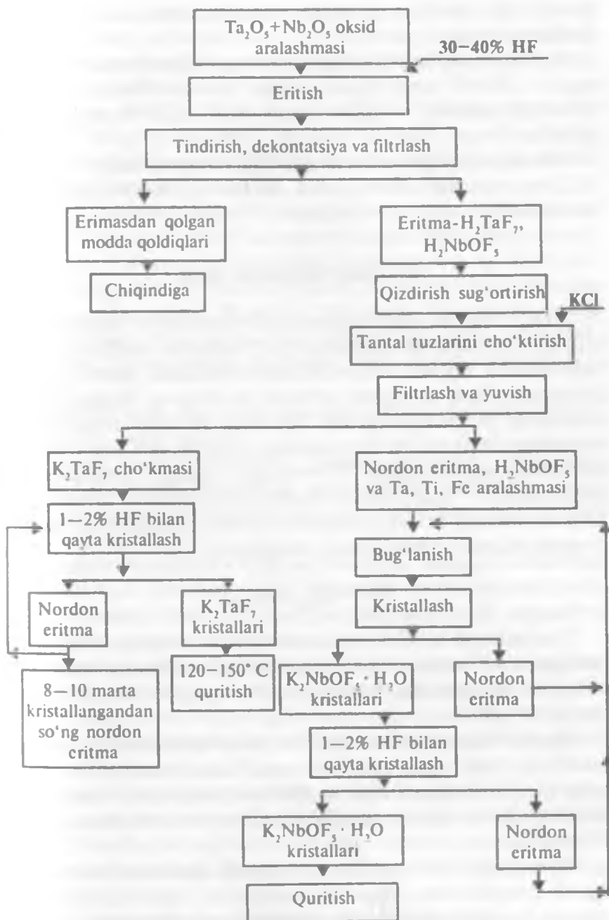
7- chizma. Tantal va niobiyning stor kompleks tuzlarini olish texnologiyasi.
