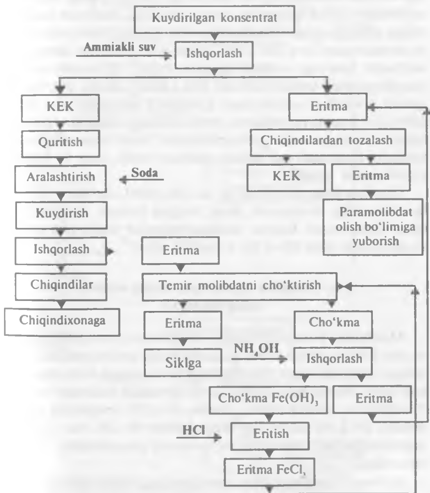
3- chizma. Chiqindilardan molibden olish texnologiyasi.
