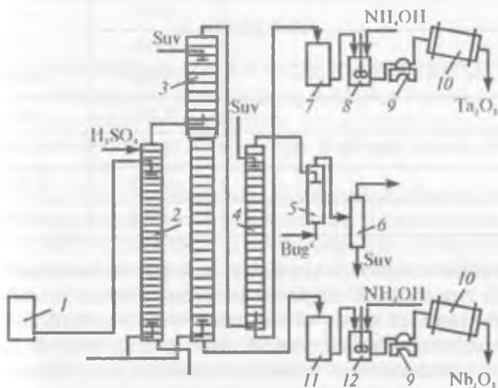
2- rasm. Ekstraktsiya usulida tantal va niobiyni ajratib olish texnologiyasi.
