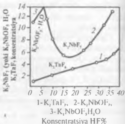
2- grafik. Turli konsentratsiyali plavik kislotalarda tantal va niobiyning fiorti komplekslarining ( 25^{\circ}C da) erishi.
