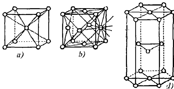
1- rasm. Metallar kristall panjalarining asosiy turlari.
