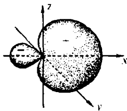
18-rasm. sp -gibrid orbitallarining alohida hosil bo'lish sxemasi.
