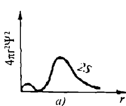
8-rasm. 2s- va 3s- elektronlarning radial taqsimlanish grafigi.
