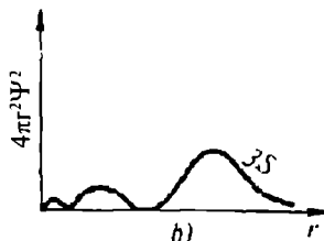
8-rasm. 2s- va 3s- elektronlarning radial taqsimlanish grafigi.
