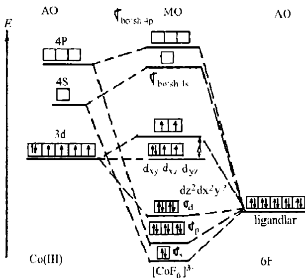
27 ras. Molekular orbitallar usulida past spinli [\text{Co}(\text{NH}_3)_6]^{3+} va yuqori spinli [\text{CoF}_6]^{3-} komplekslarining energetik diagrammalari tuzilishi.
