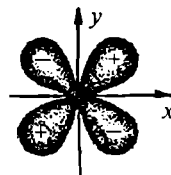
12- rasm. 3d- elektronlar bulutining fazoviy shakli.
