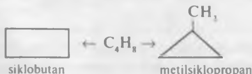
siklobutan
