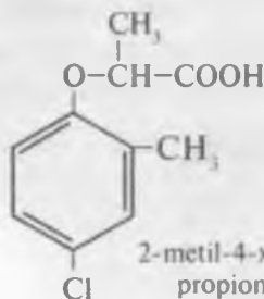
2-metil-4-xlorfenoksisirka kislota
