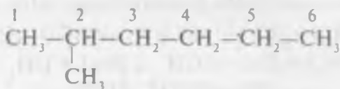
2-metilgeksan
