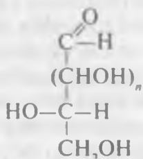
L-monosaxarid
