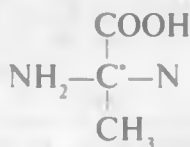
l -alanin
