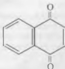
p-naftaxinon
