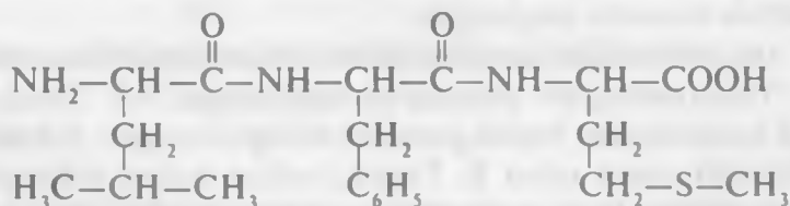
leysilfenilalanilmetsionin
