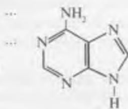
adenin
