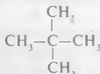
tetrametilmetan
