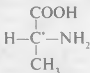
d -alanin
