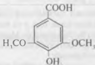
siren kislota
