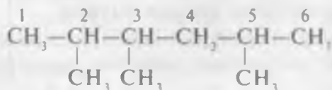
2, 3, 5-trimetilgeksan
