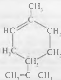
limonen
