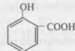
salitsil kislota
