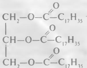
oddiy glitserid
