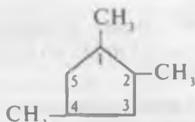
1,2,4-trimetilsiklopentan
