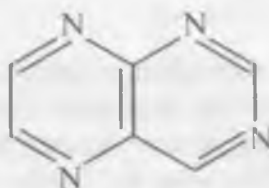
pteridin
