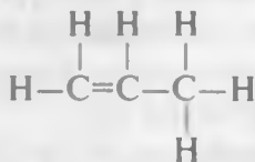
propilen (metil-etilen)
