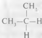
dimetilmetan
