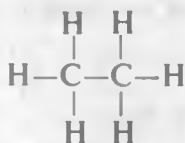
etan
