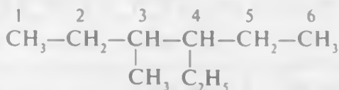
3-metil-4-etilgeksan
