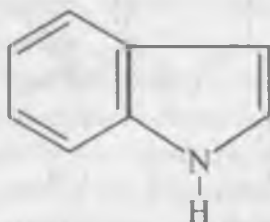
indol
