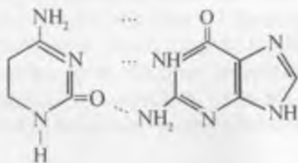
sitozin
