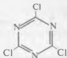
sianur-xlorid
