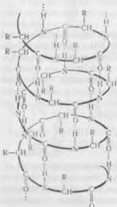
15-rasm. Oqsil molekulasiining ikkilamchi strukturasi.
