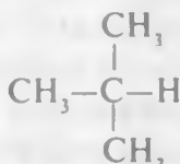
trimetilmetan
