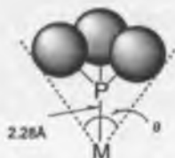
Fig. 4.8 Cone angle.
