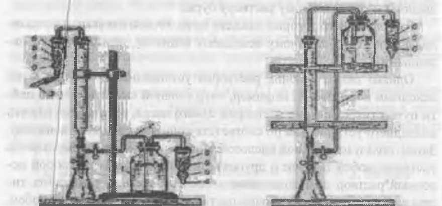
Рис. 4 Два способа соединения бюретки со склянкой, содержащей запасной рабочий раствор: 1 — склянка с раствором; 2 — сифон для переливания раствора в бюретку; 3 — трубка для засасывания раствора; 4 — трубка для натронной извести; 5 — натронная известь; 6 — вата
