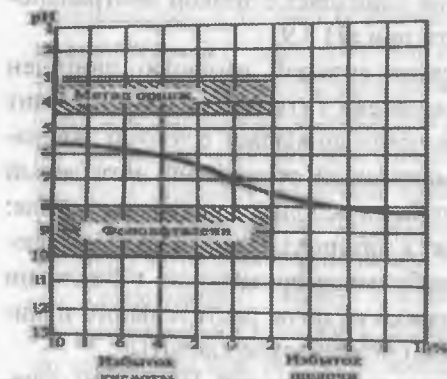
Рис. 11 Кривая нейтрализации слабой кислоты слабой щелочью
