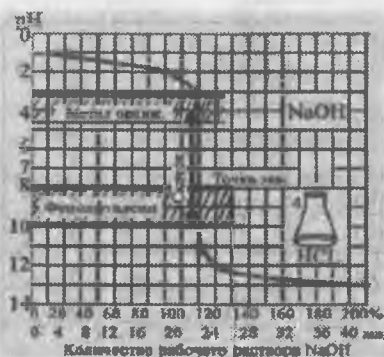
Рис. 8. Кривая титрования сильной кислоты сильной щелочью
