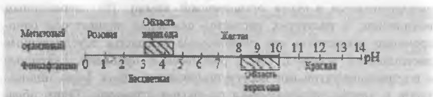
Рис. 7 Окраска фенолфталеина и метилового оранжевого при различных значениях pH
