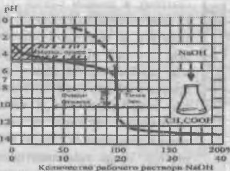
Рис. 9. Кривая титрования слабой кислоты сильной щелочи
