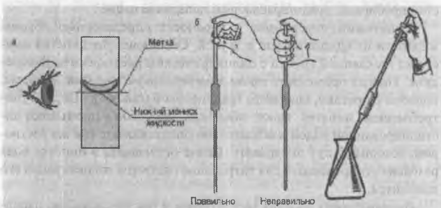
Рис. 6 Выливание раствора из пипетки
