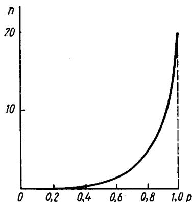
Рис. 5.3. Зависимость степени полимеризации ( n ) при линейном ступенчатом процессе синтеза полимеров от глубины превращения функциональных групп ( p )
