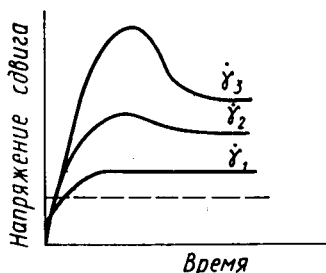
Рис. 11.9. Зависимость напряжения сдвига \tau от времени вращения внутреннего цилиндра ротационного вискозиметра:
