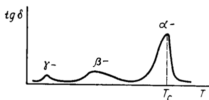
Рис. 10.7. Вторичные релаксационные переходы в стеклообразном полимере
