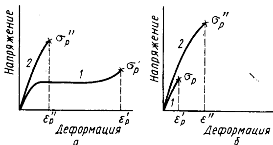
Рис. 12.16. Влияние ориентации на вид кривых напряжение — деформация:
