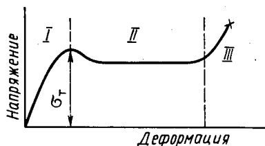
Рис. 10.2. Схематическое изображение кривой напряжение — деформация стеклообразного полимера:
