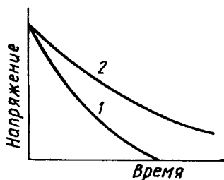
Рис. 9.19. Релаксация напряжения:
