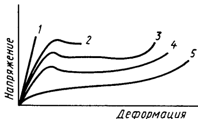
Рис. 10.5. Влияние температуры на вид кривых напряжение — деформация для стеклообразных полимеров: T_1 < T_2 < T_3 < T_4 < T_5 ; 1 — при T_1 < T_{хр} ; 5 — при T_5 > T_c
