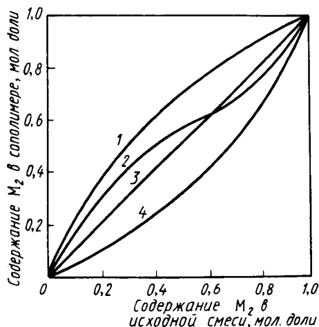
Рис. 4.1. Зависимость состава сополимера от состава исходной смеси мономеров для статистической сополимеризации мономеров M_1 и M_2 при различной реакционной способности их радикалов (различные значения констант сополимеризации r ):
