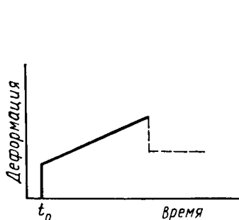
Рис. 9.5. Кривая ползучести для модели Максвелла:
