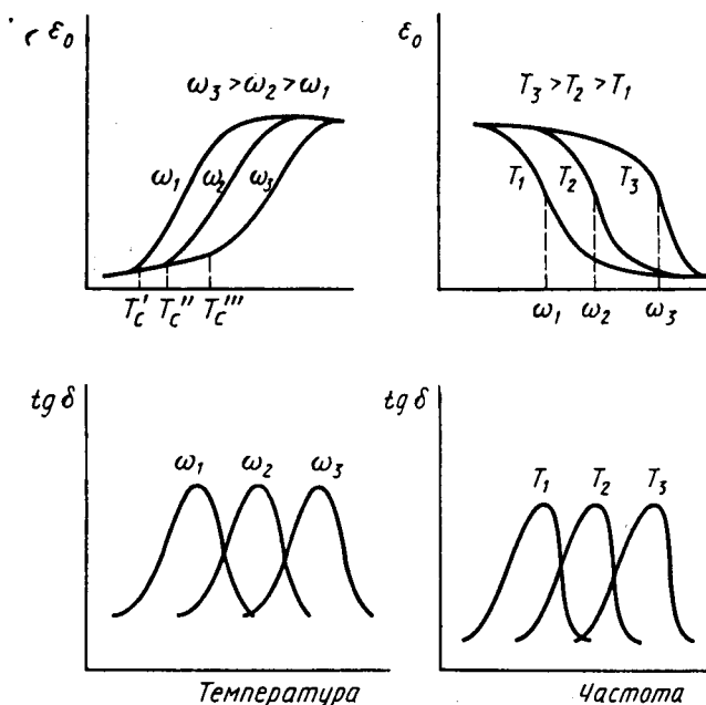
Рис. 9.16. Изменение амплитуды деформации и \lg \delta при изменении частоты и температуры
