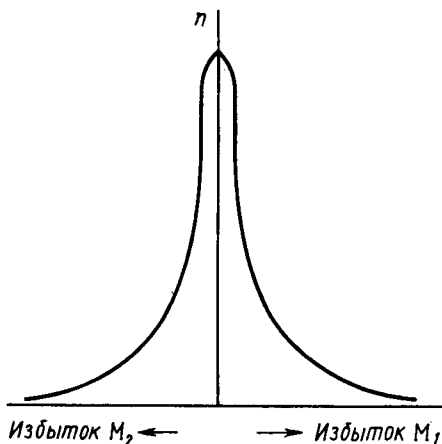
Рис. 5.2. Зависимость степени полимеризации от соотношения мономеров в исходной смеси для ступенчатых реакций синтеза полимеров
