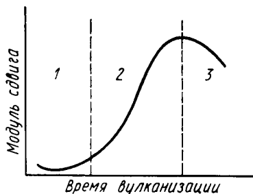
Рис. 20.1. Типичная кинетическая кривая вулканизации эластомеров:
