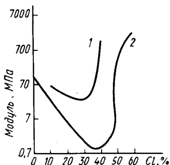
Рис. 14.1. Зависимость жесткости (модуля) хлорированного полиэтилена от содержания присоединенного хлора при проведении процесса хлорирования в водной суспензии (1) и в растворе тетрагидрофурана (2) [4]
