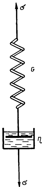
Рис. 9.2. Модель Максвелла
