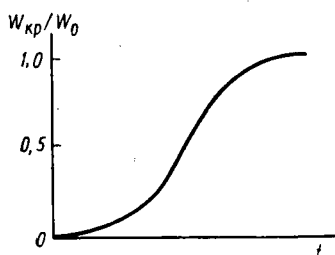
Рис. 12.7. Изотерма кристаллизации полимера
