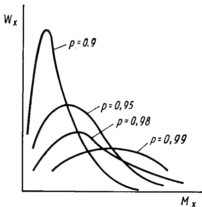
Рис. 5.4. Изменение молекулярно-массового распределения в процессе ступенчатого синтеза линейного полимера в зависимости от глубины превращения его функциональных групп
