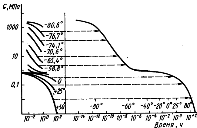
Рис. 9.18. Построение обобщенной кривой релаксации напряжения для полиизобутилена при 25°C
