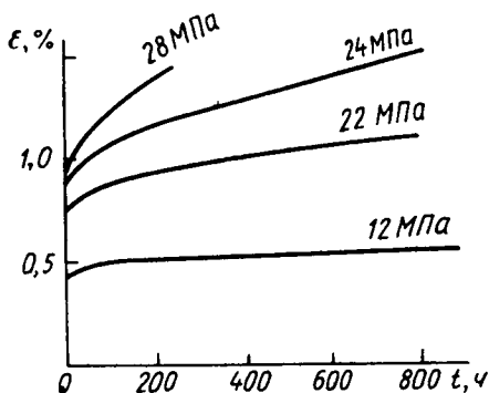
Рис. 10.6. Ползучесть полистирола при 25°C и разных величинах действующего напряжения
