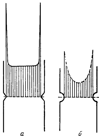
Рис. 13.1. Концентрация напряжений на микродефекте с острой (а) и сглаженной (б) вершинами
