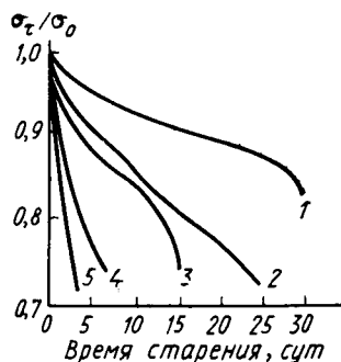
Рис. 18.8. Изменение сопротивления старению пероксидных вулканизаторов цис -1,4-полиизопрена (натуральный каучук) в присутствии защитных добавок (0,01 моль на 1 г вулканизата):
