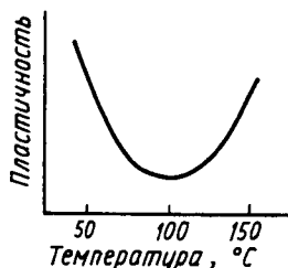
Рис. 17.2. Зависимость пластичности полиизопрена от температуры его механохимической переработки на вальцах
