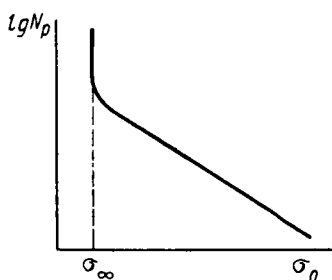
Рис. 13.14. Зависимость числа циклов до разрушения \lg N_p от амплитуды напряжения для высокомодульного материала (пластмасса)
