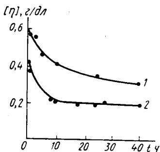
Рис. 15.2. Падение характеристической вязкости полиэтилена в тетралине при 75°C в зависимости от времени пиролиза полиэтилена при 315°C (1) и 360°C (2)
