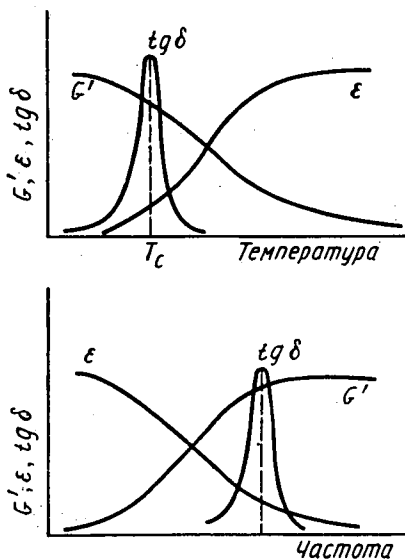
Рис. 9.15. Зависимость модуля упругости G' , амплитуды деформации \varepsilon и \text{tg } \delta от температуры и частоты деформации
