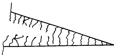
Рис. 13.3. Строение микротрещины, заполненной ориентированными сегментами полимера: показано начало роста трещины, разрывающей ориентированные молекулы внутри микротрещины
