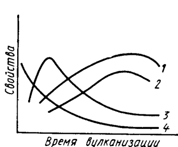
Рис. 20.2. Характерные кривые изменения свойств эластомеров при вулканизации:
