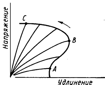
Рис. 13.5. Диаграмма (огibaющая разрывов), показывающая зависимость хода кривой \sigma — \epsilon от температуры или скорости деформации:
