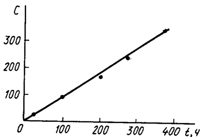
Рис. 17.3. Гидролиз волокон из аморфного полиэтилентерефталата в соляной кислоте при 70°C. Зависимость концентрации концевых групп C (моль \cdot 10^{-6}/\text{г} полимера) от времени
