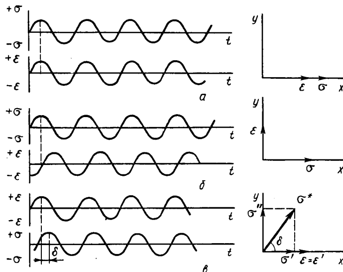
Рис. 9.13. Синусоиды напряжения и деформации и сдвиг по фазе между ними при частотном деформировании: а — упругого, б — вязкого и в — вязкоупругого тела
