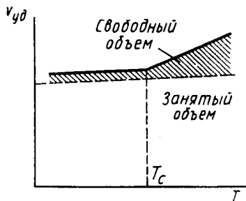
Рис. 10.1. Зависимость удельного объема ( v_{уд} ) от температуры. Температурное изменение свободного и занятого объема
