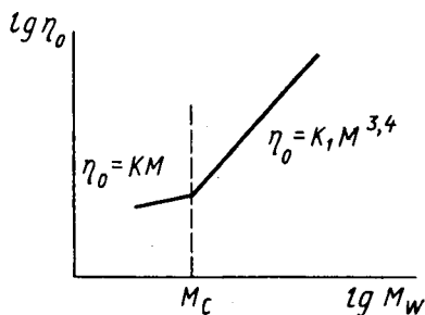
Рис. 11.8. Зависимость начальной ньютоновской вязкости от средней молекулярной массы в двойных логарифмических координатах
