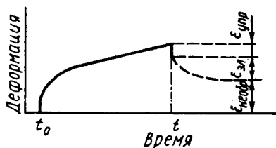
Рис. 9.9. Кривая ползучести для объединенной механической модели [уравнение (9.13)]
