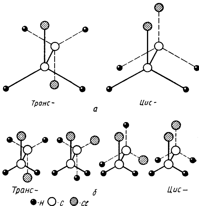
Рис. 7.1. Различные расположения атомов в молекуле этана (а) и дихлорэтана (б)
