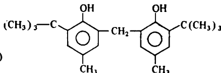
2,2'-метилден-бис (-4метил-6-трет-бутилфенол) (НГ-2246; антиоксидант 2246)
