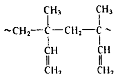
полиизопрен-1,2
