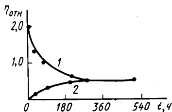
Рис. 15.1. Изменение в процессе нагревания с пероксидом бензоила относительной вязкости растворов в толуоле:
