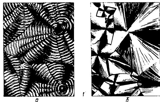
Рис. 12.5. Различные типы сферолитов: а — кольцевой, б — радиальный
