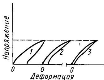
Рис. 9.11. Уменьшение площади петли гистерезиса при повторении циклов растяжение — сжатие (1, 2, 3). После некоторого числа циклов ( n ) площадь петли стабилизируется (3)
