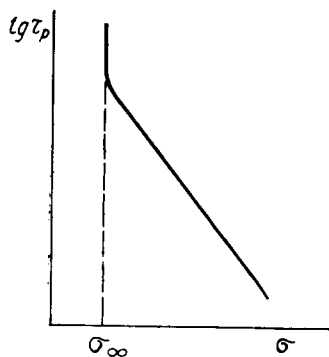
Рис. 13.10. Схема, показывающая наличие безопасного напряжения
