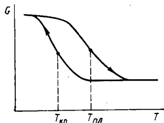
Рис. 12.10. Температурная зависимость модуля упругости G кристаллического полимера в области плавления:
