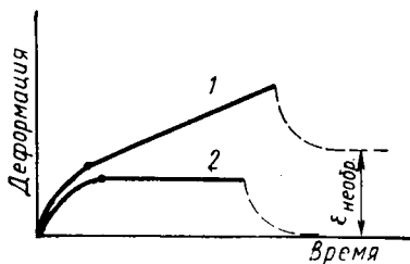
Рис. 9.4. Ползучесть в линейном (1) и пространственном (2) полимере:
