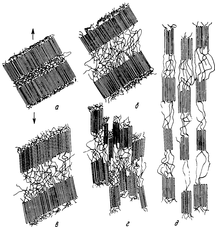
Рис. 12.12. Схема перестройки структуры кристаллического полимера в процессе деформации
