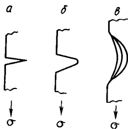
Рис. 13.4. Постепенное уширение устья трещины в эластомере и скругление ее вершины (а, б); образование тяжей на поздней стадии растяжения перед разрывом (в)
