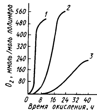
Рис. 18.7. Кинетические кривые окисления цис -1,4-полиизопрена (натуральный каучук) при 120°C в присутствии 1,5% (1) и 0,5% (2) стеарата железа и без него (3)
