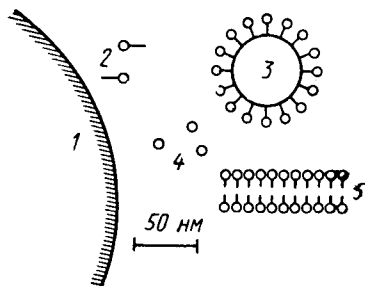
Рис. 6.1. Схематическое изображение эмульсионной полимеризации (примерное содержание частиц в 1 см 3 указано в скобках) [13]:
