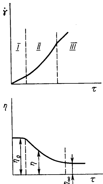
Рис. 11.7. Зависимость скорости сдвига и вязкости от напряжения сдвига \tau :
