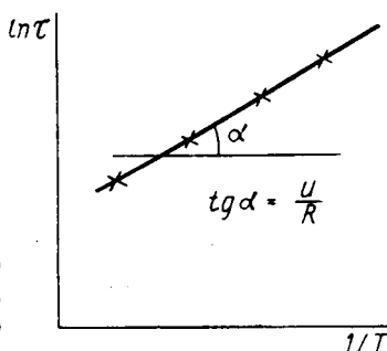
Рис. 9.17. Определение энергии активации процесса релаксации
