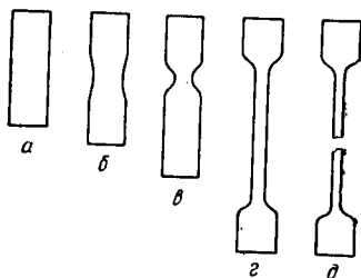
Рис. 10.3. Различные стадии деформации стеклообразного полимера:
