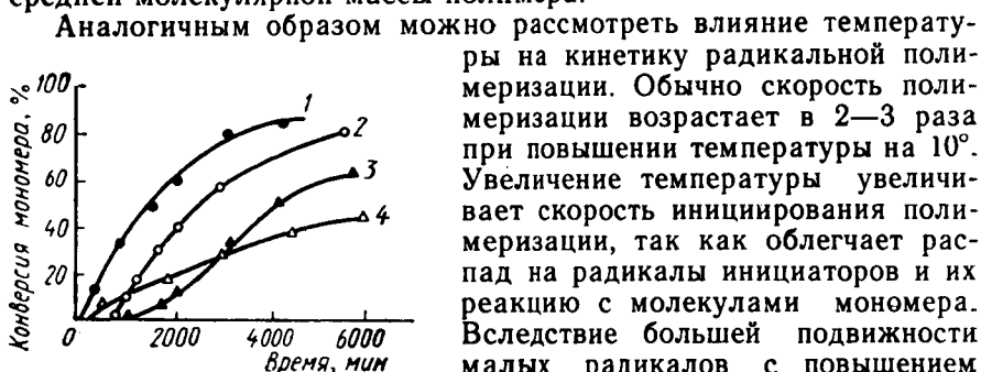
Рис. 1.3. Термическая полимеризация стирола при 100°C в присутствии ингибиторов и замедлителей: 1 — без добавок; 2 — 0,1% бензохинона (ингибитор); 3 — 0,2% нитробензола (ингибитор); 4 — 0,5% нитробензола (замедлитель)
