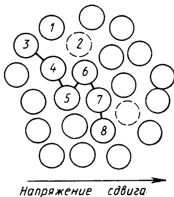
Рис. 11.6. Схема, поясняющая механизм течения низкомолекулярной и высокомолекулярной жидкости под действием напряжения сдвига \tau
