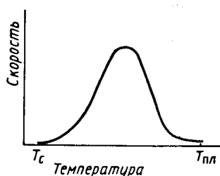
Рис. 12.8. Зависимость скорости кристаллизации от температуры
