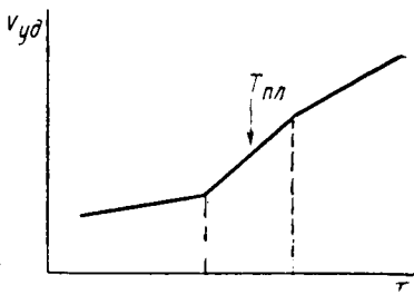
Рис. 12.9. Зависимость удельного объема V_{уд} от температуры для кристаллического полимера в процессе нагревания: пунктиром отмечен интервал температур между началом и концом плавления
