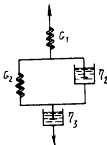
Рис. 9.8. Объединенная механическая модель вязкоупругого полимера
