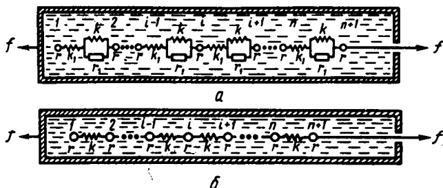
Рис. 9.20. Модель макромолекулы по Каргину и Слонимскому:
