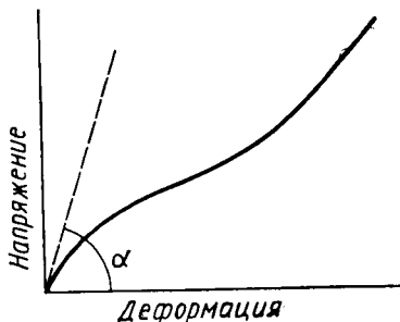
Рис. 8.3. Кривая напряжение — деформация эластомера: E — модуль растяжения; \operatorname{tg} \alpha = E
