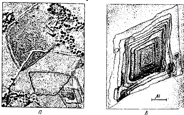
Рис. 12.6. Монокристаллы полиэтилена: а — плоский; б — пирамида
