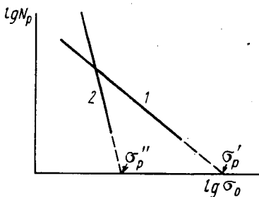
Рис. 13.15. Зависимость числа циклов до разрушения \lg N_p от амплитуды напряжения \lg \sigma_0 для низкомоульного материала (резина)
