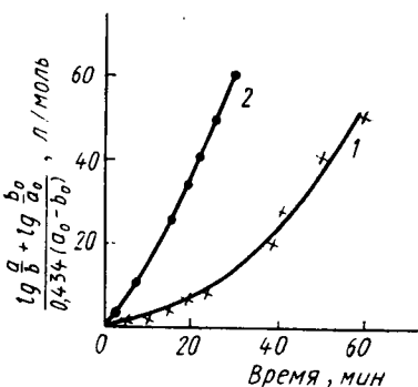
Рис. 14.3. Кинетика гидролиза поливинилацетата [4] со степенью полимеризации около 9000 (1) и этилацетата (2) в среде ацетон — вода в отношении 70 : 30 об. долей, % при 20°C:
