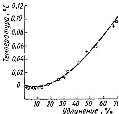
Рис. 8.5. Изменение температуры натурального каучука в процессе деформирования
