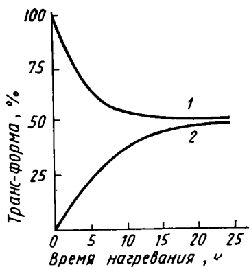
Рис. 19.2. Изомеризация транс -1,4-полиизопрена (гуттаперча) — 1 и цис -1,4-1,4-полиизопрена (натуральный каучук) — 2 при 140°C под действием диоксида серы
