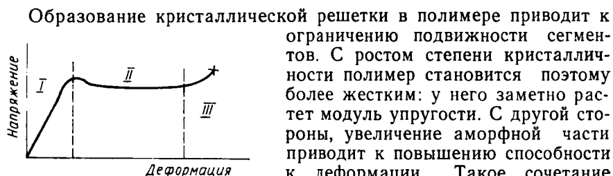
Рис. 12.11. Кривая напряжение — деформация кристаллического полимера
