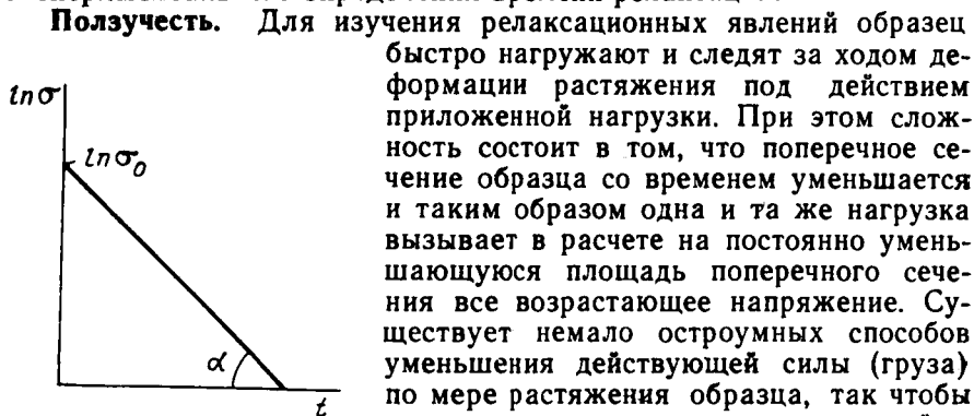
Рис. 9.3. Релаксация напряжения в модели Максвелла (9.10) и определение времени релаксации \tau = 1/\operatorname{tg} \alpha
