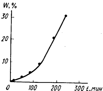
Рис. 15.3. Кинетика выделения уксусной кислоты ( W , %) при термодеструкции поливинилацетата при 235^{\circ}\text{C}
