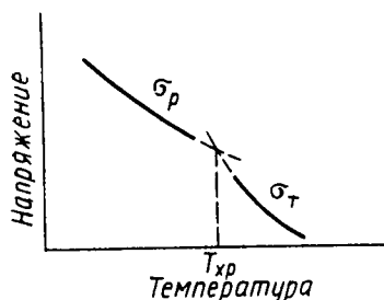
Рис. 10.8. Зависимость прочности \sigma_p и предела вынужденной эластичности \sigma_t от температуры:
