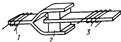
Рис. 9.12. Рабочий узел прибора для частотного нагружения образца:
