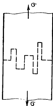
Рис. 13.7. Распространение трещины в высокоориентированном полимере
