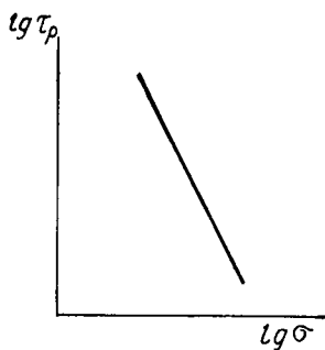
Рис. 13.11. Зависимость долговечности от напряжения для эластичных полимеров
