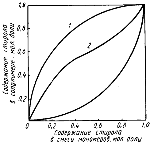
Рис. 4.2. Зависимость состава сополимера от состава исходной смеси мономеров при сополимеризации стирола с метилметакрилатом различными способами:
