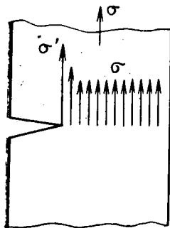
Рис. 10.4. Концентрация напряжений при растяжении образца, имеющего дефект в виде микротрещины
