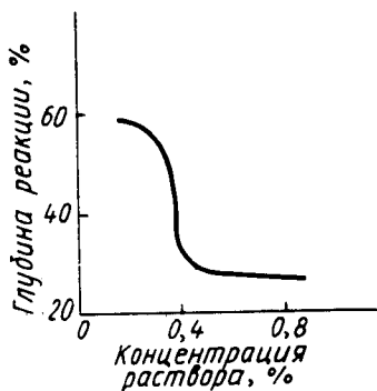
Рис. 19.1. Изменение глубины реакции присоединения тиобензойной кислоты к цис -1,4-полиизопрену в зависимости от концентрации его растворов
