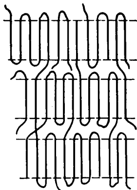
Рис. 12.3. Схема соединения ламелей проходными молекулами. Наличие аморфных областей между ламелями
