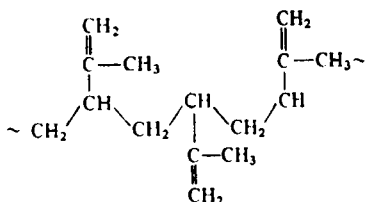
3,4-полиизопрен синдиотактический
