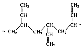
1,2-синдиотактическая
