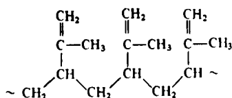
3,4-полиизопрен изотактический
