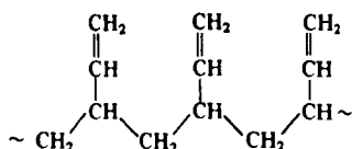
1,2-изотактическая
