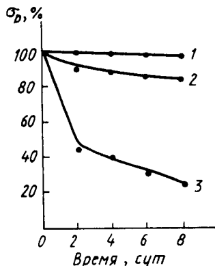
Рис. 18.6. Зависимость разрывной прочности полиамидного волокна капрон ( \sigma_p в % от исходного) от продолжительности нагревания на воздухе при различных температурах:
