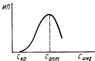
Рис. 18.10. Зависимость продолжительности индукционного периода (мин) окисления полимера от концентрации ингибитора процесса (г/моль полимера): на оси абсцисс указаны положения критической и оптимальной концентраций ингибитора
