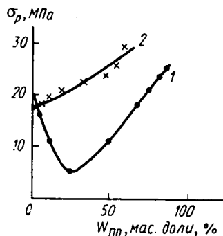
Рис. 14.2. Зависимость разрывной прочности блок-сополимеров этилена с пропиленом от содержания звеньев пропилена ( W_{пр} , мас. %) при 6 (1) и 24 (2) блоках в цепи [4]
