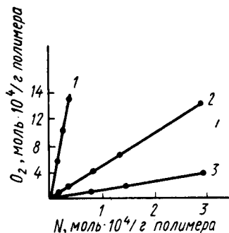
Рис. 18.5. Зависимость между количеством присоединенного в процессе окисления кислорода и степенью деградации сшитого полиизопрена (число разрывов молекулярных цепей N ) при различных температурах окисления:
