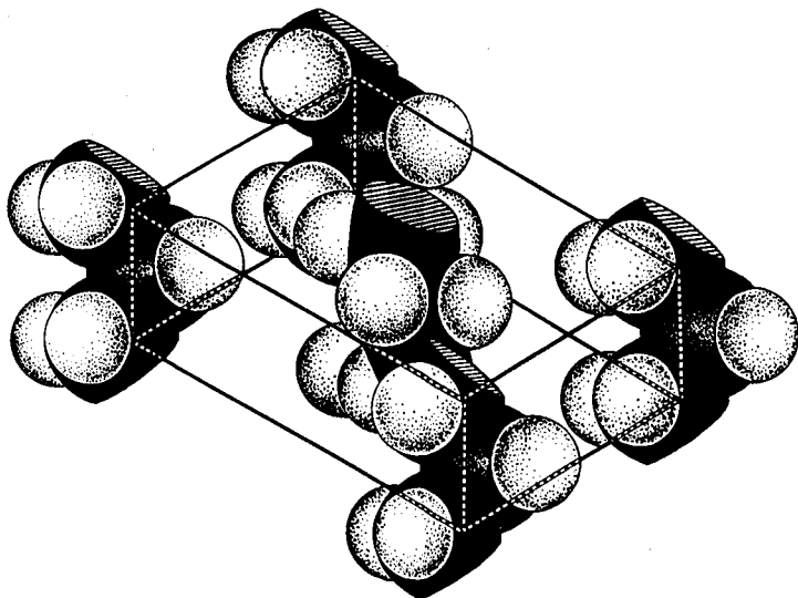
Рис. 12.1. Расположение участков макромолекул полиэтилена в элементарной ячейке кристалла
