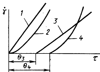
Рис. 11.1. Различные типы кривых течения (реологических кривых):
