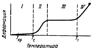
Рис. 7.6. Термомеханическая кривая аморфного полимера:
