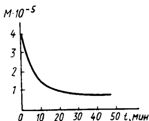
Рис. 17.1. Падение молекулярной массы сополимера бутадиена со стиролом в зависимости от времени обработки на вальцах в присутствии 1% \beta -тионафтола (акцептор свободных радикалов)
