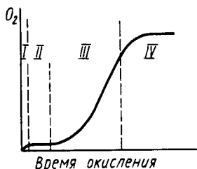
Рис. 18.1. Кинетическая кривая окисления полимеров:
