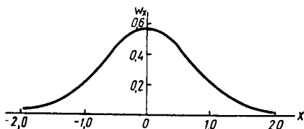
Рис. 8.6. Вид функции распределения, описываемый уравнением (8.15)
