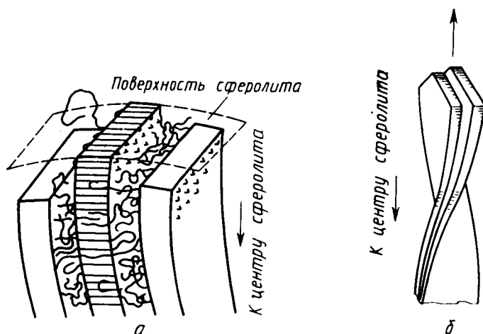
Рис. 12.4. Схема укладки макромолекул в сферолите. Расположение ламелей в радиальном (а) и кольцевом (б) сферолите
