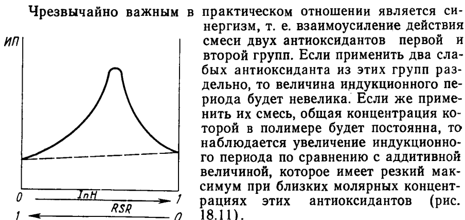
Рис. 18.11. Проявление синергизма защитного действия антиоксидантов аминного ( I_nH ) и сульфидного ( RSR ) типов при их совместном применении (индукционный период — концентрации ингибиторов)
