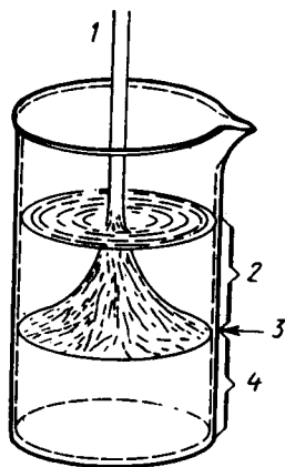
Рис. 5.1. Межфазная поликонденсация с образованием полиамидной пленки на границе раздела фаз растворов мономеров [10]:
