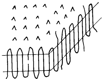
Рис. 12.2. Образование ламели из сложенных цепей
