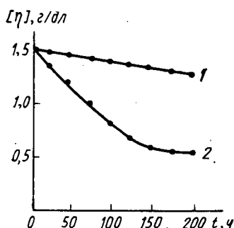
Рис. 16.1. Влияние облучения пленок ацетилцеллюлозы ультрафиолетовым светом на характеристическую вязкость ее ацетоновых растворов в атмосфере азота (1) и воздуха (2)
