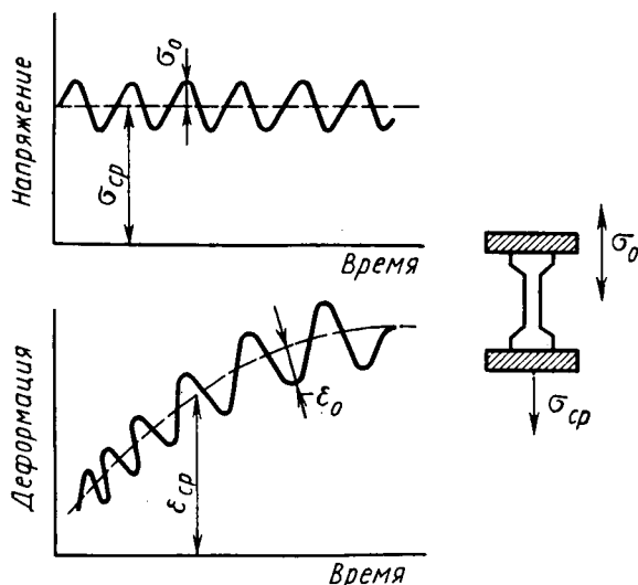
Рис. 13.13. Изменение амплитуды деформации \epsilon_0 и среднего значения деформации \epsilon_{cp} в условиях многократных деформаций при заданном постоянном \sigma_0 и \sigma_{cp} . Показана схема прибора для испытаний при \sigma_0 = \text{const} и \sigma_{cp} = \text{const}
