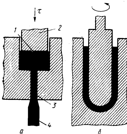
Рис. 11.4. Схема рабочего узла капиллярного (а) и ротационного (б) вискозиметров:
