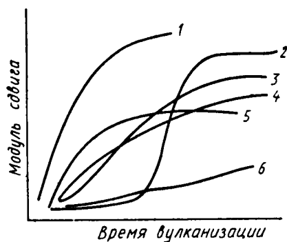
Рис. 20.4. Типичные кинетические кривые вулканизации эластомеров в присутствии различных ускорителей серной вулканизации:
