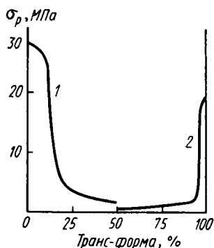
Рис. 19.3. Влияние изомеризации цис -1,4-полиизопрена (1) и транс -1,4-полиизопрена (2) на их прочность
