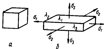
Рис. 8.2. Схематическое изображение трехмерной деформации: а — образец до деформации; б — после деформации
