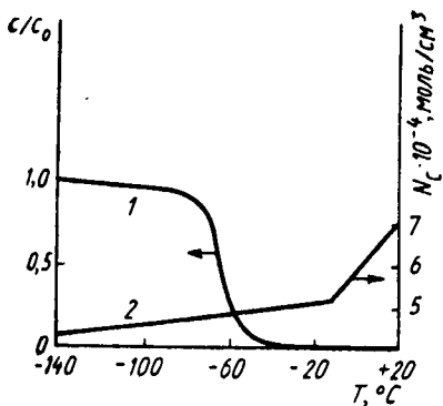
Рис. 16.3. Изменение относительной концентрации c/c_0 свободных радикалов (1) и числа поперечных связей N_c \cdot 10^{-4} моль/см 3 (2) при размораживании облученного в стеклообразном состоянии полиизопрена
