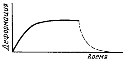
Рис. 9. 7. Кривая ползучести для модели Кельвина — Фойхта в соответствии с уравнением (9.12) (ср. с кривой 2 на рис. 9.4)
