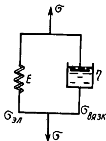
Рис. 9.6. Модель Кельвина — Фойхта
