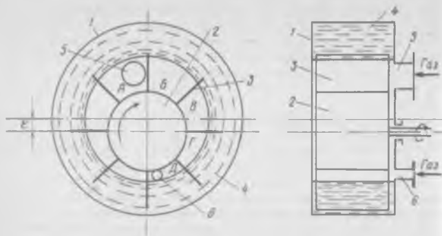
Рис. 9-9. Роторный водокольцевой (мокрый) компрессор:
