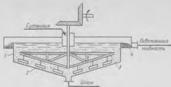
Рис. 10-1. Отстойник непрерывного действия с гребковой мешалкой:
