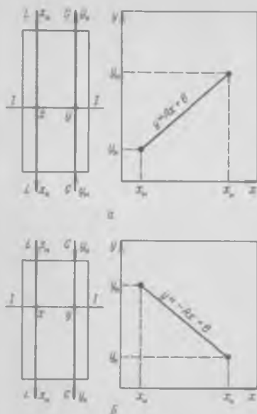
Рис. 1-2. К выводу уравнений материального баланса и рабочей линии газа (на примере абсорбции): а – противоток; б – прямоток
