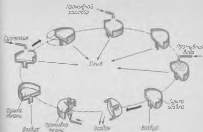
Рис. 10-21. Схема работы карусельного вакуум-фильтра
