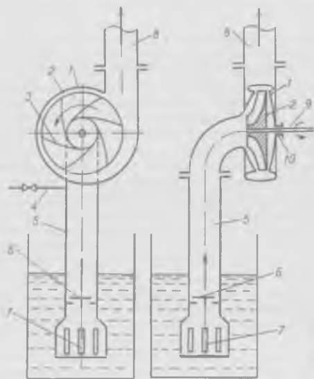
Рис. 8-15. Центробежный насос:
