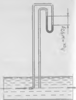
Рис. 6-14. Измерение локальной скорости жидкости пневмометрической трубкой
