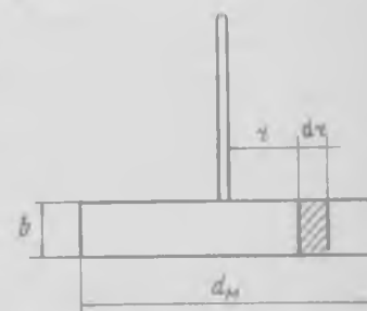
Рис. 7-4. К расчету мощности, затрачиваемой на перемешивание
