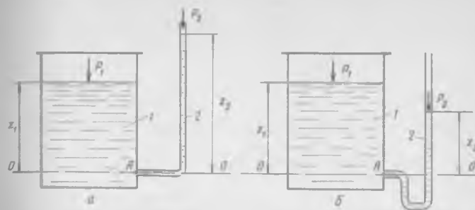
Рис. 6-3. К определению давления с помощью пьезометра: 1 — емкость; 2 — пьезометрическая трубка
