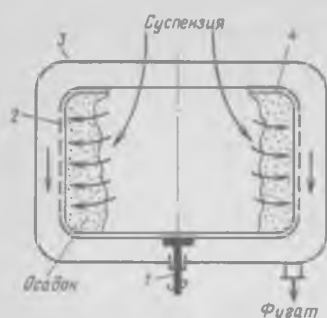
Рис. 10-22. Фильтрующая центрифуга периодического действия: 1 - вертикальный вал; 2 - перфорированный барабан; 3 - кожух; 4 - фильтровальная ткань
