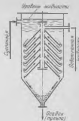
Рис. 10-2. Отстойник непрерывного действия с коническими полками
