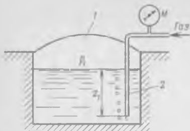
Рис. 6-4. К определению объема жидкости в хранилище: 1 - хранилище; 2 - измерительная трубка
