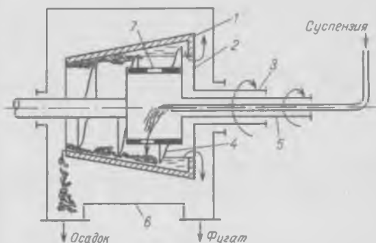
Рис. 10-8. Схема отстойной центрифуги непрерывного действия со шнековой выгрузкой осадка: 1 — конический барабан; 2 — внутренний барабан; 3 — полой внешний вал; 4 — лопасти шнека; 5 — полой внутренний вал; 6 — кожух; 7 — окна во внутреннем барабане
