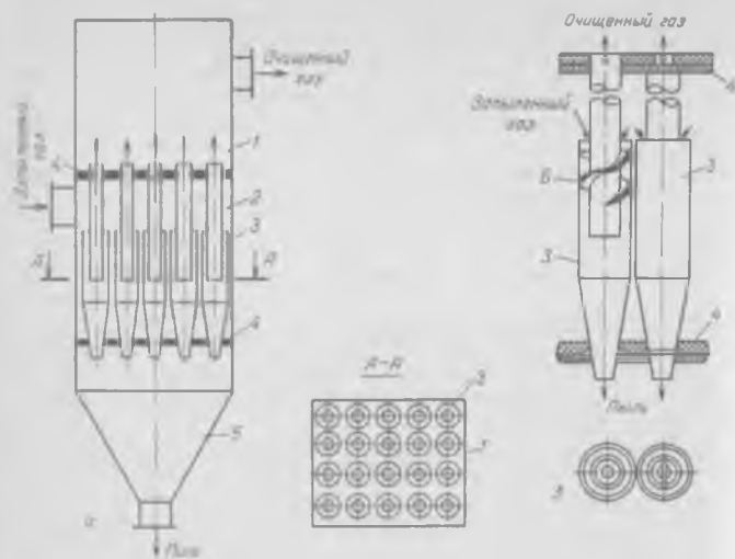
Рис. 10-6. Батарейный циклон (а) и его элементы (б):
