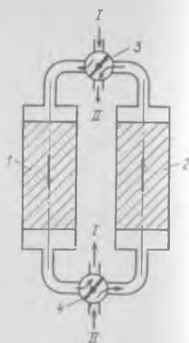
Рис. 13-19. Схема работы регенераторов с неподвижной насадкой: 1, 2 – регенеративные теплообменники с насадкой; 3, 4 – клапаны; I и II – холодный и горячий теплоносители
