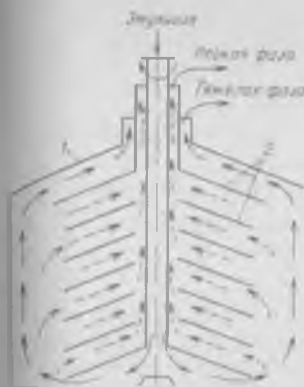
Рис. 10-9. Схема барабана сепаратора: 1 — корпус (ротор); 2 — тарелки
