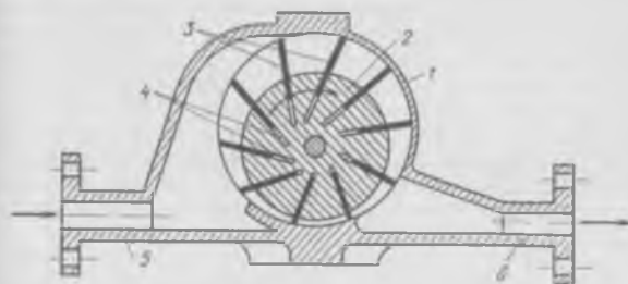
Рис. 9-8. Роторный компрессор пластинчатого (шиберного) типа:
