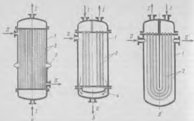
Рис. 13-6. Кожухотрубчатые теплообменники с компенсацией неодинаковости температурных удлинений труб и кожуха:
