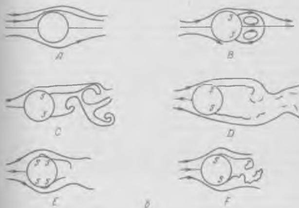
Рис. 6-15. Обтекание цилиндра поперечным потоком жидкости: а — зависимость коэффициента сопротивления \zeta от критерия Рейнольдса; б — характер обтекания цилиндра потоком жидкости. Остальные пояснения в тексте
