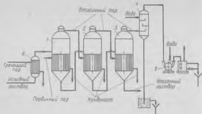
Рис. 14-2. Многокорпусная прямоточная выпарная установка: 1-3- корпуса; 4- барометрический конденсатор; 5- вакуум-насос; 6- подогреватель исходного раствора
