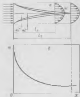
Рис. 11-12. Формирование полей скоростей и температур t(a) и изменение коэффициента теплоотдачи \alpha(b) на начальном участке труб при ламинарном движении теплоносителя
