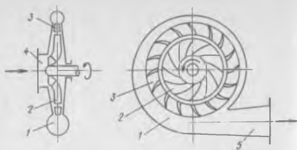
Рис. 9-12. Турбогазодувка:
