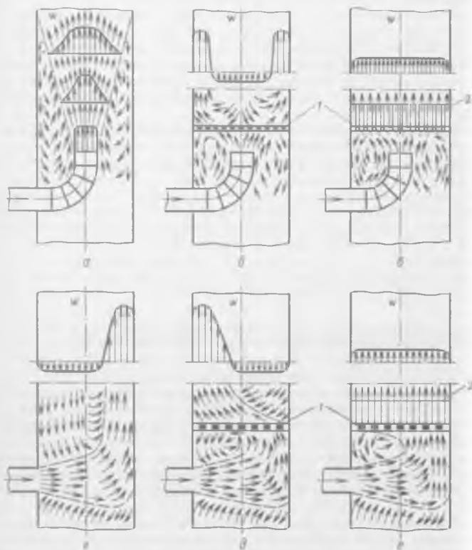
Рис. 5-1. Схемы распределения потока газа на входе в аппарат с центральным (а, б, г) и боковым (з, д, е) вводом потока и скоростей газа по сечению аппарата:
