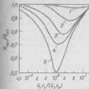
Рис. 11-21. Сравнение прямого ( Q_{\text{пр}} ) и противотока ( Q_{\text{пр}} ). 1 - KF/(G_1 c_1) = 0,1 ; 2 - 0,5; 3 - 1,0; 4 - 2,0; 5 - \infty
