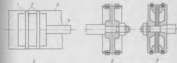
Рис. 8-3. Устройство поршня (а) и конструкции облегченных дисковых поршней — сплошного (б) и составного (в): 1 — поршень; 2 — сменные уплотняющие кольца; 3 — цилиндр; 4 — шток
