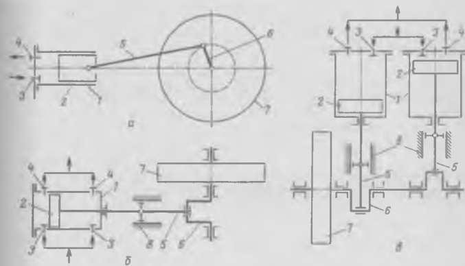
Рис. 9-4. Поршневые компрессоры простого действия:
