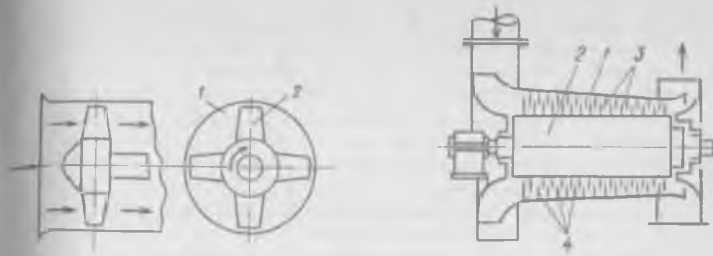
Рис. 9-13. Осевой (пропеллерный) вентилятор:
