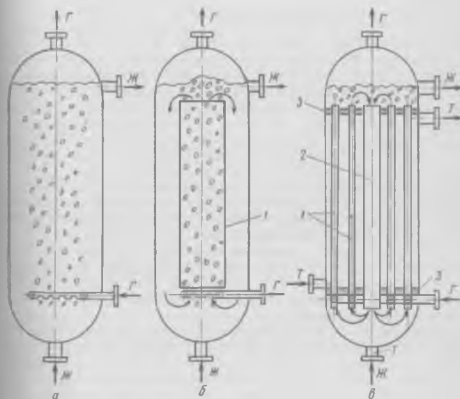
Рис. 7-9. Принципиальные схемы перемешивания с помощью сжатого газа: а — с центральным барботером; б — с газлифтной (эрлифтной) трубой; в — кожухотрубчатый аппарат с газлифтными трубами и циркуляционной трубой; 1 — газлифтные трубы; 2 — циркуляционная труба; 3 — трубные решетки; Ж — жидкость; Г — газ; Т — теплоноситель
