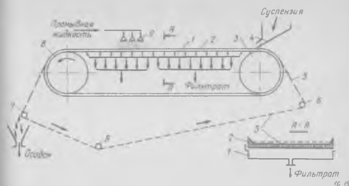
Рис. 10-19. Ленточный вакуум-фильтр:
