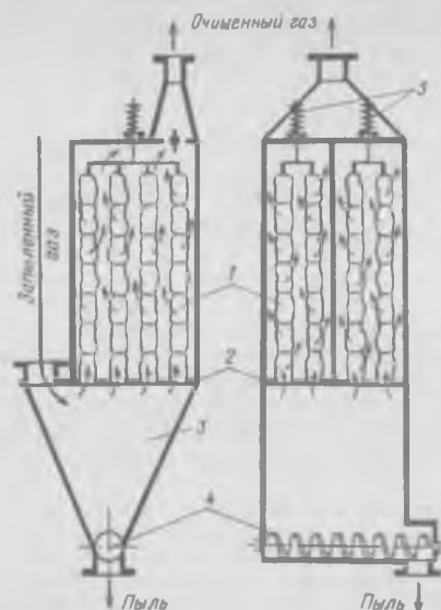
Рис. 10-24. Рукавный фильтр:
