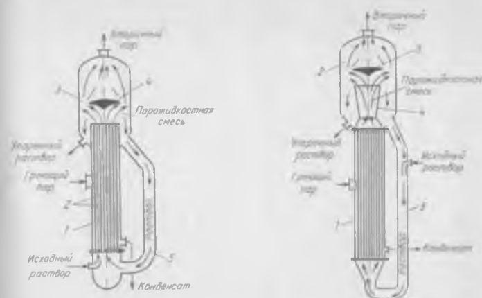
Рис. 14-7. Выпарной аппарат с вынесенной циркуляционной трубой:
