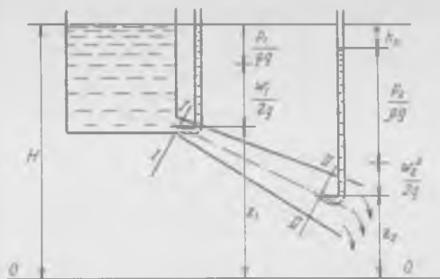
Рис. 6-6. К объяснению физического смысла уравнения Бернулли
