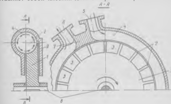
Рис. 8-23. Вихревой насос:
