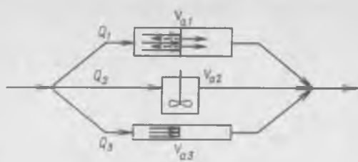
Рис. 5-9. Схема комбинированной модели структуры потоков:
