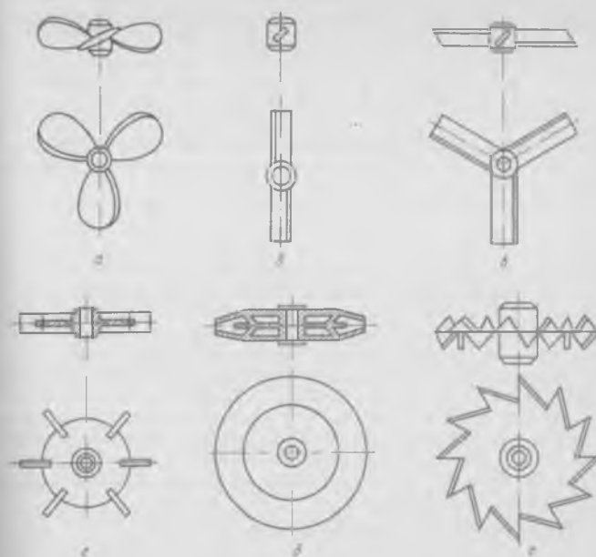
Рис. 7-8. Быстроходные мешалки:
