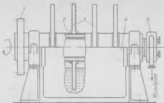
Рис. 10-20. Дисковый вакуум-фильтр:
