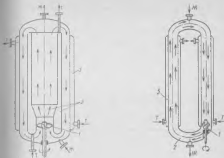
Рис. 7-10. Аппарат с винтовой мешалкой и диффузором:
