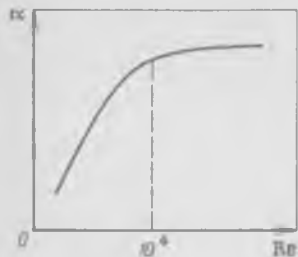
Рис. 6-10. Зависимость коэффициента расхода от критерия Рейнольдса
