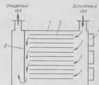
Рис. 10-4. Пылесадительная камера:
