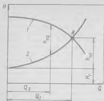
Рис. 8-21. Совместная характеристика центробежного насоса (1) и сети (2)
