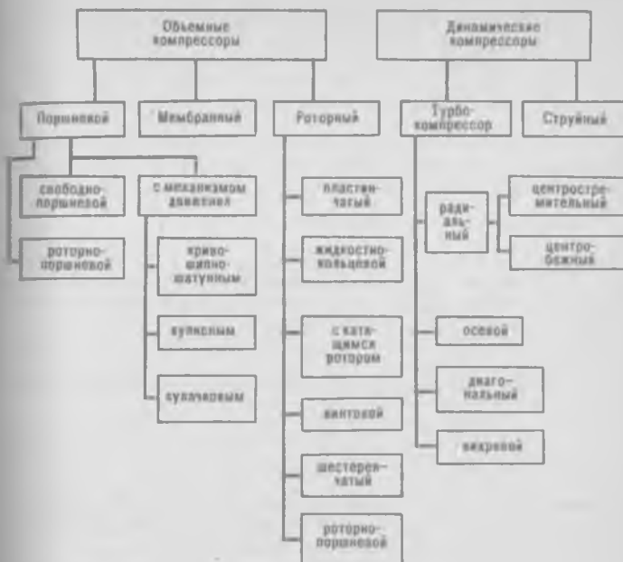
Рис. 9-1. Классификация основных типов компрессоров
