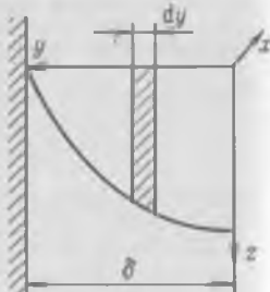
Рис. 6-18. Распределение скоростей по толщине стекающей пленки жидкости
