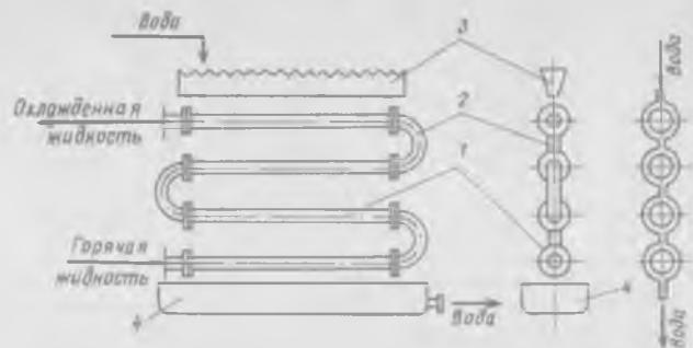
Рис. 13-10. Оросительный холодильник:
