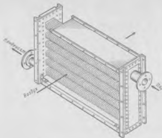
Рис. 13-13. Пластиначатый калорифер для подогрева воздуха
