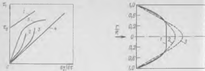
Рис. 6-27. Реологические характеристики жидкостей разных типов: 1 — бингамовской; 2 — неньютоновской (кажущаяся вязкость); 3 — дилатантной; 4 — ньютоновской; 5 — псевдопластичной
