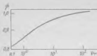
Рис. 11-7. Зависимость коэффициента \psi от критерия Прандтля
