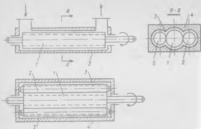
Рис. 8-12. Винтовой насос:
