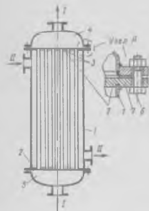
Рис. 13-1. Кожухотрубчатый теплообменник жесткой конструкции:
