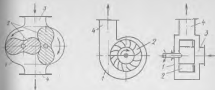
Рис. 9-10. Ротационный компрессор (газодувка) с двухлопастными роторами:
