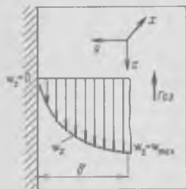
Рис. 6-18. Распределение скоростей по толщине стекающей пленки жидкости
