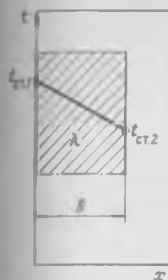
Рис. 11-1. К выводу уравнения теплопроводности плоской стенки
