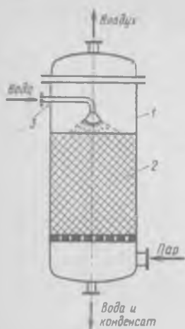
Рис. 13-18. Насадочный теплообменник-конденсатор: 1 – корпус; 2 – насадка; 3 – распределительное устройство
