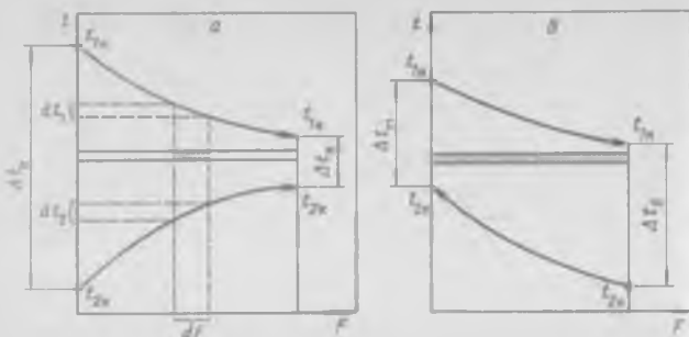
Рис. 11-17. К выводу уравнения теплопередачи при переменных температурах теплоносителей: а - при прямотоке; б - при противотоке
