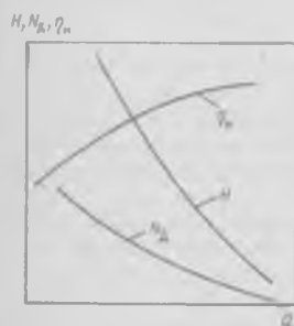
Рис. 8-24. Характеристика вихревого насоса
