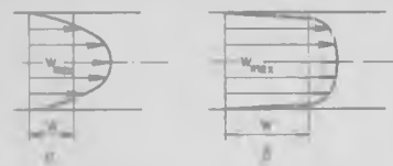
Рис. 3-4. Распределение скоростей по сечению потока при ламинарном (а) и турбулентном (б) режиме движения
