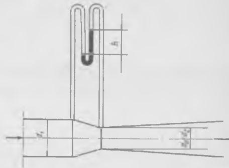
Рис. 6-13. Труба Вентури
