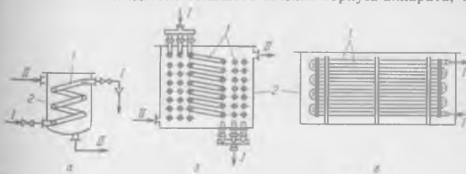
Рис. 13-8. Аппараты с погружными теплообменниками:
