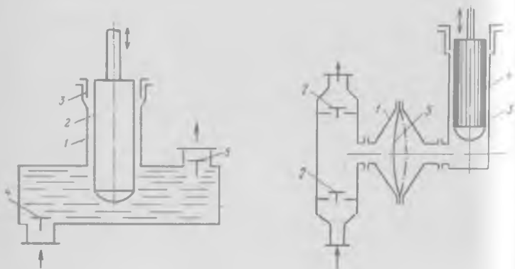
Рис. 8-5. Плунжерный вертикальный насос простого действия:
