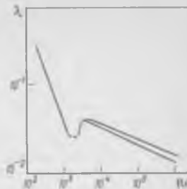
Рис. 6-7. Зависимость коэффициента трения \lambda от критерия Рейнольдса
