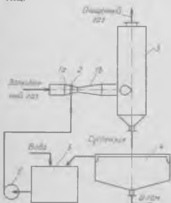
Рис. 10-27. Схема очистки газа с применением скруббера Вентури:
