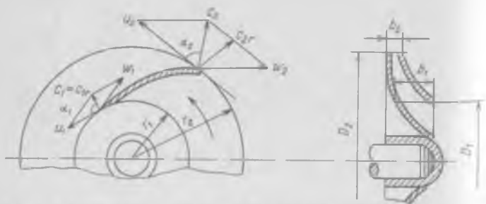
Рис. 8-17. К выводу основного уравнения центробежных машин
