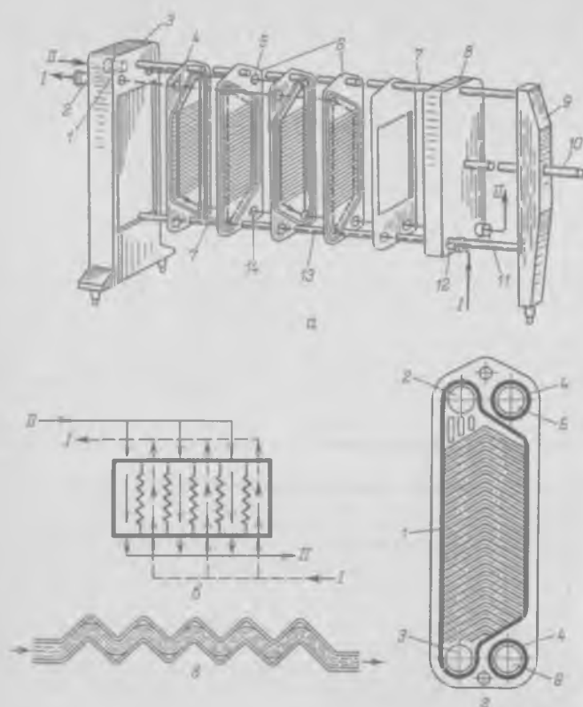
Рис. 13-14. Пластиначатый теплообменник «фильтр-прессного» типа и его элементы:
