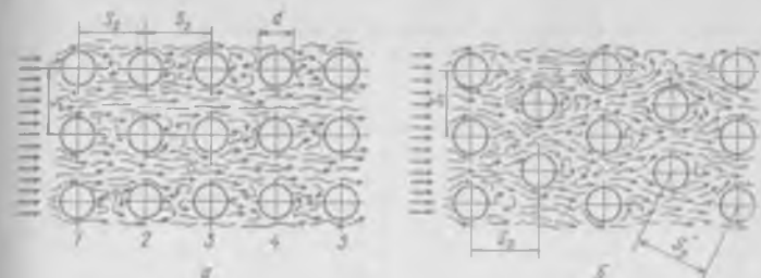
Рис. 11-14. Схема обтекания пучков труб: a – коридорных; b – шахматных; 1–5 – ряды труб
