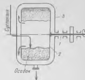
Рис. 10-7. Схема отстойной центрифуги периодического действия с горизонтальным валом и ручной выгрузкой осадка: 1 — вращающийся вал; 2 — барабан; 3 — кожух
