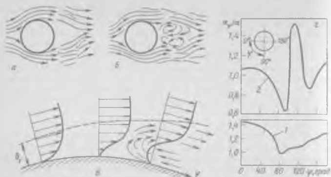
Рис. 11-13. Схема поперечного обтекания трубы теплоносителем:
