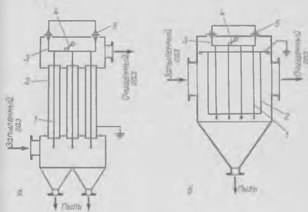
Рис. 10-12. Трубчатый (а) и пластинчатый (б) электрофильтры:
