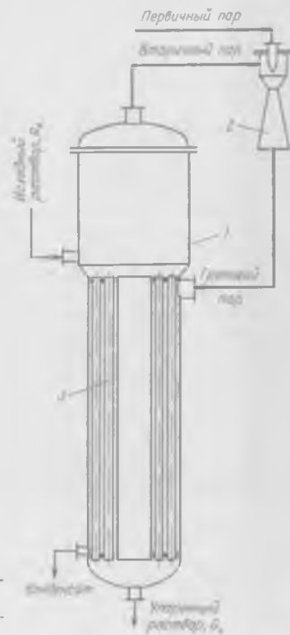
Рис. 14-6. Схема выпарного аппарата с тепловым насосом:
