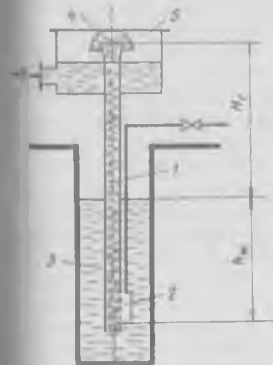
Рис. 8-26. Воздушный подъемник (эрлифт):
