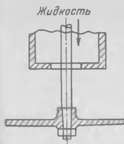
Рис. 6-22. Схема тарельчатого рабочего элемента
