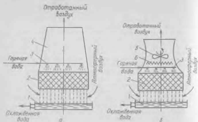
Рис. 12-10. Градири с естественной (а) и принудительной (б) тягой: 1 – поддоны; 2 – слои насадки; 3 – распределители охлаждающей воды; 4 – полая часть градири для обеспечения естественной тяги; 5 – осевой вентилятор; 6 – брызгоотбойник
