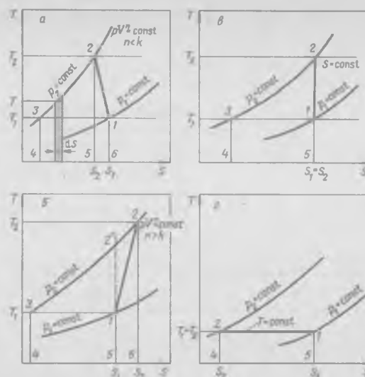
Рис. 9-2. Диаграммы S - T компрессорных процессов, описываемых уравнениями (9.3) — (9.5)
