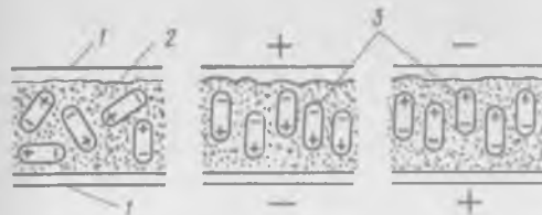
Рис. 12-9. Иллюстрация принципа высокочастотного (диэлектрического) нагрева: 1 — пластины конденсатора, к которым подведен ток высокой частоты; 2 — нагреваемый материал (диэлектрик); 3 — ориентированные (условно) частицы материала
