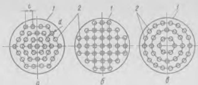
Рис. 13-2. Способы размещения труб в трубных решетках:
