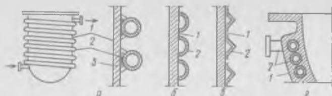
Рис. 13-9. Аппараты с наружными змеевиками:
