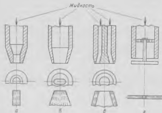
Рис. 6-21. Формы сопловых каналов и образующихся струй в струйных форсунках: а - цилиндрическое сопло; б - коническое сопло; в - игольчатое сопло; г - сопло в виде кругового прореза
