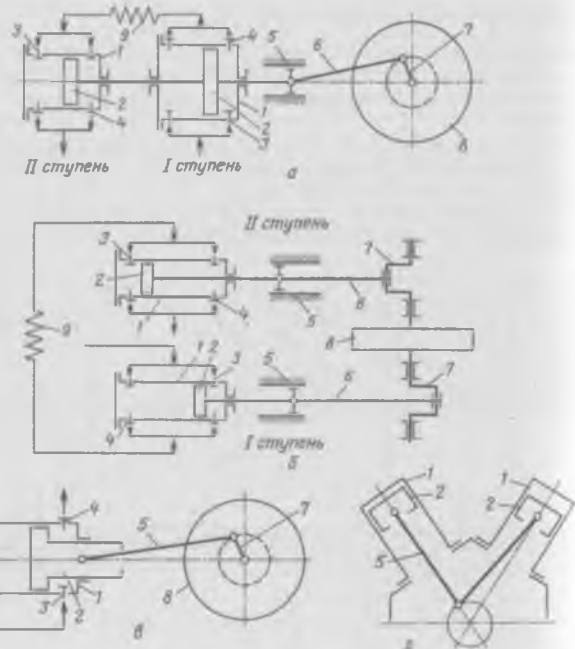
Рис. 9-5. Поршневые компрессоры двойного действия:
