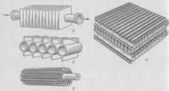
Рис. 13-12. Элементы теплообменников с оребрениями: а - поперечное оребрение; б - продольное «пластинчатое» оребрение; в - продольное оребрение; г - оребрение гофрированием плоских поверхностей теплообмена
