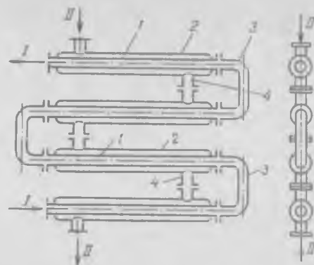
Рис. 13-7. Двухтрубный теплообменник типа «труба в трубе»:
