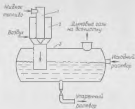
Рис. 14-11. Барботажный выпарной аппарат с погружной горелкой:
