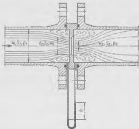
Рис. 6-11. Диафрагма для измерения расхода потока в трубопроводе
