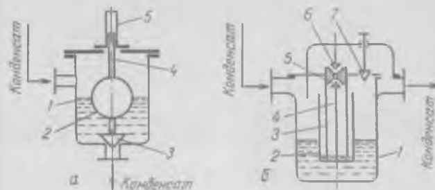
Рис. 12-3. Конденсатоотводчики:
