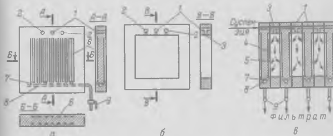
Рис. 10-17. Фильтр-пресс:
