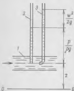
Рис. 6-5. К выводу уравнения Бернулли для горизонтального потока:
