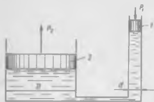
Рис. 6-2. Схема гидравлического пресса
