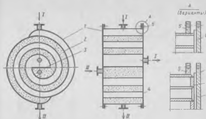
Рис. 13-15. Спиральный теплообменник:
