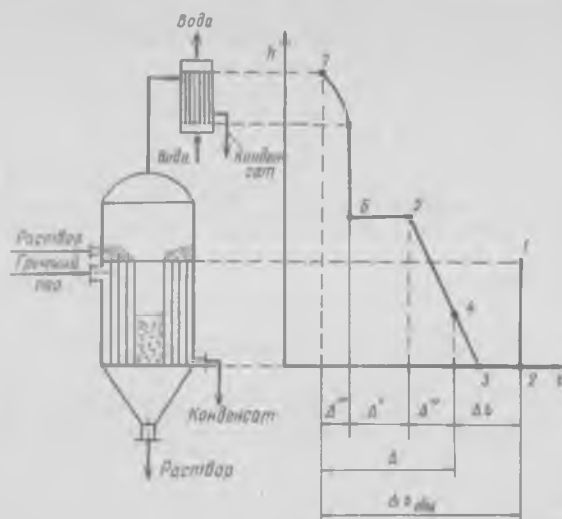
Рис. 14-3. Схема аппарата и температурный график выпарной установки: 1-2 конденсация греющего пара (без учета охлаждения конденсата); 3-5 изменение температуры кипения под действием гидростатического столба жидкости; 4 температура кипения раствора; 5-6 концентрационная температурная депрессия; 6-7 гидродинамическая температурная депрессия
