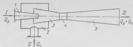
Рис. 8-25. Струйный насос:
