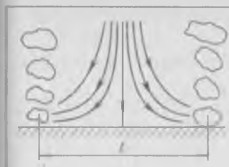
Рис. 11-10. Схема процесса теплоотдачи при пузырьчатом кипении
