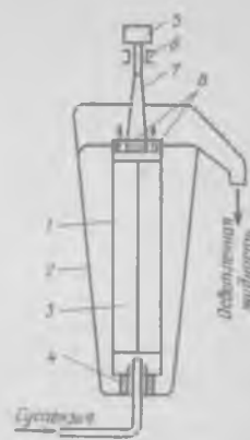
Рис. 10-10. Трубчатая сверхцентрифуга периодического действия для осветления жидкостей: 1 — трубчатый барабан (ротор); 2 — кожух; 3 — радиальные лопасти; 4 — подпятник; 5 — шкив; 6 — опора; 7 — шпиндель; 8 — отверстия для вывода осветленной жидкости
