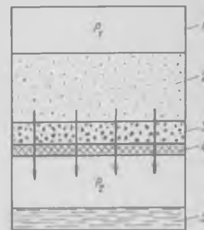
Рис. 10-13. Схема филтра для разделения суспензии
