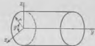
Рис. 3-9. К выводу уравнения Навье–Стокса для цилиндрических координат
