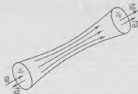
Рис. 3-7. К выводу уравнения (3.35)
