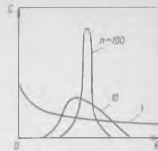
Рис. 5-7. Кривые отклика для ячеечной модели при импульсном вводе индикатора
