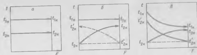
Рис. 11-20. К выбору взаимного направления движения теплоносителей (варианты а-в)
