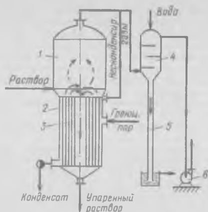
Рис. 14-1. Схема однокорпусной выпарной установки:
