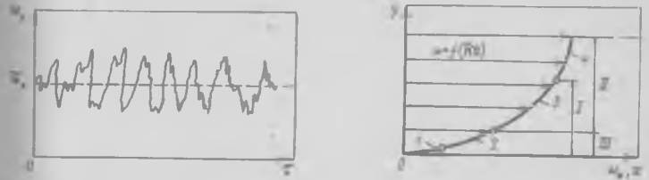
Рис. 3-5. Истинная w_x и осредненная \bar{w}_x локальные скорости жидкости в турбулентном потоке
