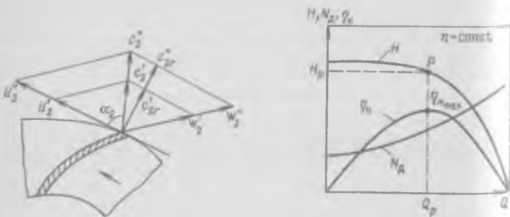
Рис. 8-18. Подобие параллелограммов скоростей при разных числах оборотов рабочего колеса
