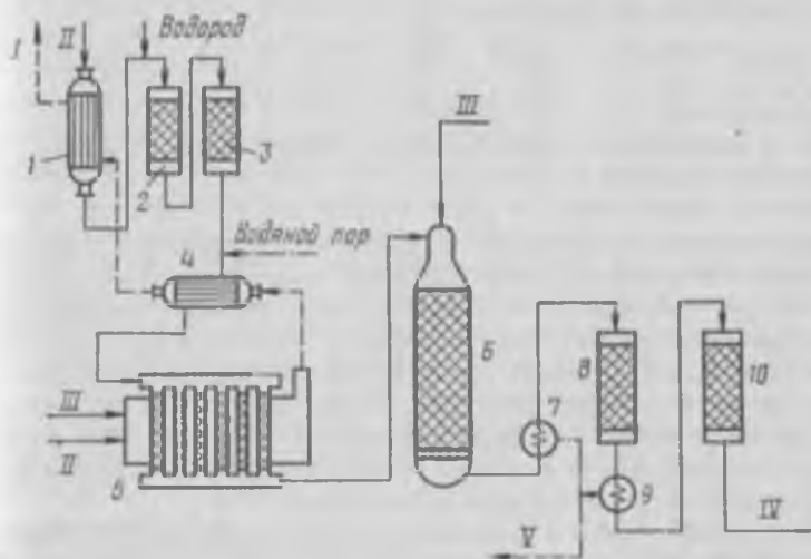
Рис. 9.20. Энерготехнологическая схема конверсии метана природного газа:
