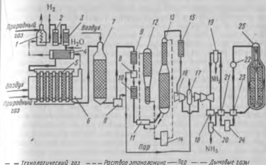
Рис. 10.6. Принципиальная схема синтеза аммиака под средним давлением:
