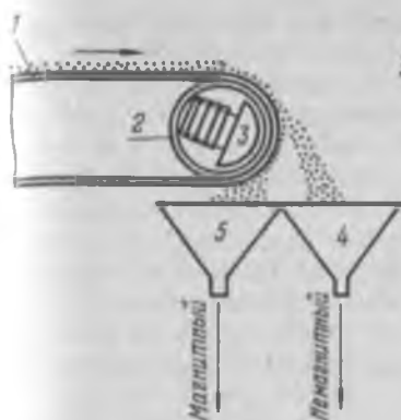
Рис. 7.3. Схема электромагнитного сепаратора:
