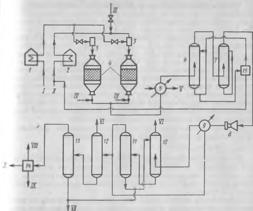
Рис. 14.6. Схема дегидрирования бутана в кипящем слое катализатора:
