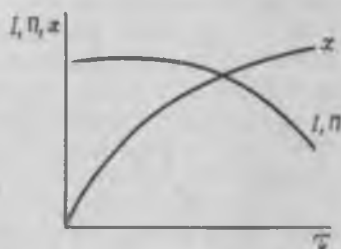
Рис. 3.1. Изменение производительности \Pi , интенсивности I и степени превращения x во времени для реактора идеального вытеснения
