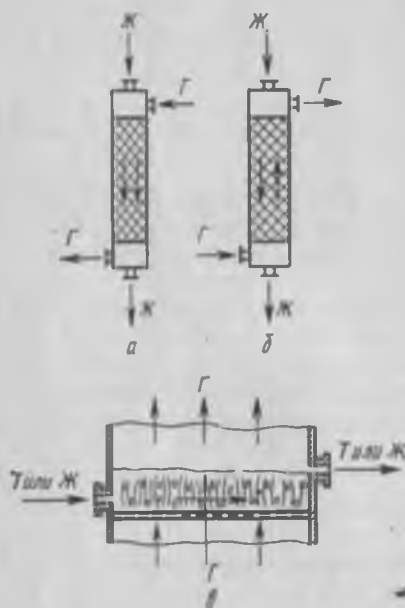
Рис. 2.6. Направление движения потоков в двухфазной системе Г—Ж:
