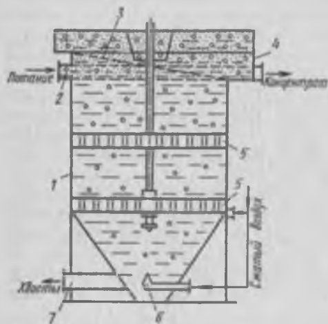
Рис. 7.6. Принципиальная схема пневматической флотомашины ФП-100:
