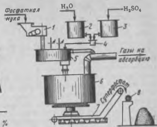
Рис. 12.2. Технологическая схема непрерывного способа производства суперфосфата:
