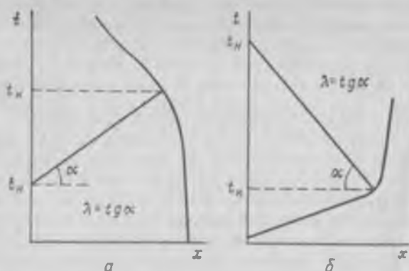
Рис. 3.16. Зависимость конечной температуры процесса t_N от степени превращения x для экзотермической (а) и эндотермической (б) реакций в адиабатическом реакторе идеального вытеснения
