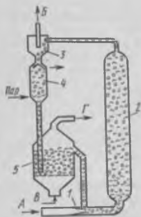
Рис. 5.15. Схема установки каталитического крекинга с восходящим потоком взвеси пылевидного катализатора:
