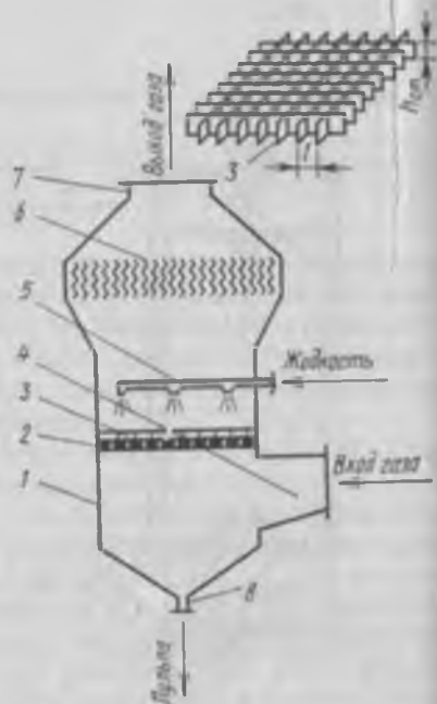
Рис. 4.11. Пенный аппарат:
