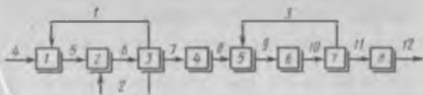
Рис. 6.11. Замкнутая схема
