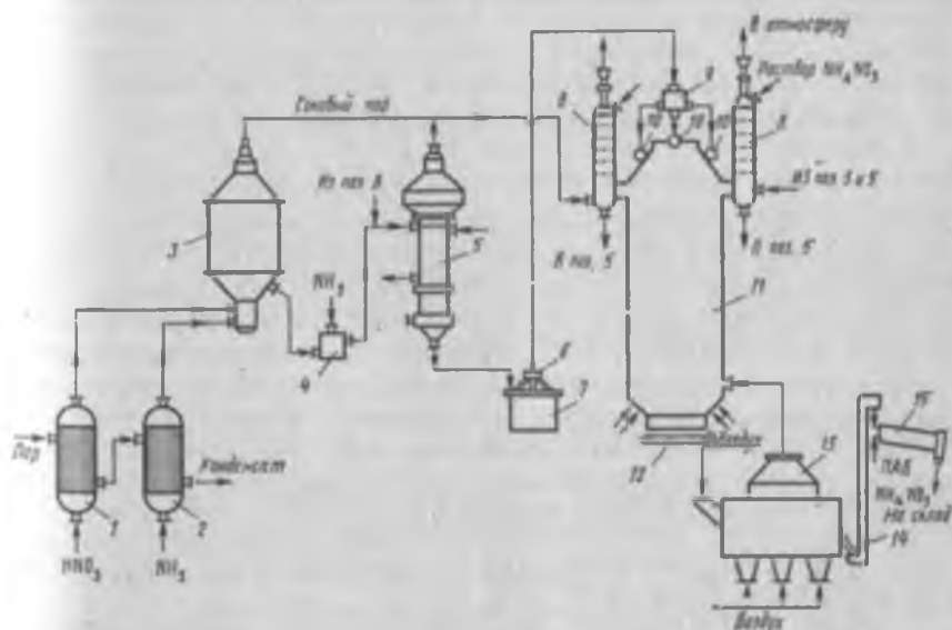
1 — подогреватель азотной кислоты; 2 — подогреватель аммиака; 3 — нейтрализатор ИТН; 4 — донеперизатор; 5 — выпарной аппарат; 6 — погружной насос; 7 — сборник плава сепаратор; 8 — промывная колонна; 9 — напорный сборник для плава; 10 — аэрогравитатор; 11 — грануляционная башня; 12 — транспортер; 13 — холодильник КС; 14 — адепатор; 15 — агрегатация барабан.
