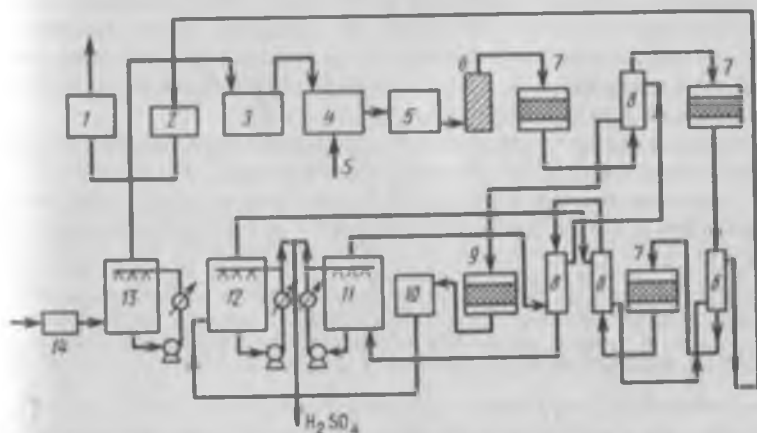
Рис. 6.17. Энерготехнологическая схема производства серной кислоты: 1, 10 — экономайзеры; 2 — газовая турбина; 3 — компрессор; 4 — установка для сжигания серы; 5 — котел-утилизатор; 6 — газовый фильтр; 7, 9 — контактные аппараты; 8 — тепло- обменник; 11, 12 — абсорберы; 13 — сушильная башня; 14 — воздушный фильтр
