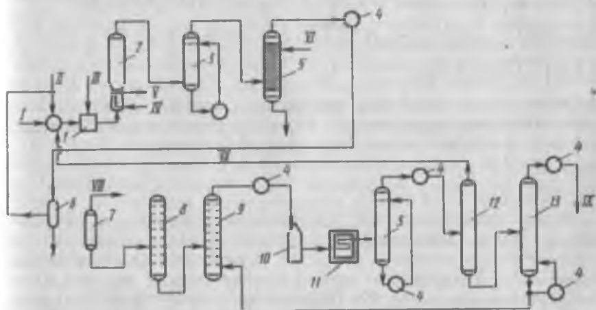
Рис. 14.11. Упрощенная схема синтеза винилхлорида из этилена:
