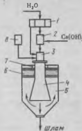
Рис. 7.9. Схема известково-содового способа умягчения воды:
