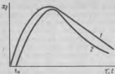
Рис. 9.12. Зависимость выхода бензина каталитического крекинга x_6 от времени пребывания сырья в реакторе (1) и температуры (2)
