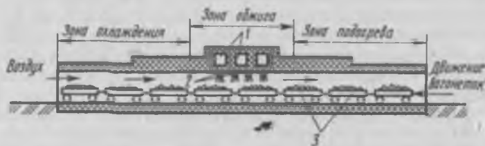
Рис. 4.17. Туннельная печь (продольный разрез):
