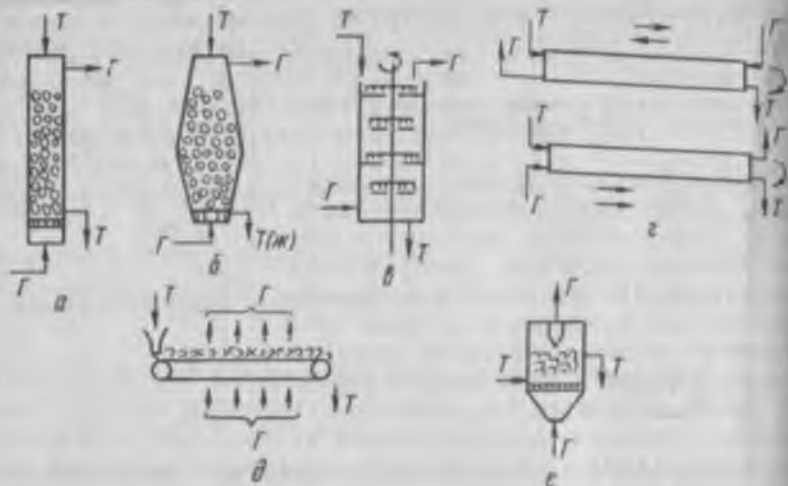
Рис. 4.14. Типы реакторов для процессов с участием газовых и твердых реагентов ( G-T ) для политермического ( a-d ) и изотермического ( e ) режимов:
