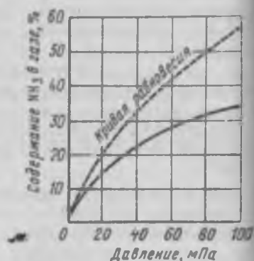
Рис. 10.3. Зависимость выхода аммиака от давления (объемная скорость 30 000 ч -1 ; t=500^\circ\text{C} ; катализатор железный)
