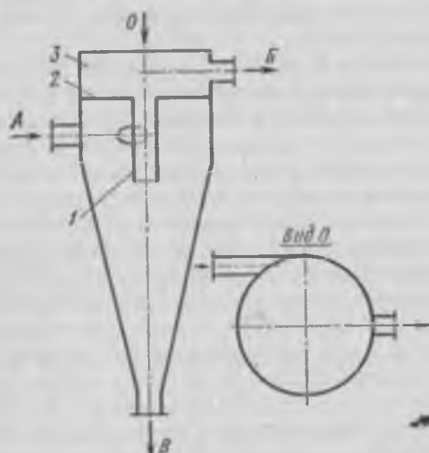
Рис. 7.2. Схема гидроциклона:
