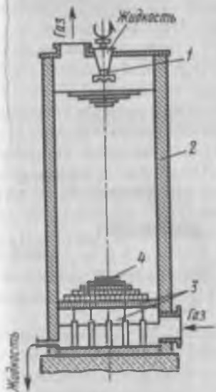
Рис. 4.8. Башня с насадкой:
