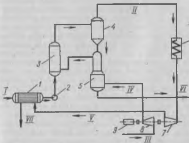
Рис. 8.8. Энерготехнологическая система мокрого сжигания сульфитных щелоков:
