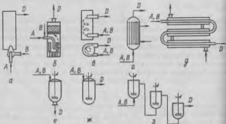
Рис. 4.3. Типы реакторов для гомогенных процессов газофазных (а—д) и жидкофазных (е—з):
