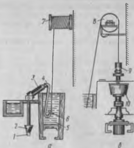
Рис. 15.11. Схема прядения:
