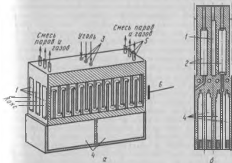
Рис. 9.15. Коксовая печь:
