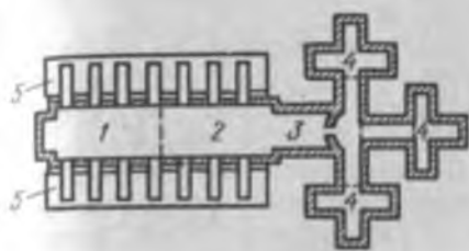
Рис. 4.18. Схема стекловаренной печи (вид сверху):
