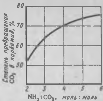
Рис. 12.7. Зависимость выхода карбамида от соотношения аммиака и диоксида углерода ( t=180\div 200^\circ\text{C} , P=180\div 200 МПа)
