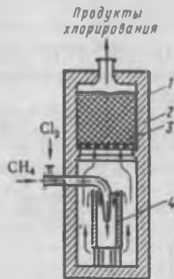
Рис. 14.9. Аппарат для хлорирования метана
