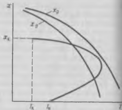
Рис. 5.12. Изменение степени превращения для экзотермической реакции в трубчатом контактном аппарате:
