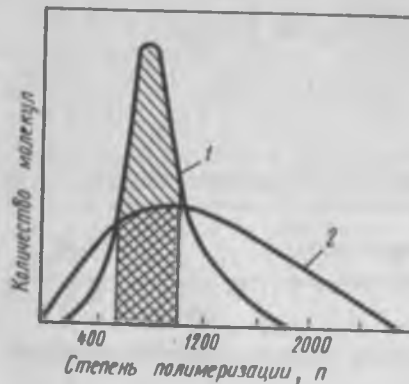
Рис. 15.1. Распределение молекул по степени полимеризации: 1 — пиктоцеллюлоза; 2 — полистирол
