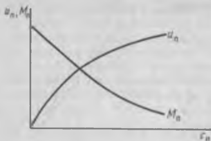
Рис. 15.5. Зависимость скорости полимеризации ( u_n ) и средней молярной массы ( M_n ) от концентрации инициатора c_n
