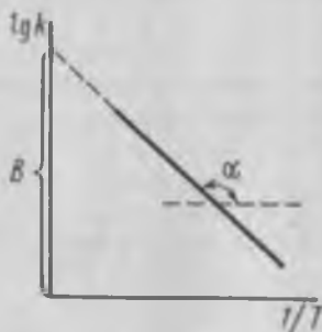
Рис. 2.11. Зависимость константы скорости реакции от температуры
