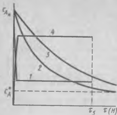
Рис. 2.4. Изменение концентраций по времени процесса для простой обратимой реакции:
