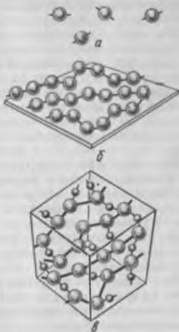
Рис. 15.3. Связь между мономерами в молекуле полимера:
