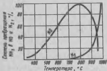
Рис. 10.8. Зависимость степени превращения аммиака от температуры ( \tau = \text{const} , катализатор Pt—Pd—Rh)
