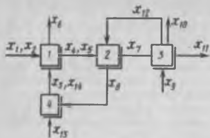
Рис. 6.13. Схема замкнутой ХТС
