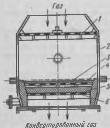
Рис. 10.10. Контактный аппарат:
