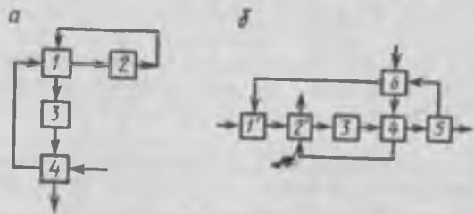
Рис. 6.5. Замкнутая ХТС:
