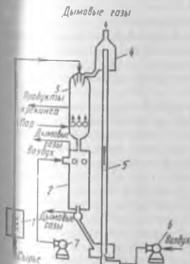
Рис. 9.13. Схема каталитического крекинга в плотном слое движущегося катализатора: 1 — труба подачи сырья; 2 — реактор; 3 — регенератор; 4 — бункер; 5 — котел-утилизатор; 6 — труба подачи воздуха; 7 — воздуходувка
