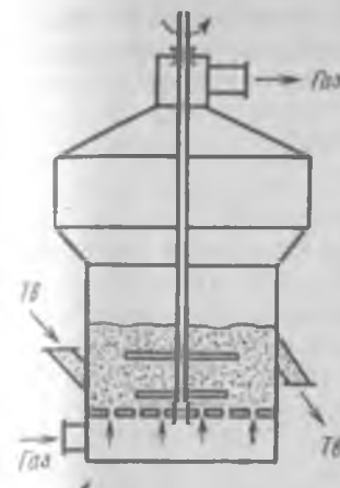
Рис. 3.13. Реактор полного смешения — аппарат КС с мешалкой
