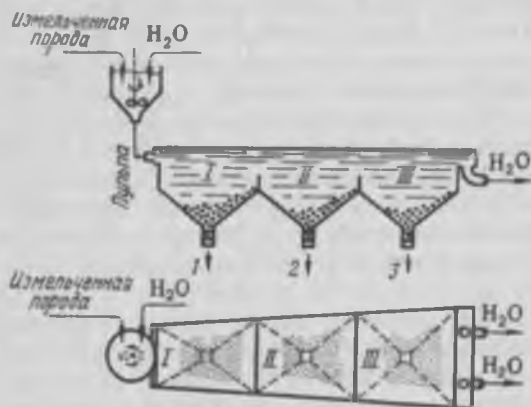
Рис. 7.1. Принципиальная схема мокрого гравитационного обогащения:
