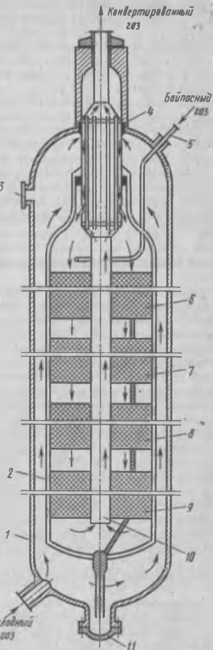
рис. 10.7. Схема четырехполочной колонны синтеза аммиака под средним давлением:
