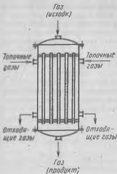
Рис. 3.7. Реактор идеального вытеснения — контактный аппарат для эндотермических реакций с катализатором в трубках
