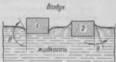
Рис. 7.4. Влияние смачивания
