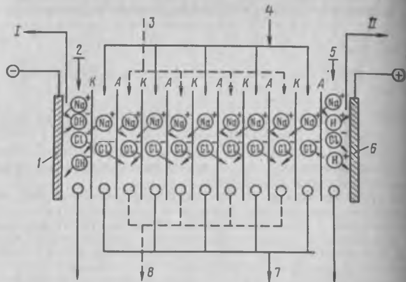
Рис. 8.3. Схема процесса электролиза:
