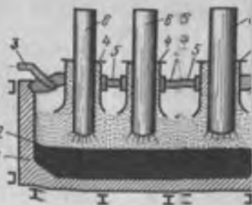
Рис. 4.19. Дуговая печь прямого ва для производства карбида кальция
