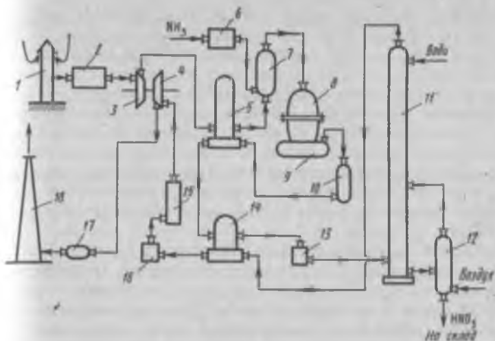
Рис. 10.11. Принципиальная технологическая схема получения разбавленной азотной кислоты под повышенным давлением (0,73 МПа):
