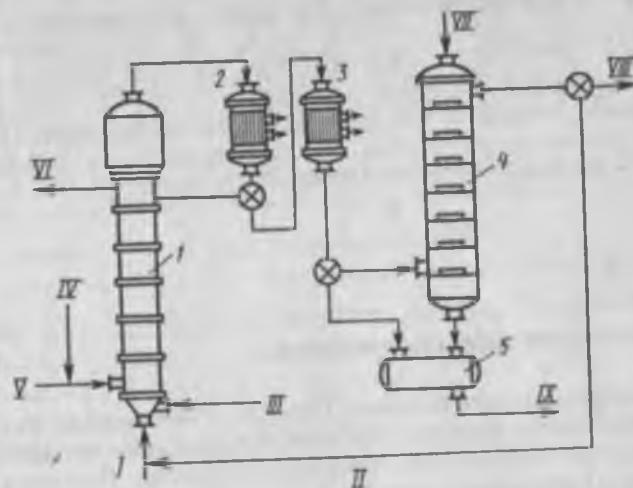
Рис. 14.15. Схема получения ацетальдегида гидратацией ацетилена в жидкой фазе:
