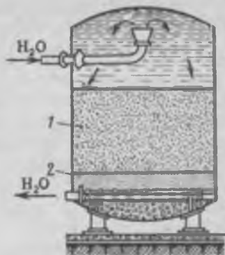
Рис. 7.11. Катионитовый фильтр: 1 — катионит; 2 — песок
