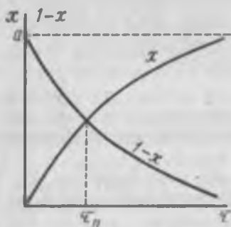
Рис. 4.1. Зависимость выхода продукта и количества оставшегося вещества (1-x) от времени для необратимой реакции первого порядка
