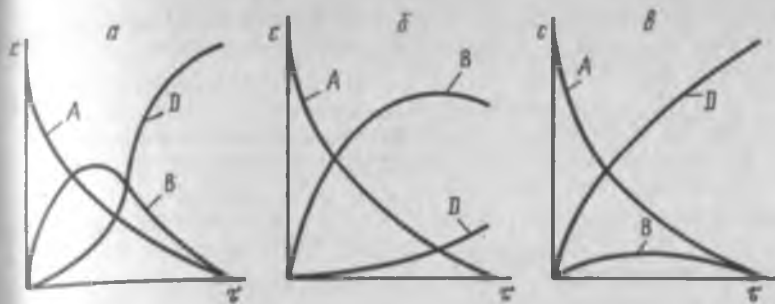
Рис. 2.3. Изменение концентрации в последовательных необратимых реакциях
