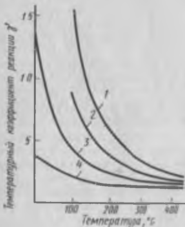
Рис. 2.10. Зависимость температурного коэффициента скорости реакции \gamma от температуры t и энергии активации E :
