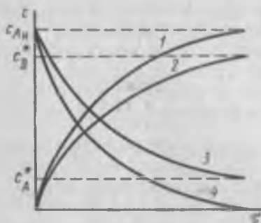
Рис. 2.1. Типичные кривые изменения концентраций реагентов во времени для простых реакций типа A \rightarrow D в реакторах вытеснения:
