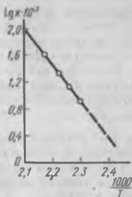
Рис. 15.4. Зависимость константы скорости поликонденсации гексаметилендиамина с себаценовой кислотой ( E=100 кДж/моль) от температуры
