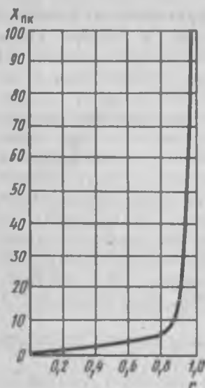
Рис. 15.6. Зависимость степени полимеризации ( \bar{X}_{пк} ) от коэффициента эквивалентности ( r )
