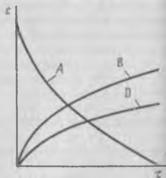
Рис. 2.2. Изменение концентраций в бинарнопараллельной необратимой реакции
