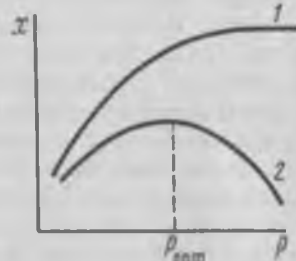
Рис. 2.9. Зависимость выхода продукта от давления для обратимой газовой реакции ( \tau, t, c_A, c_B = \text{const} ): 1 — \Delta n < 0 ; 2 — \Delta n > 0
